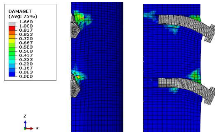
Figura 13 - Dano à tração no núcleo de concreto
