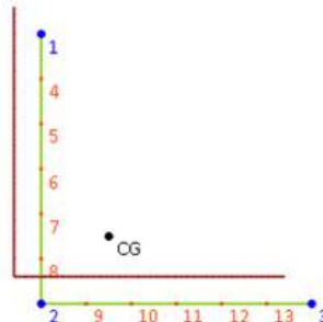
Figura 20 — Resultados para análise numérica via GBTUL para cantoneira L60x60x2.38x1330 — Determinação da carga crítica de flambagem elástica e respectivo modo de falha. Torção 92,21% e Flexão 7,78%.
