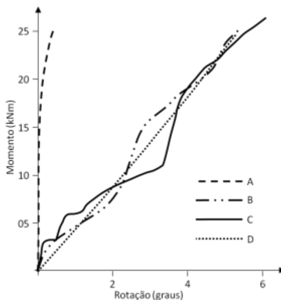
Figura 4 – Resultados de Prabha, Rekha, Marimuthu, Saravanan, Pa lani e Surendran[7] para LCPP de espessura 6 mm, altura 205 mm, com 10 mm entre a viga e a coluna: (A) Modelo de Frye-Morris (1975); (B) Resultado experimental; (C) Resultado do software Abaqus; (D) Modelo proposto por Prabha et al.
