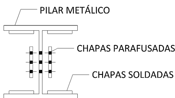
Figura 7: União de perfis metálicos utilizados como pilar (seção transversal)
