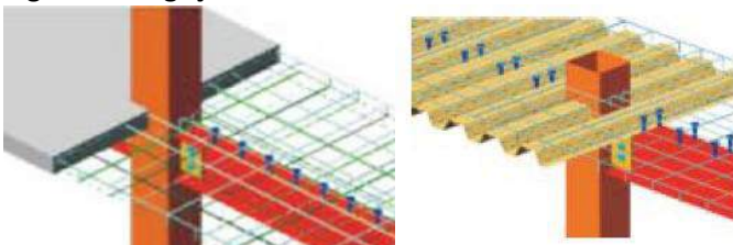
Figura 12 -Ligações mistas
