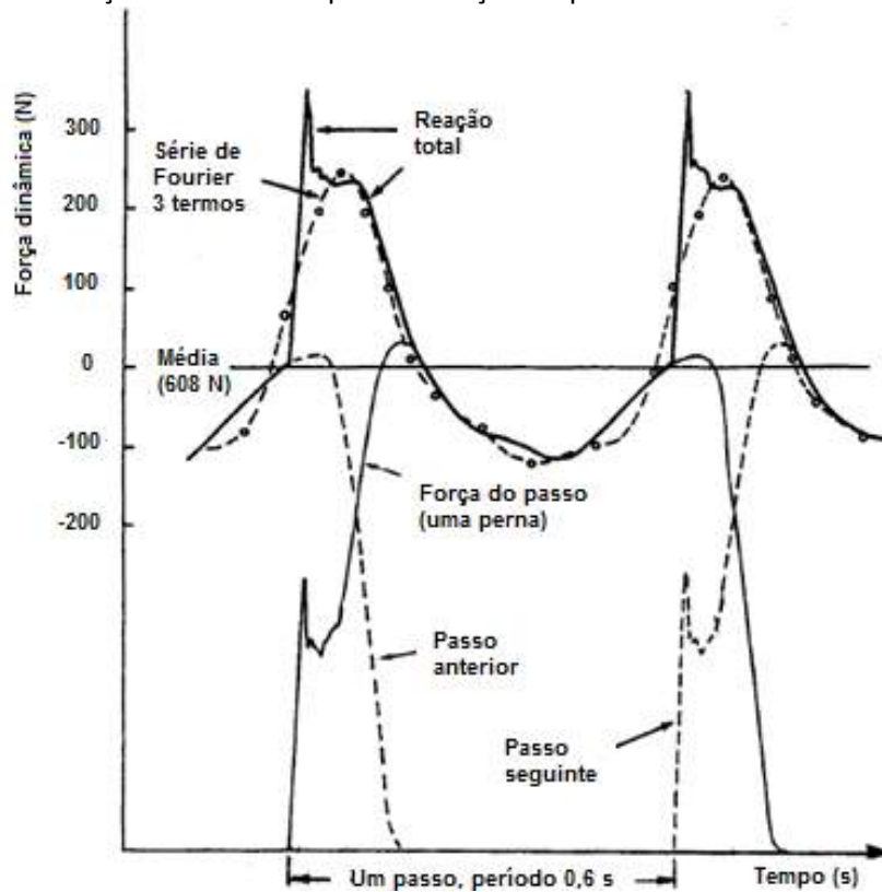
Figura 5 - Componentes harmônicas da série de Fourier para caminhada [10].
