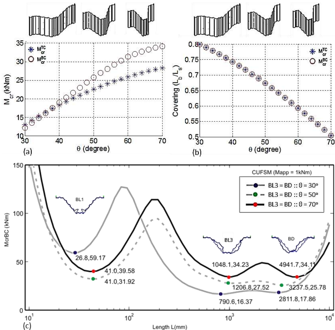
Figura 17: Tendências resultantes da variação do ângulo \theta entre almas e mesas para enrijecedores trapezoidais com w_{incl}=17 mm, w_{mid}=15 mm, ang_3 = 46^\circ : (a) momentos críticos associados à compressão da mesa superior e inferior, (b) taxa de cobrimento e (c) curvas de "assinatura" para compressão da mesa inferior M_{cr}^{BC} e ângulo entre mesas e almas \theta = 30^\circ, 50^\circ e 70^\circ .
