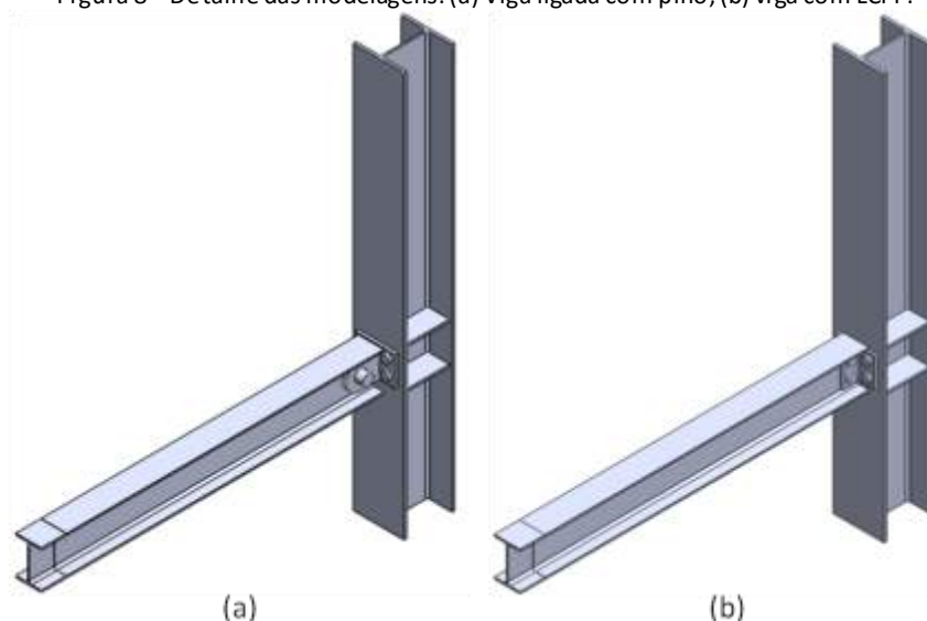
Figura 8 – Detalhe das modelagens: (a) Viga ligada com pino; (b) viga com LCPP.
