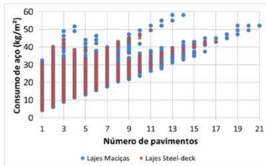
Figura 33 - Relação entre número de pavimentos da torre e o consumo para aço MR250. (Fonte: elaborada pelos autores)
