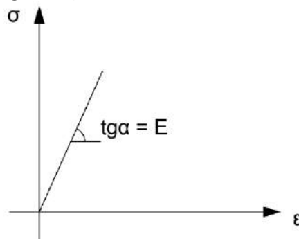
Figura 21 – Modelo constitutivo usado na análise linear.
