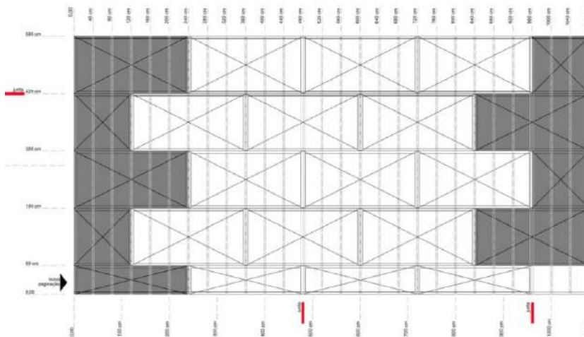
Figura 6 - Paginação de placas com juntas de dilatação. Fonte: BRICKA [13]
