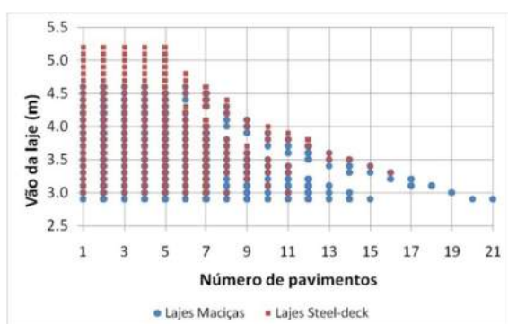
Figura 25 - Relação entre vão da laje e número de pavimentos de pilares em perfis em aço MR250. (Fonte: elaborada pelos autores)
