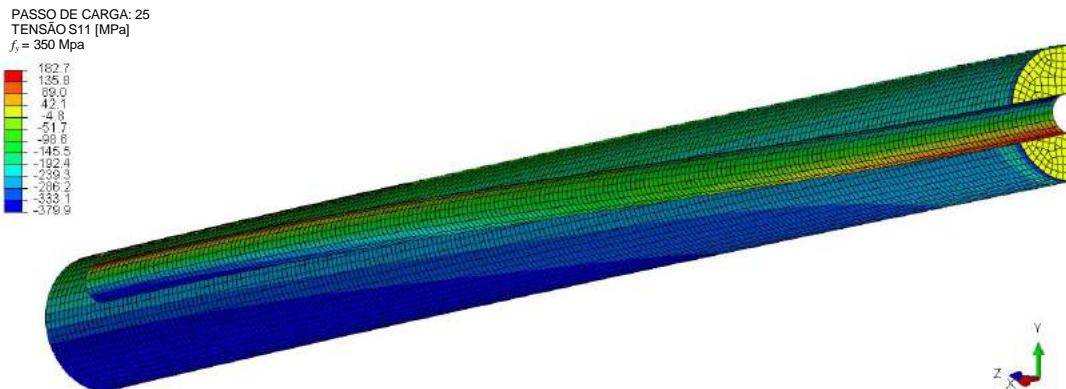
Figura 15 – Modelo 17 sem travamentos – Tensões atuantes – Passo de carga 25 ( \lambda_0 = 1,07 e \lambda = 80 )
