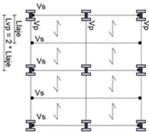
Figura 1 – Sistema de piso 2M. (Fonte: adaptado de Brito e Silva [8]).
