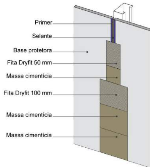
Figura 2: Tratamento de juntas da Drylevis Fonte: Criado pelos autores
