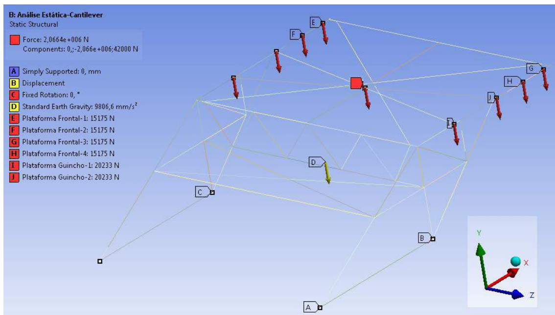
Figura 7 – Condições de contorno aplicadas ao modelo de elementos finitos da treliça içadora de aduelas.
