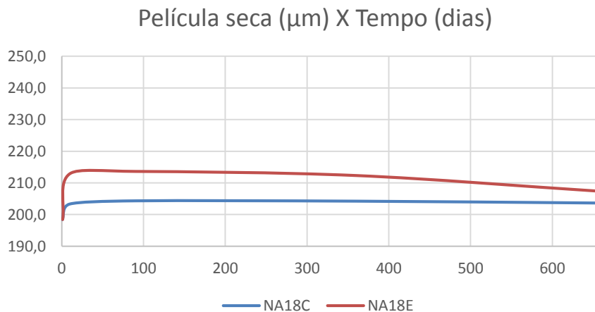
Figura 32: Comparativo gráfico entre corpos NA18 (C) não exposto e (E) exposto
