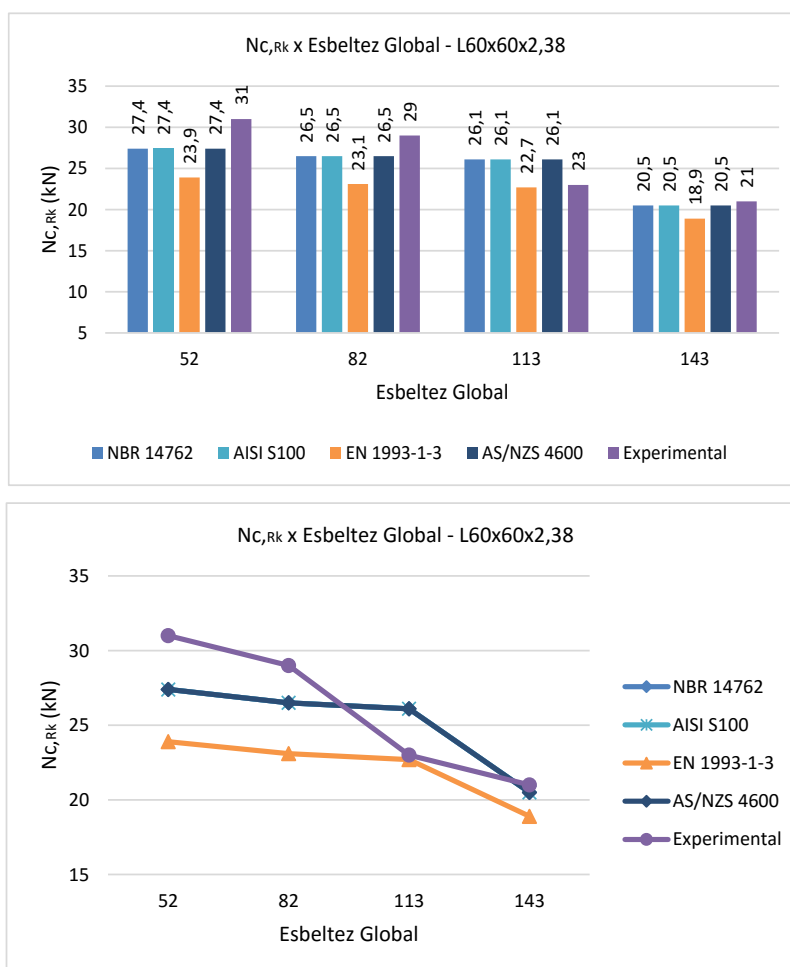
Figura 12 — Resultados analíticos para cantoneira simples - MLE
