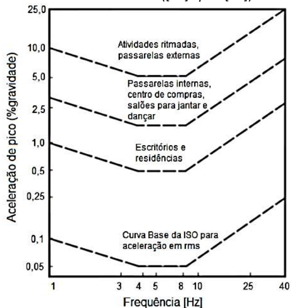
Figura 12 - Aceleração de pico recomendada para conforto humano para vibrações devido a atividades humanas ([23] apud [24]).
