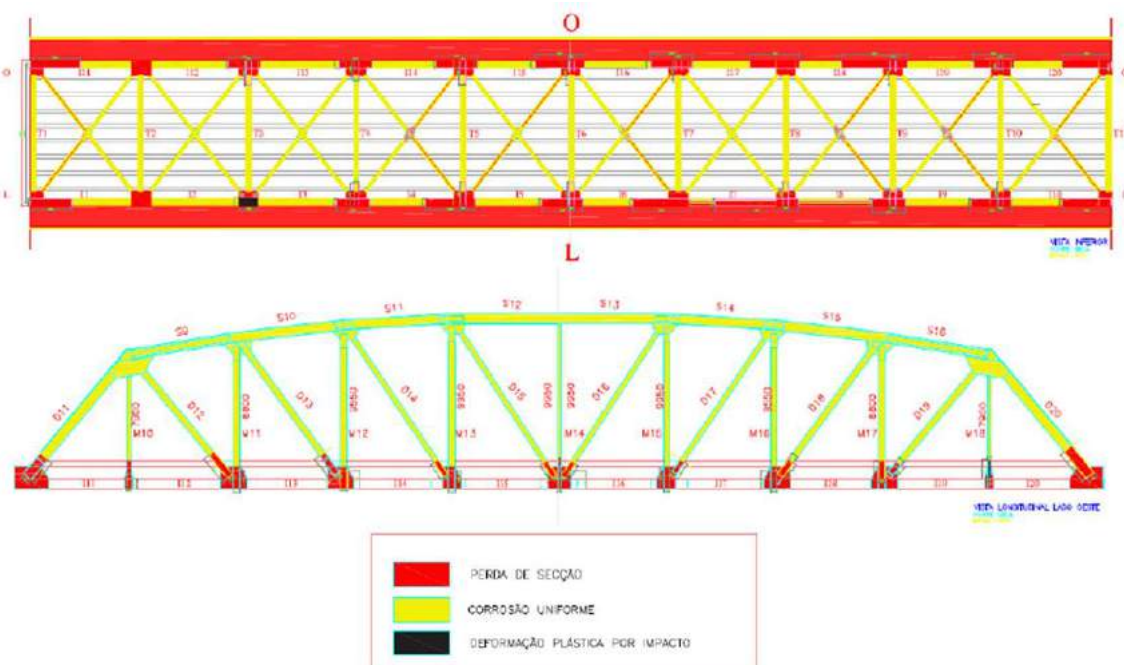
Figura 09 – Indicativos de reparos e recuperação da estrutura
