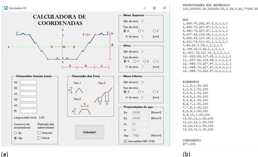
Figura 18: (a) Implementação de sistema generativo com interface gráfica amigável; (b) arquivo de texto com inputs para análise de flambagem elástica no programa computacional CUF5M.
