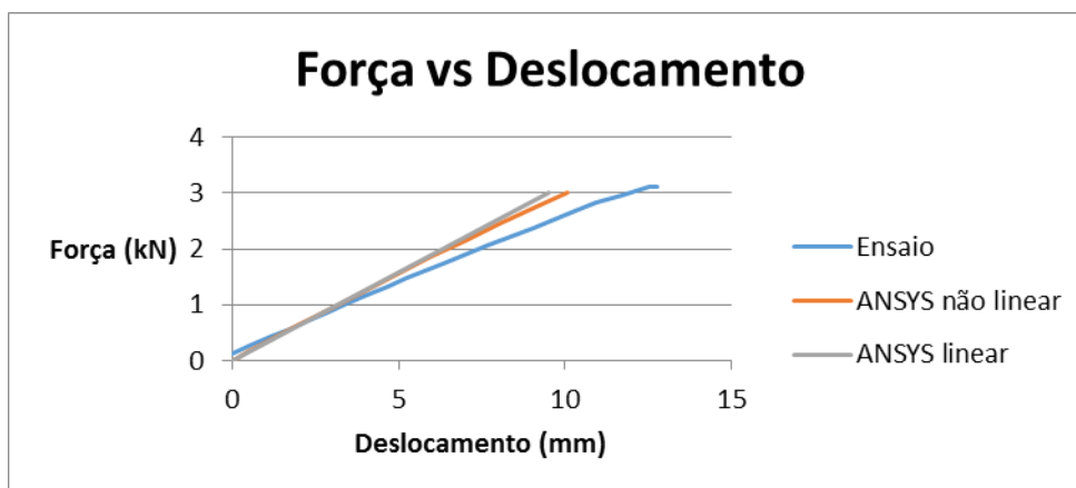
Figura 29 – Comparação de curvas Força vs Deslocamento.
