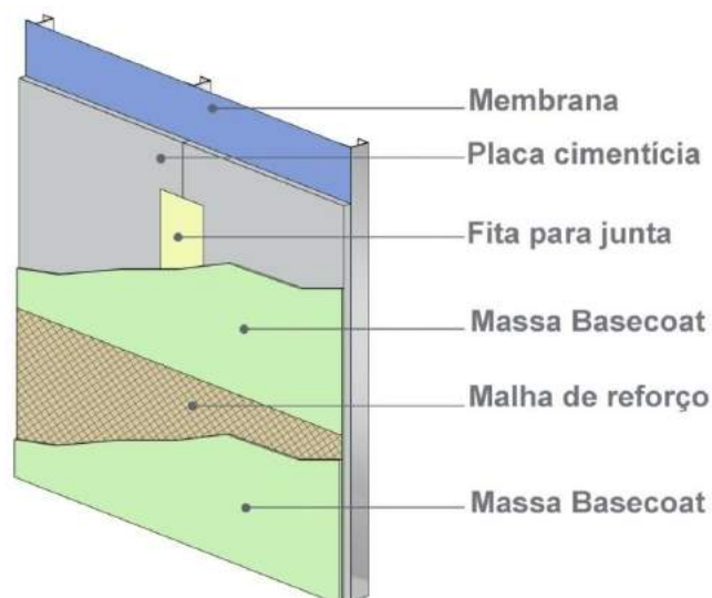
Figura 8: Tratamento de juntas da USG Fonte: Criado pelos autores
