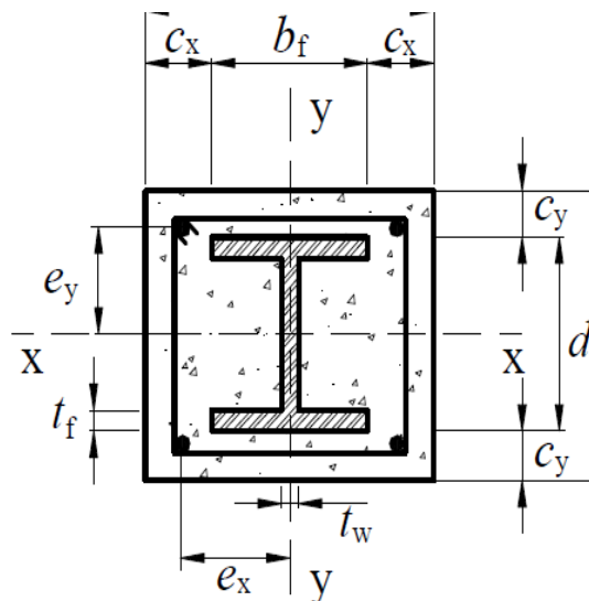
Figura 2 – Seção transversal do pilar misto totalmente revestido.
