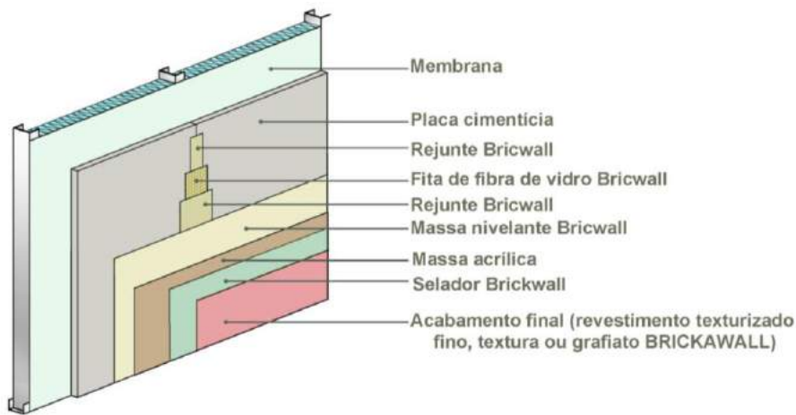
Figura 5: Tratamento de juntas da Bricka Fonte: Criado pelos autores
