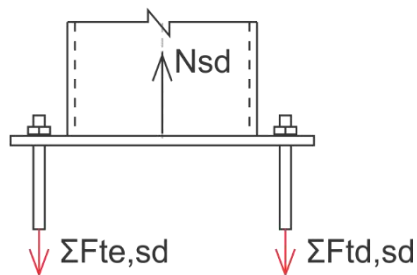
Figura 09 – Situação caso 01 solicitado a esforço de tração
