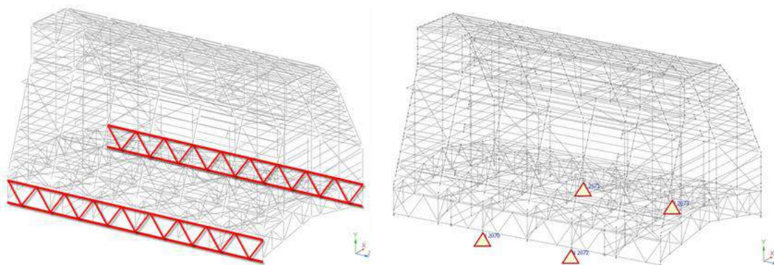
Figura 22. Viga de apeo. Esquema de apoyo para el caso de la etapa de deslizamiento.
