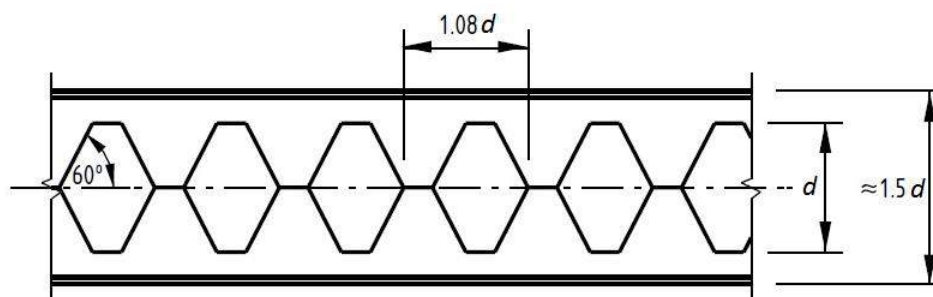
Figura 5 – Viga castelada padrão Anglo-Saxão (BS 5950-1:2000 [5]).
