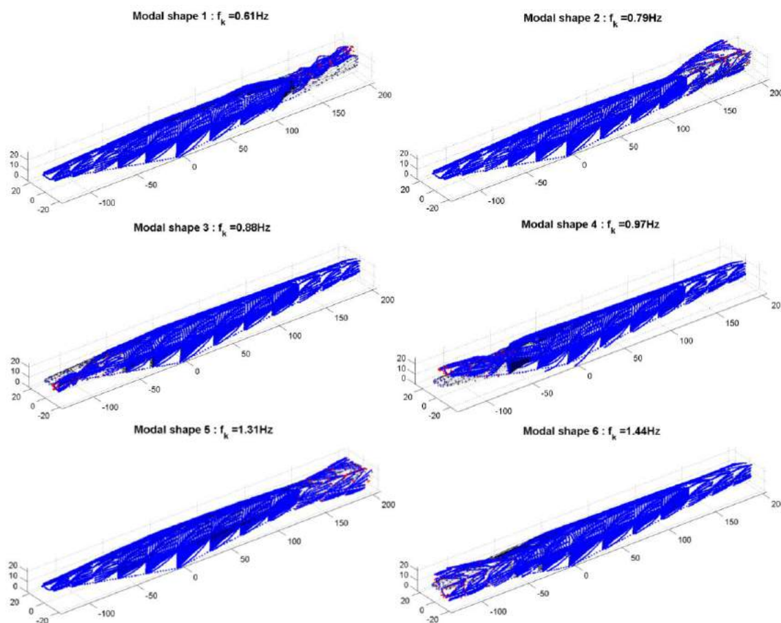
Figura 10 – Formas modais e frequências naturais de vibração livre.
