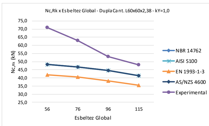
Figura 14 - Resultados analíticos para dupla cantoneira – rótula na direção y - MLE
