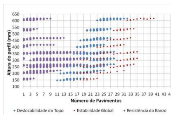
Figura 28 - Relação entre vão da laje e número de da torre e perfis em aço AR345 com laje maciça.
