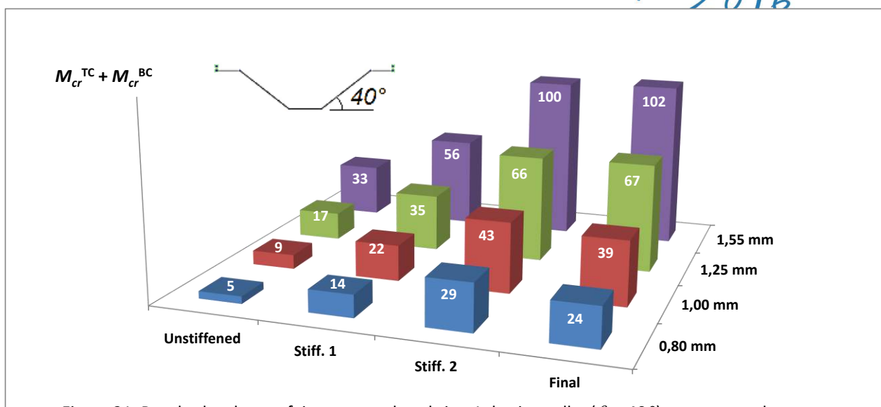
Figura 21: Resultados do aperfeiçoamento do subtipo 1 de viga-calha ( \theta = 40^\circ ), em termos de amplitude de momentos críticos de flambagem ( M_{cr}^{TC} + M_{cr}^{BC} ).
