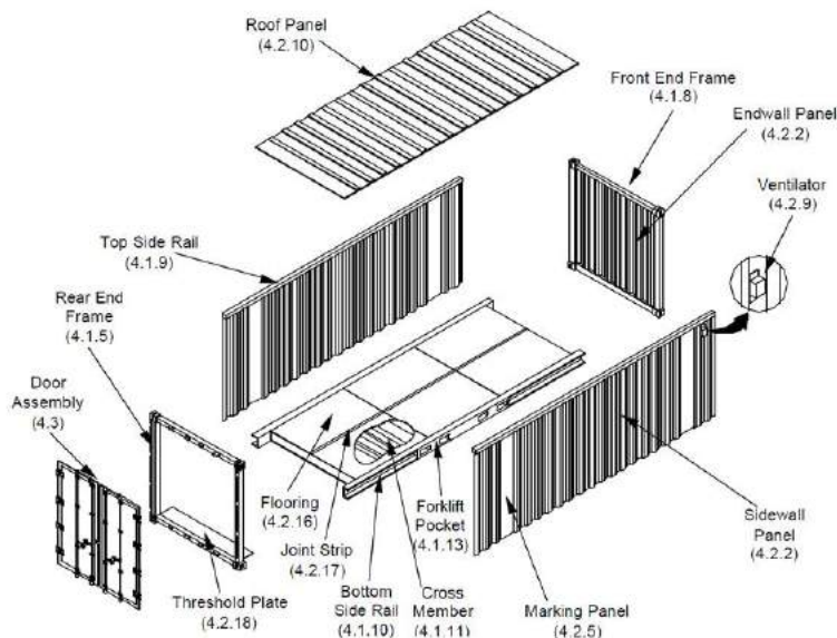
Figura 6: Estrutura secundária do container. Fonte: Residential Shipping Container Primer [13].
