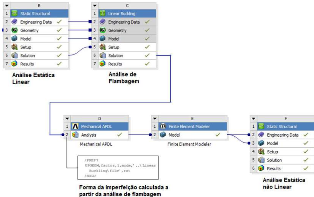
Figura 9 – Fluxograma de análises de elementos finitos realizadas no programa ANSYS.
