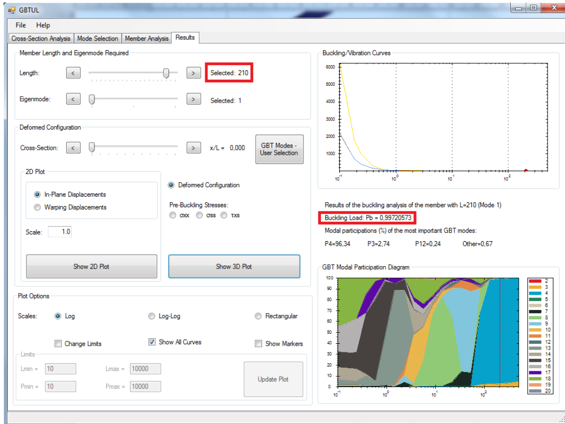
Figura 17 – Resultados do programa GBTUL ( M_{cre} = 0,997 \text{ kN.m} , L_{flamb} = 210 \text{ cm} ).
