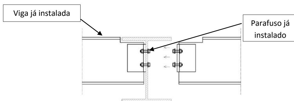
Figura 9 - Conexão com parafusos compartilhados não permitem a instalação posterior de outras vigas e podem comprometer a estratégia de montagem. Fonte: os autores.
