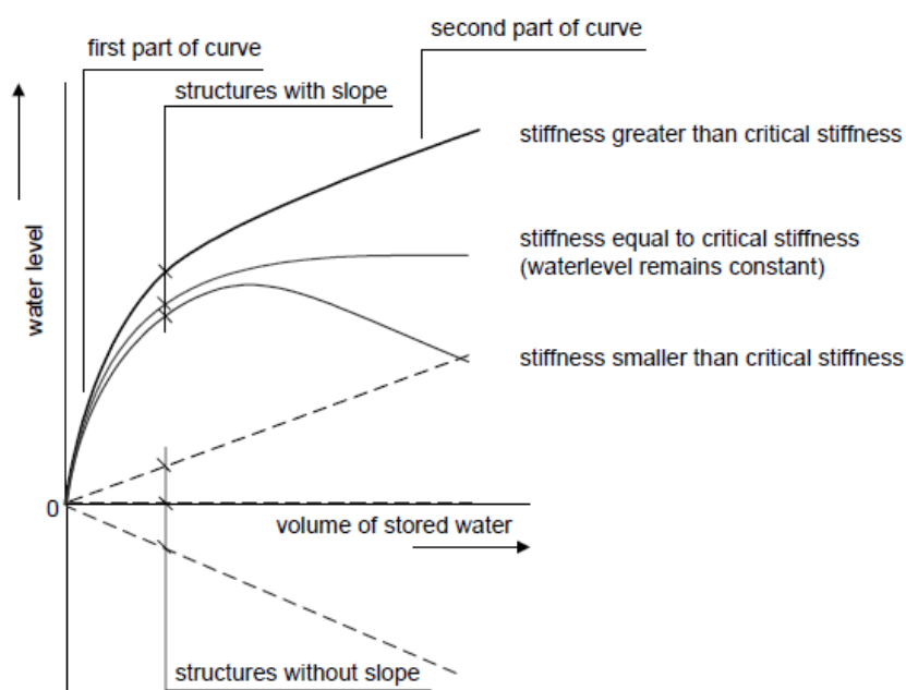
Figura 06 – Gráfico mostrando a relação entre volume armazenado e lâmina d'água para diferentes rigidezes.
