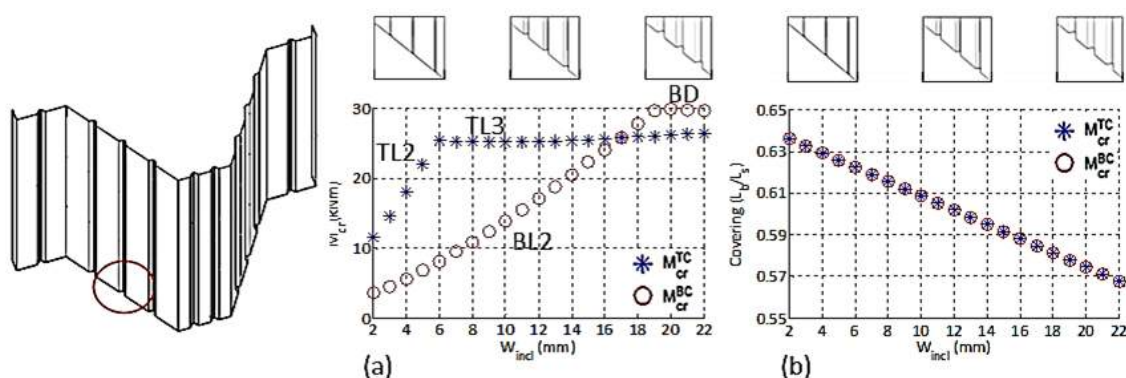
Figura 13: Tendências resultantes da variação da largura da parede inclinada de enrijecedores trapezoidais na alma ( 45^\circ , w_{\text{mid}} = 5 \text{ mm} ): (a) momentos críticos associados à compressão da mesa superior e inferior e (b) taxa de cobertura.
