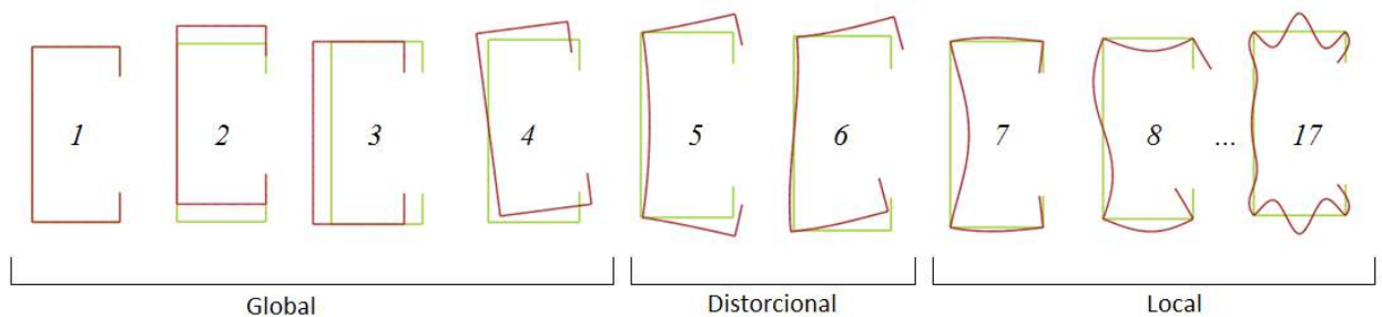
Figura 5: Modos de flambagem adotados com auxílio do programa computacional GBTUL.
