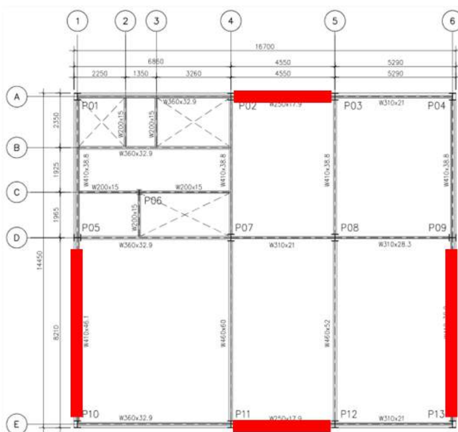
Figura 2 - Planta com a localização das treliças verticais Fonte: As autoras (2016).
