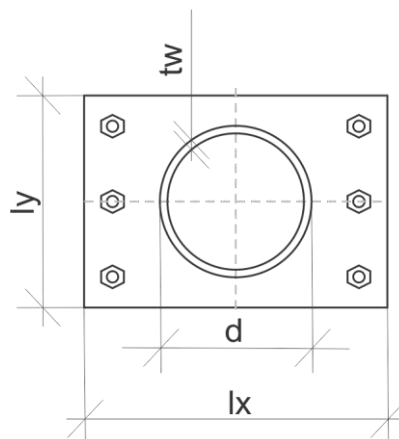
Figura 02 – Base retangular para pilar metálico de seção circular
