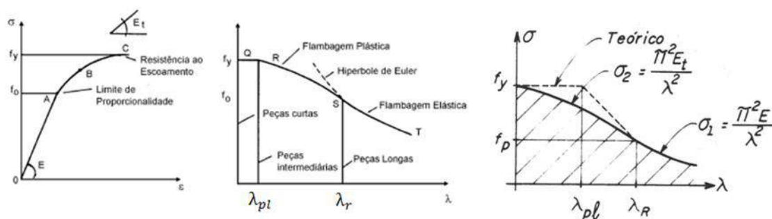
Figura 8 – Delimitação da ocorrência de flambagem elástica e de flambagem inelástica em função dos índices de esbeltez \lambda_r e \lambda_{pl} .
