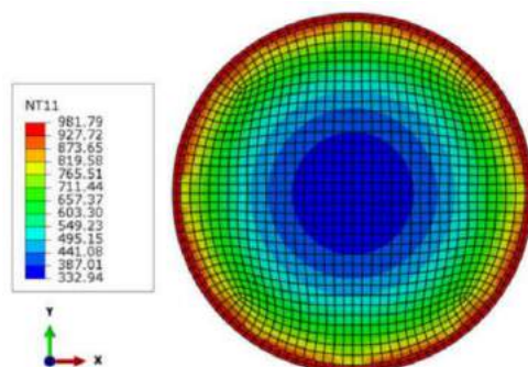
Figura 12: Distribuição de Temperatura na Seção Transversal
