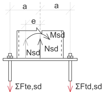
Figura 12 – Distância entre o eixo dos chumbadores e o centro da placa.
