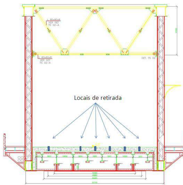
Figura 07 – Local de retirada dos corpos de prova de concreto
