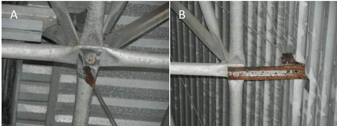
Figura 6 – Estado inicial da estrutura (A- ligação de cabos com a coberta; B- Ligação platibanda com coberta)
