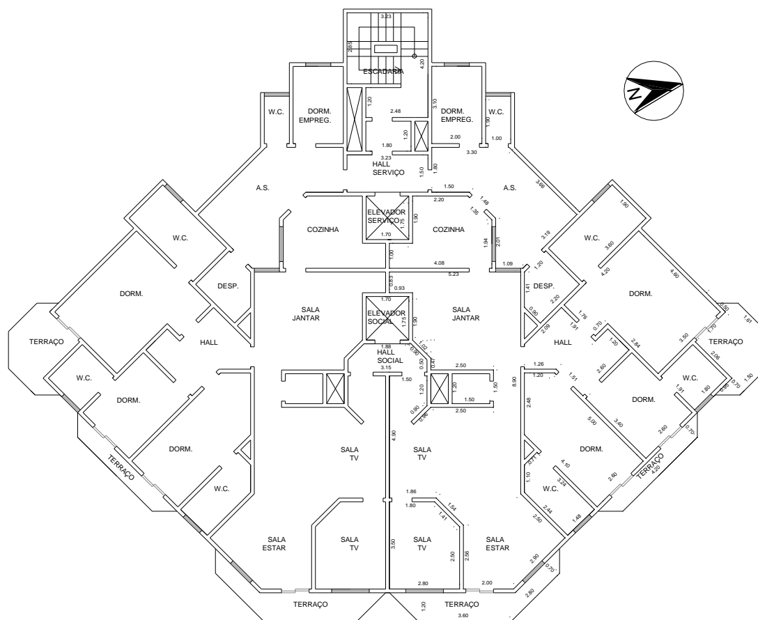
Figura 10: Planta do pavimento-tipo – Residencial San Marcos.
