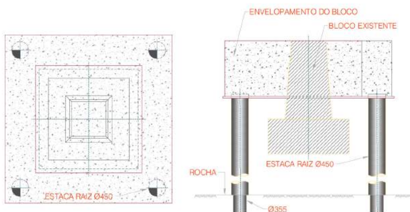
Figura 9: Reforço típico das bases dos vãos de acesso da Ponte Hercílio Luz.
