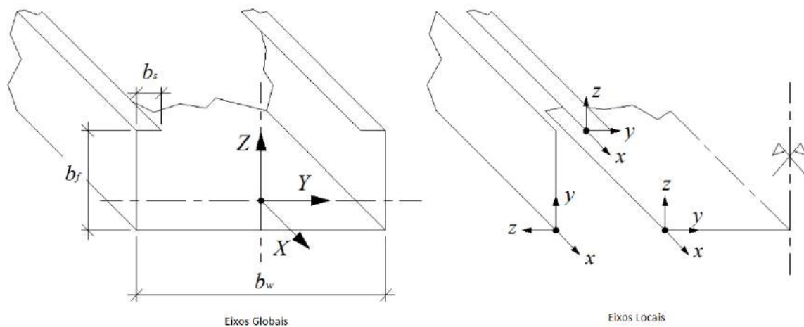
Figura 2: Convenção de eixos em uma seção de chapas dobradas do tipo U enrijecido.
