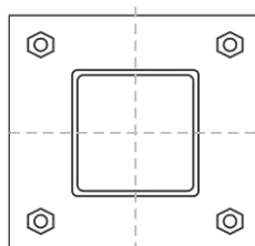
Figura 05 – Base quadrada para pilar metálico de seção quadrada
