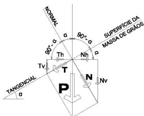
Figura 8 – Decomposição do vetor peso P nas componentes T e N
