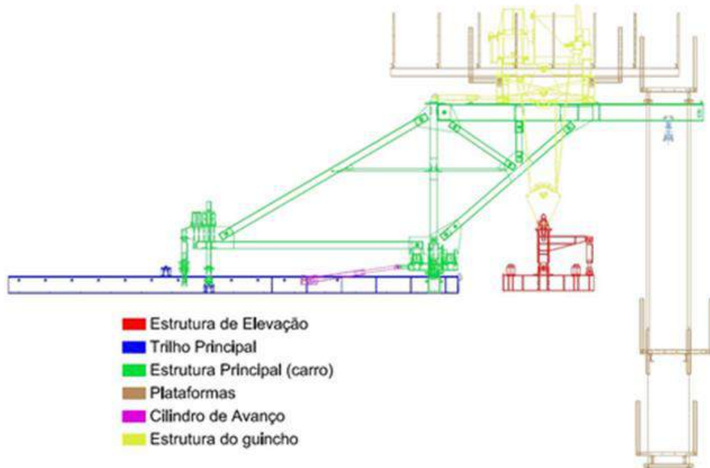
Figura 2 – Identificação dos elementos da treliça içadora de aduelas.
