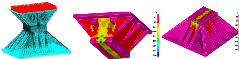
Figura 10: Modelo e distribuição de tensões de von Mises obtidas para o apoio dos pilones [Mpa].
