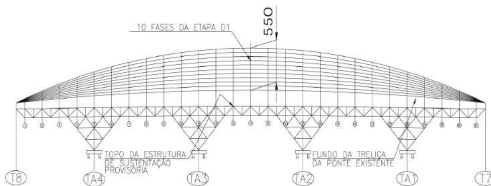
Figura 8: Etapas da Fase 1 da transferência de cargas.
