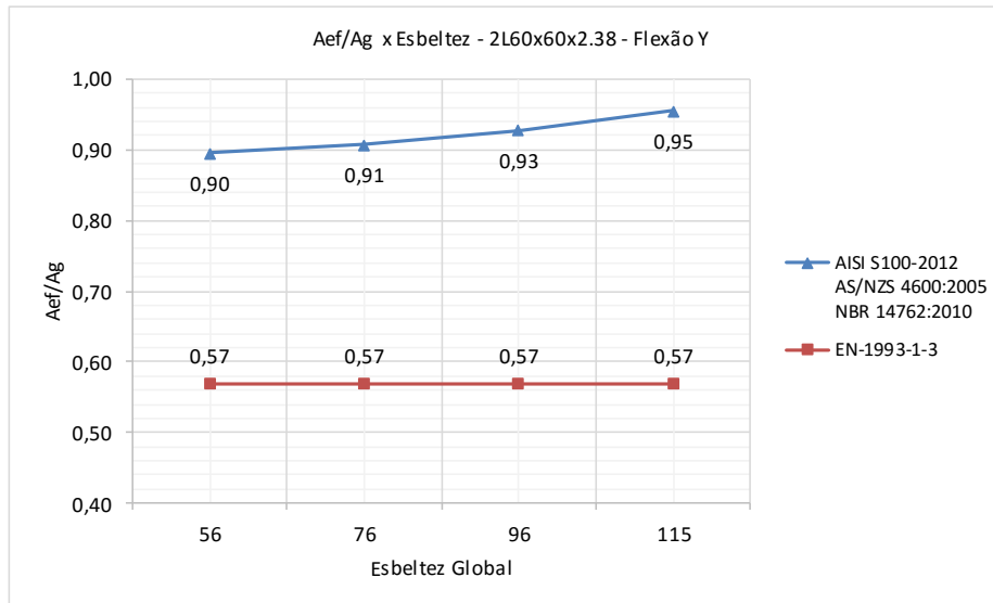
Figura 17 — Resultados analíticos para dupla cantoneira com flexão liberada para eixo Y – A_{ef}/A_g \times E.G. - MLE
