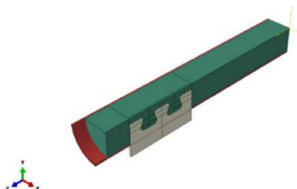
Figura 14: Modelo Numérico do Pilar Misto com o uso do Conector Crestbond
