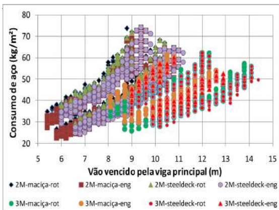
Figura 13 - Consumo de aço dos perfis das vigas em aço MR250. (Fonte: elaborada pelos autores)
