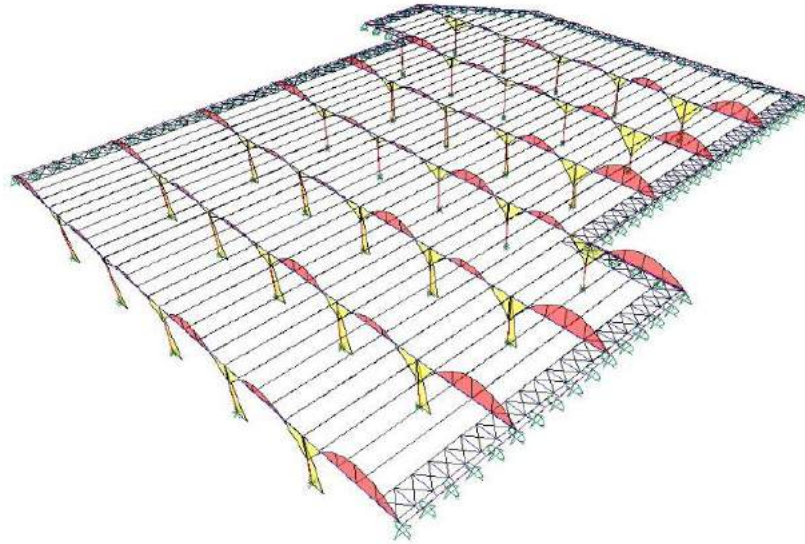
Figura 13 – Imagem do modelo de análise, mostrando a existência de momento fletor nos pilares centrais.
