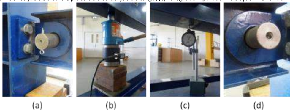
Figura 6 – Ensaio da viga ligada com pino: (a, d) Ligação com pino; (b) atuador hidráulico, célula de carga, placas de compensação de altura e placa de distribuição de carga; (c) relógio comparador na seção inferior da viga.
