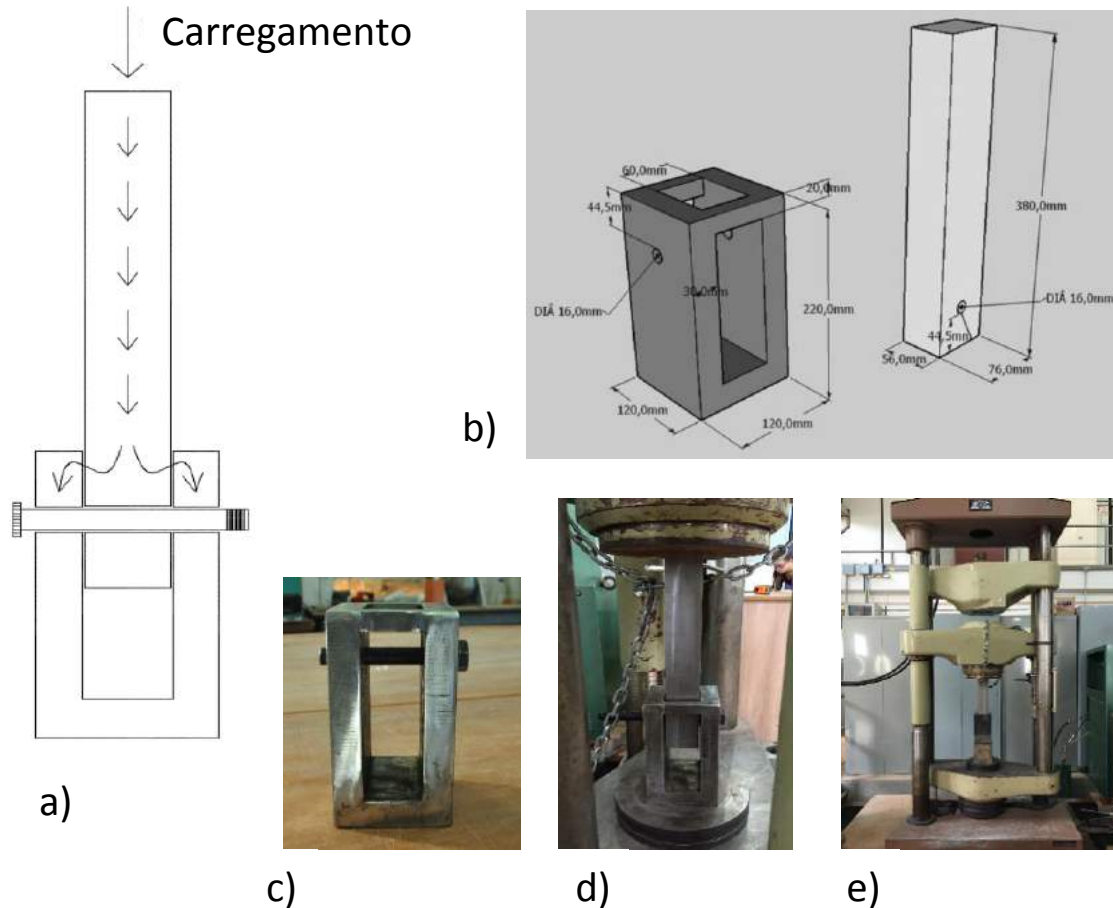
Figura 4 – Concepção do ensaio e aparato de aplicação do carregamento. (a) Distribuição do carregamento aplicado em dois planos de corte; (b) dimensões do aparato de ensaio; (c) parte inferior do aparato de ensaio; (d) e (e) aplicação do carregamento no aparato de ensaio e consequente cisalhamento do parafuso.
