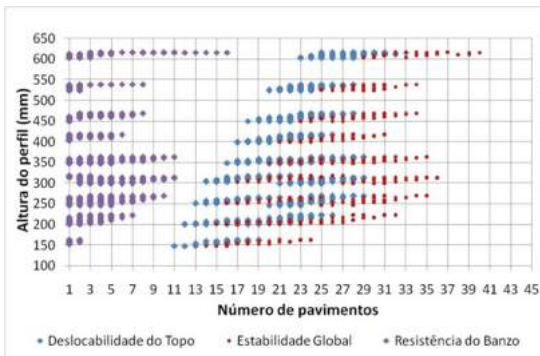
Figura 29 - Relação entre número de pavimentos da torre e perfis em aço MR250 e laje steel-deck. (Fonte: elaborada pelos autores)
