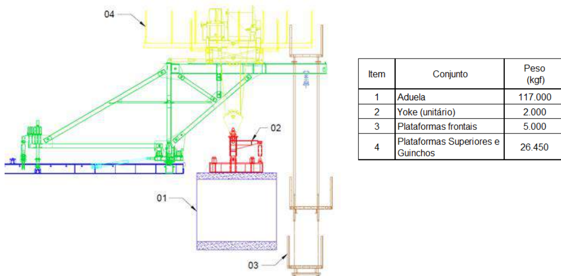
Figura 4 – Pesos dos conjuntos presentes no equipamento da treliça içadora de aduelas.
