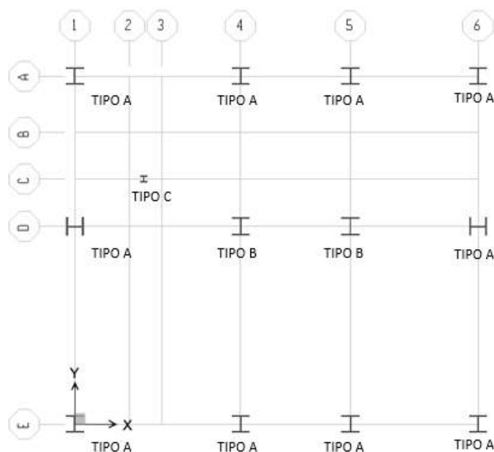
Figura 5 - Legenda de tipos de pilares Fonte: As autoras (2016).
