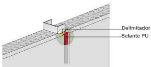
Figura 7 - Tratamento de juntas de dilatação Fonte: Adaptado de Bricka [13].
