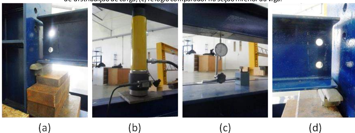
Figura 5 – Ensaio de viga simplesmente apoiada. (a, d) Apoios simples; (b) macaco hidráulico, célula de carga e placa de distribuição de carga; (c) relógio comparador na seção inferior da viga.
