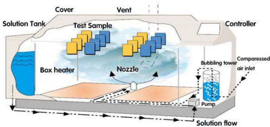
Figura 03: Esquema da câmara de névoa salina
