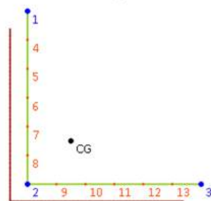
Figura 21 — Resultados para análise numérica via GBTUL para cantoneira L60x60x2.38x1685 – Determinação da carga crítica de flambagem elástica e respectivo modo de falha. Flambagem por flexão em torno do eixo de menor inercia 99,81%.
