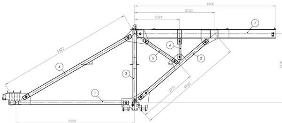
Figura 3 – Estrutura da treliça içadora de aduelas.
