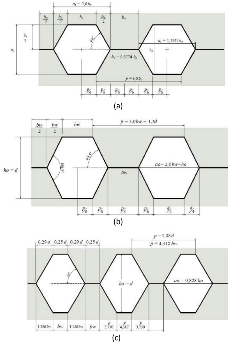
Figura 6 - Geometria dos padrões (a) Litzka (b) Peiner e (c) Anglo-saxão (fonte: Silveira [2]).
