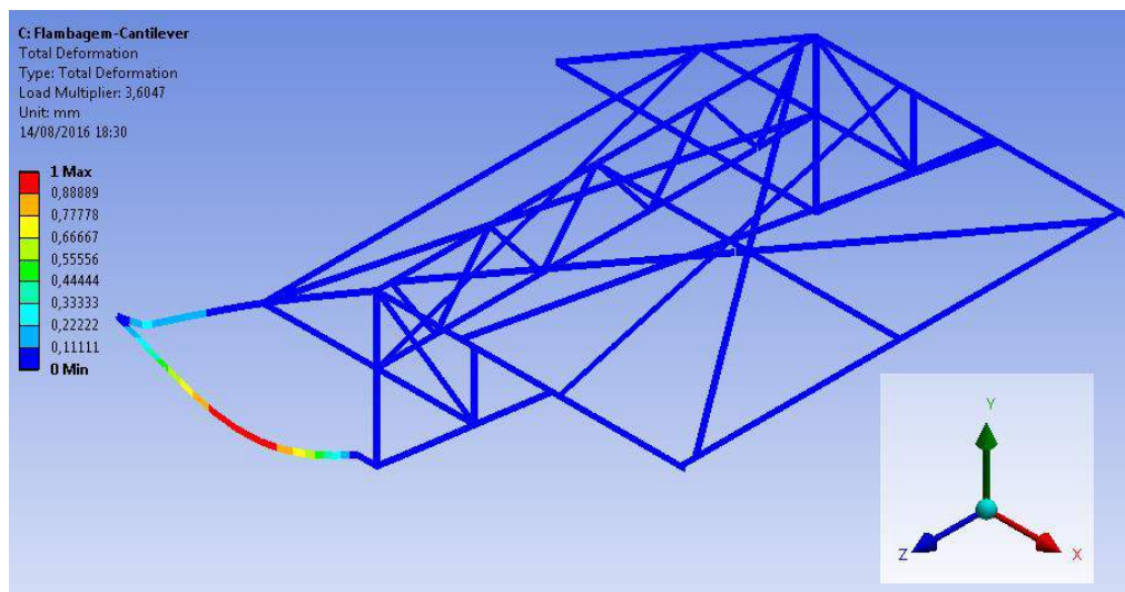
Figura 10 – Resultado do primeiro autovalor de \lambda_1 = 3,6047 .
