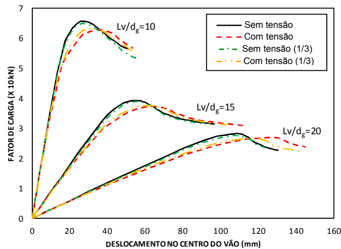
Figura 19 - Curvas de resistência para o perfil W 410x38,8, padrão celular.
