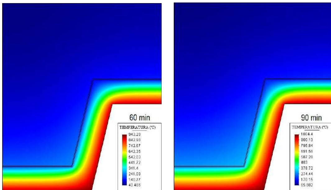
Figura 5 – Resultados da análise térmica para TRRF de 60 min e 90 min
