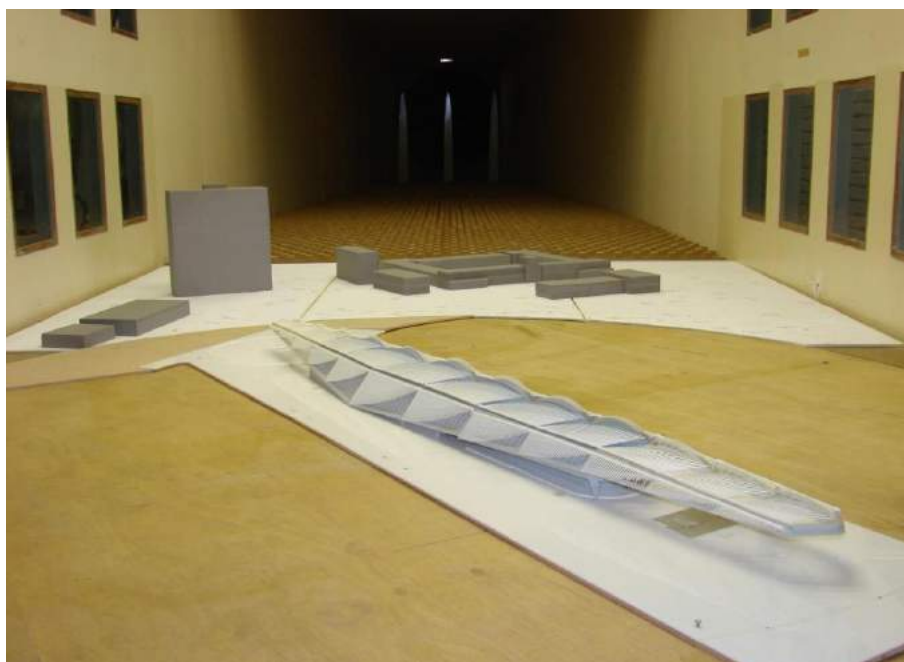
Figura 2 – Modelo reduzido do Museu do Amanhã no interior do túnel de vento.
