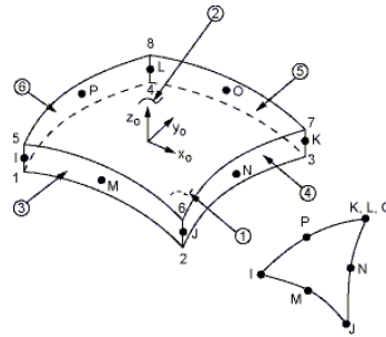
Figura 20 – Elemento Finito SHELL281 (Fonte: [7]).
