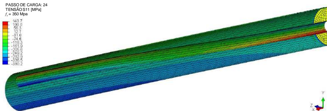
Figura 14 – Modelo 17 sem travamentos – Tensões atuantes – Passo de carga 24 ( \lambda_0 = 1,07 e \lambda = 80 )
