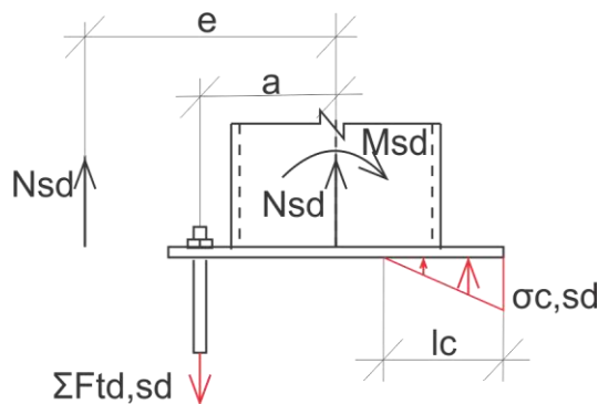
Figura 14 - Situação caso 03 solicitada a esforço de tração
