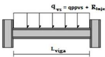
Figura 3 – Viga secundária. (Fonte: elaborada pelos autores).
