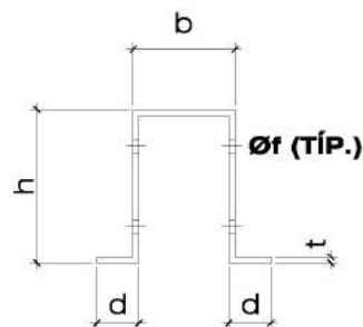
Figura 3 – Terça em perfil “cartola”
