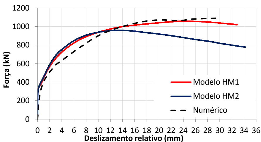
Figura 11 - Curvas força versus deslizamento experimental e numérico
