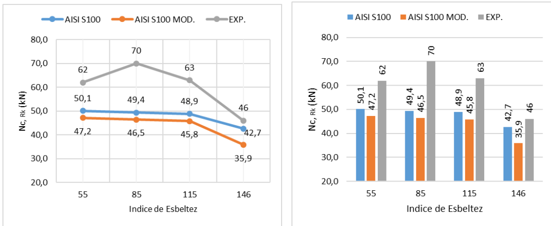
Figura 23 – Cantoneira dupla – flexão em X
