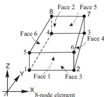
Figura 3 - Elemento de Malha C3D8 - adaptado de Starossek & Falah [6]
