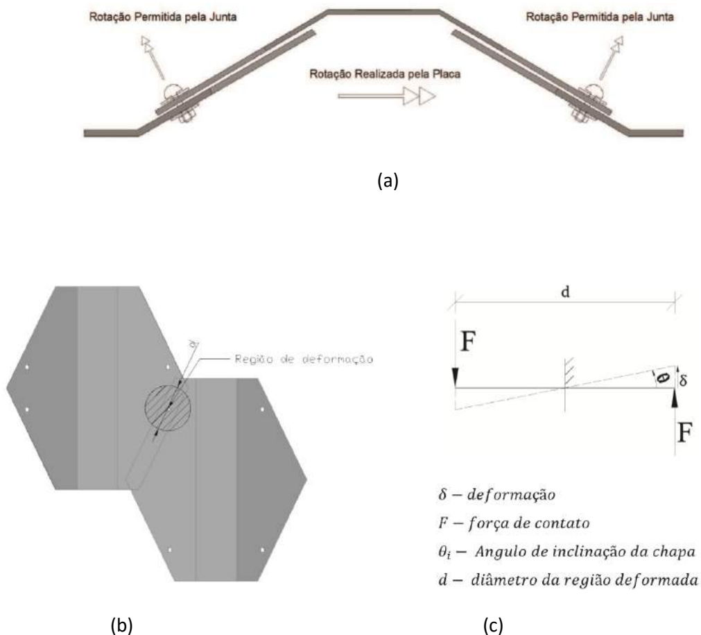
Figura 11 – Considerações de DIAS (2015) para determinar valor de “ k ”.
