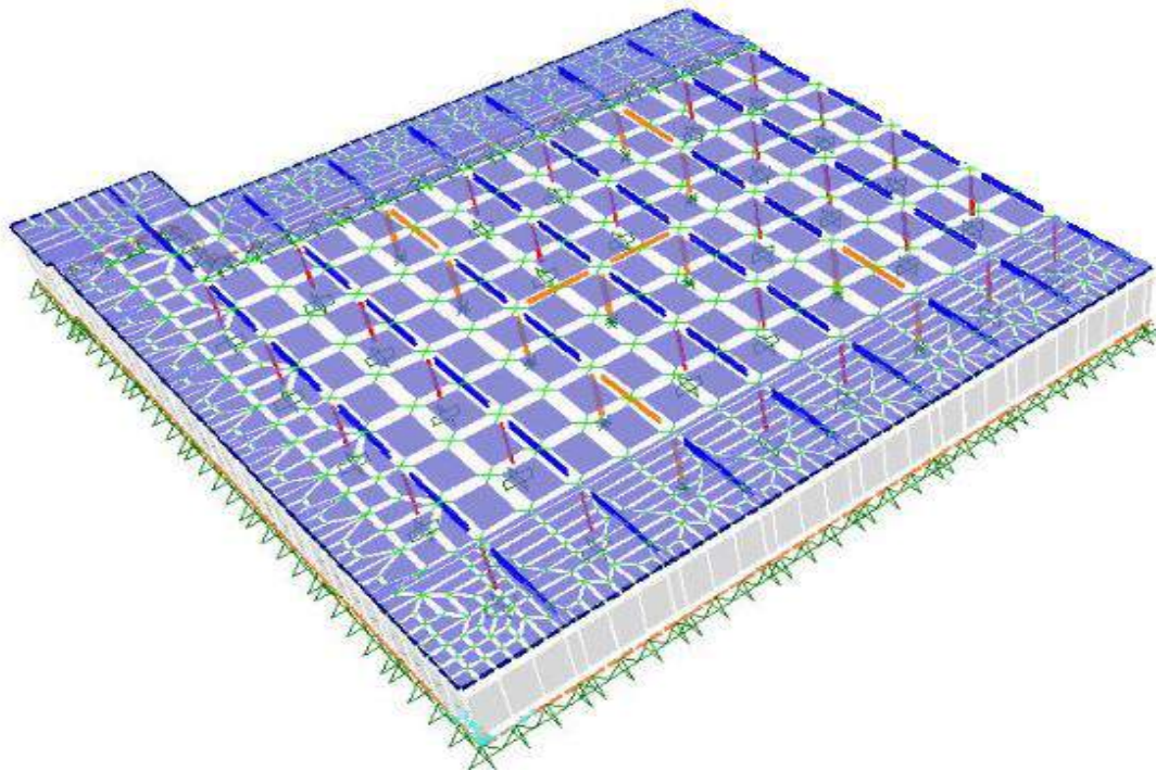
Figura 12 – Modelo de análise no sistema “roof deck”, aonde, o diafragma é simulado por uma malha de elementos “shell”.
