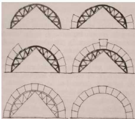
Figura 13 – Sequência de execução de um arco com apoios provisórios (DIAS, 2015).
