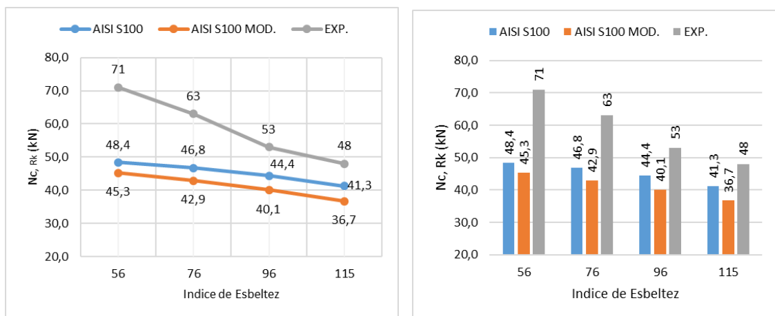
Figura 24 – Cantoneira dupla – flexão em Y
