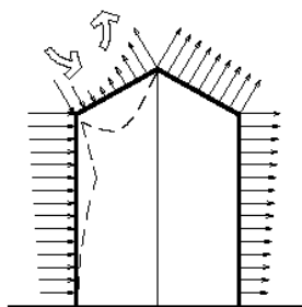
Figura 12 – Sobrepressão no teto a barlavento
