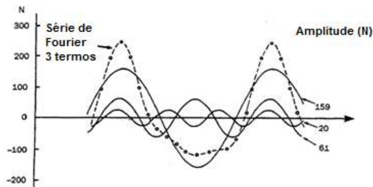
Figura 5 - Componentes harmônicas da série de Fourier para caminhada [10].
