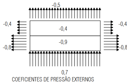
Figura 16 – Coeficientes de Pressão obtidos pela ABNT NBR 6123:1988 para o vento a 90º
