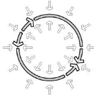
Figura 10 – Anel sob esforços axiais provocados por cargas radiais
