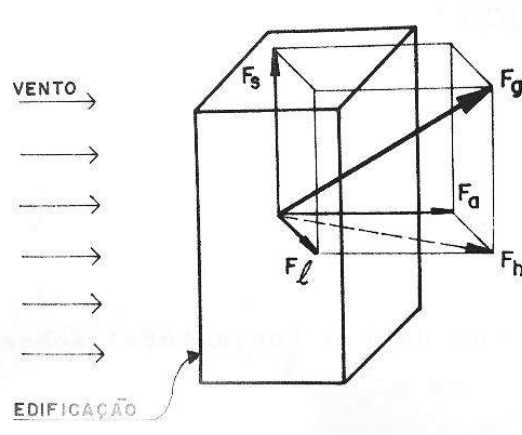
Figura 5 - Forças aerodinâmicas sobre uma edificação. Pitta [1987].
