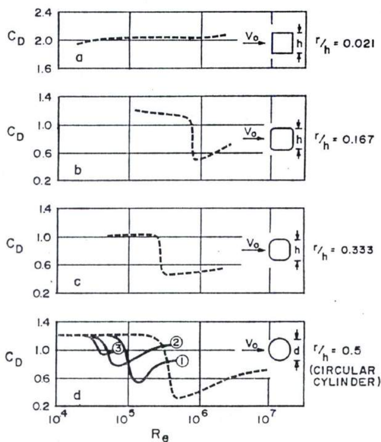
Figura 4 - Influência da variação do número de Reynolds sobre o coeficiente de arrasto de acordo com a forma da seção transversal. Os números 1, 2 e 3 na última figura representam rugosidades diferentes da superfície da seção circular e têm efeito semelhante ao de uma variação da turbulência no escoamento incidente [3].
