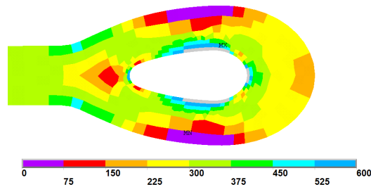
Figura 11: Tensões de von Mises nas extremidades das barras de olhal [Mpa].
