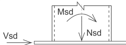
Figura 06 – Solicitações provenientes da estrutura com esforço normal de compressão
