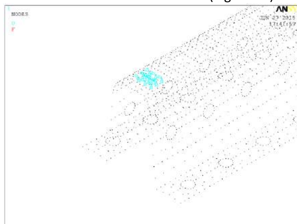
Figura 24 – Modelação das condições de apoio.
