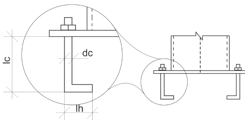
Figura 15 – Dimensões do chumbador formado com extremidade inferior a 90
