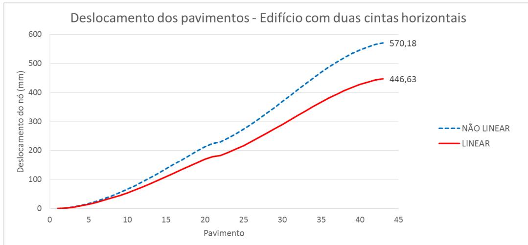
Gráfico 3 - Deslocamentos no edifício com treliças verticais e duas treliças horizontais Fonte: As autoras (2016).
