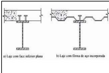
Figura 8 – Viga Mista
