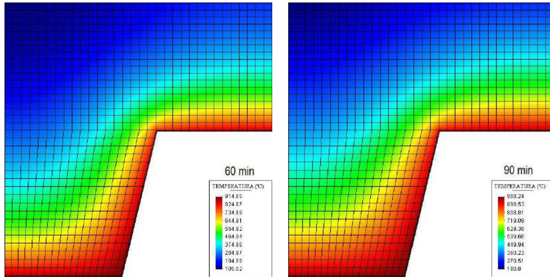
Figura 3 – Resultados da análise térmica para TRRF de 60 min e 90 min
