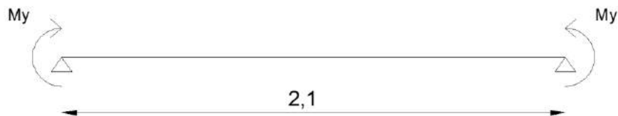
Figura 16 – Momento fletor aplicado para análise de estabilidade no ANSYS (medidas em metros).
