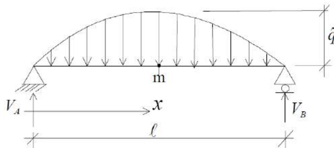
Figura 08 – Carregamento senoidal aproximado.
