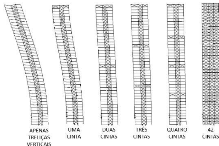
Figura 7 - Modelos deformados em análise não-linear (P-Delta) (escala 20x) Fonte: As autoras (2016).
