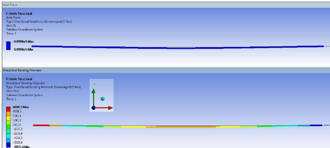
Figura 14 – Resultados de força axial e de momento fletor atuantes na barra crítica da treliça içadora de aduelas - Condição de desvio de eixo da barra de 10 mm.
