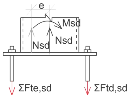
Figura 11 - Situação caso 02 solicitado a esforço de tração
