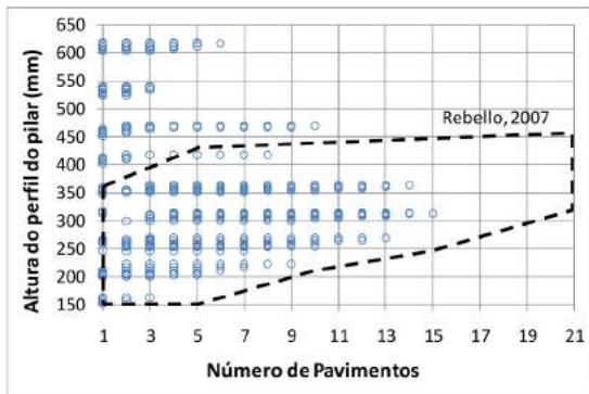
Figura 20 - Relação do número de pavimentos e perfis do pilar em aço AR345 e laje steel-deck. (Fonte: elaborada pelos autores)
