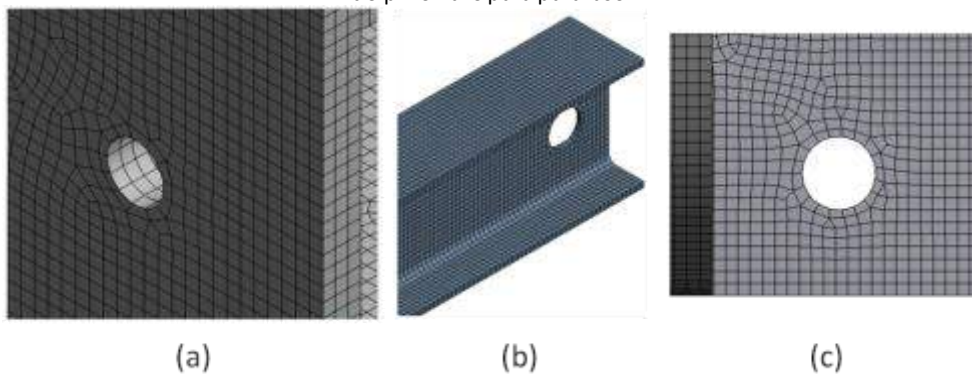
Figura 10 – Malha na coluna, viga e suporte do pino. (a) Detalhe da coluna; (b) Viga: região da ligação; (c) Suporte do pino: furo para parafuso.
