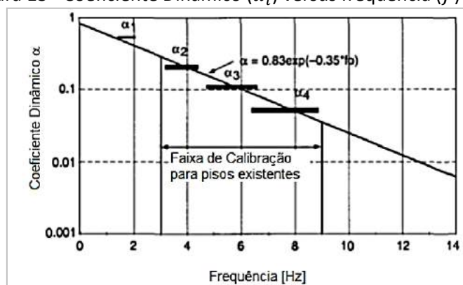
Figura 13 - Coeficiente Dinâmico ( \alpha_i ) versus frequência ( f ) [23].
