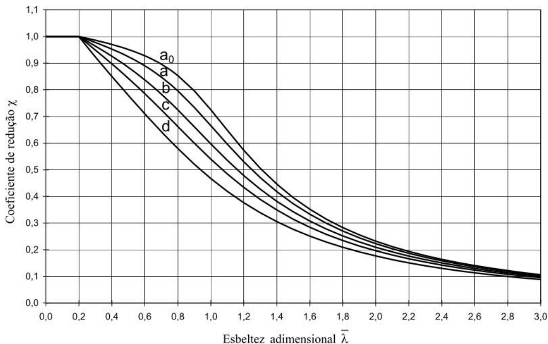
Figura 2 — Valor de \chi em função do índice de esbeltez adimensional \bar{\lambda} Fonte: Eurocode EN-1993-1-1
