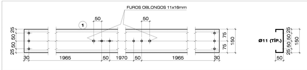
Figura 2 – Exemplo de furação em terça metálica
