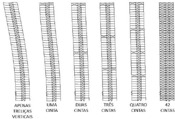
Figura 6 - Modelos deformados em análise linear (escala 20x) Fonte: As autoras (2016).
