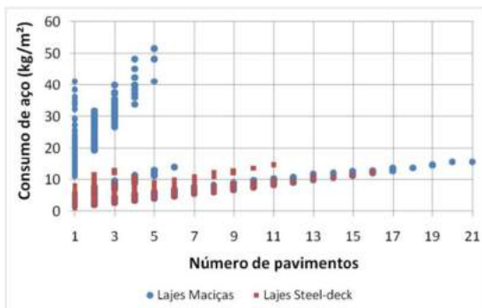
Figura 21 - Consumo de aço dos pilares de perfis em aço MR250. (Fonte: elaborada pelos autores)
