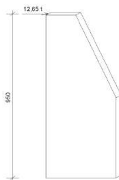
Figura 18 – Modelo de enrijecedor (Fonte: Elaborada pelo autor)
