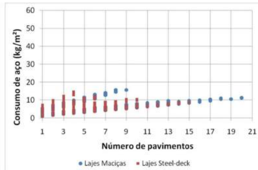
Figura 22 - Consumo de aço dos pilares de perfis em aço AR345. (Fonte: elaborada pelos autores)
