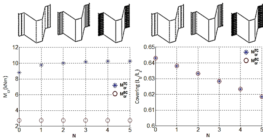
Figura 11: Tendências resultantes da inclusão de enrijecedores trapezoidais (larguras de 5 mm, 45°) na mesa superior: (a) momentos críticos associados à compressão da mesa superior e inferior e (b) taxa de cobertura
