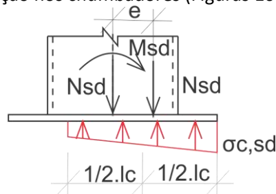
Figura 10 - Situação caso 02 solicitado a esforço de compressão
