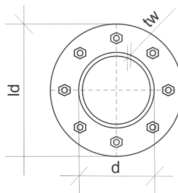
Figura 03 – Base circular para pilar metálico de seção circular
