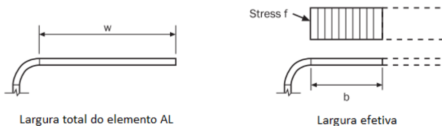
Figura 5 — Largura total e efetiva de um elemento AL Fonte: AISI S100-2007
