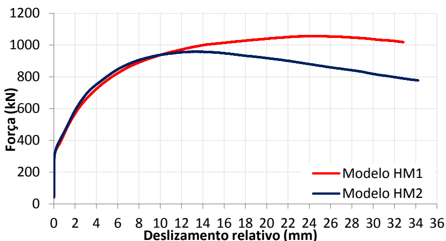
Figura 8 - Curvas força versus deslizamento dos modelos experimentais
