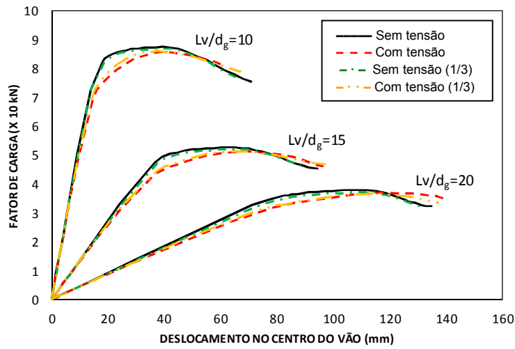
Figura 21 - Curvas de resistência para o perfil W 410x60,0, padrão celular.
