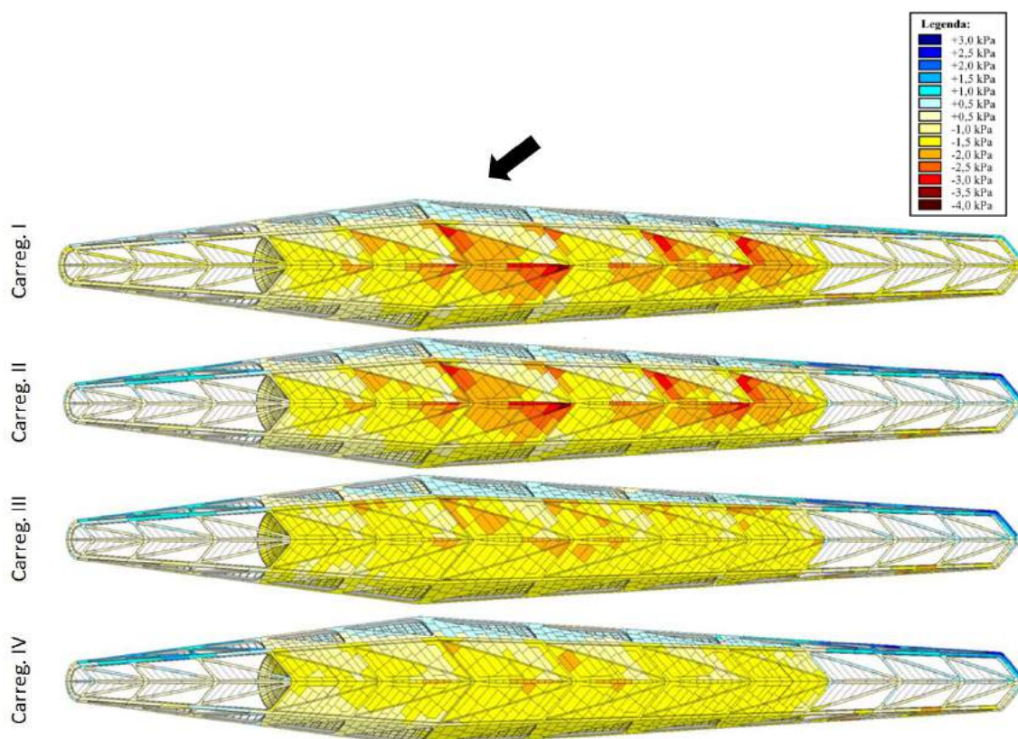
Figura 9 – Carregamentos I a IV para ângulo 150°.
