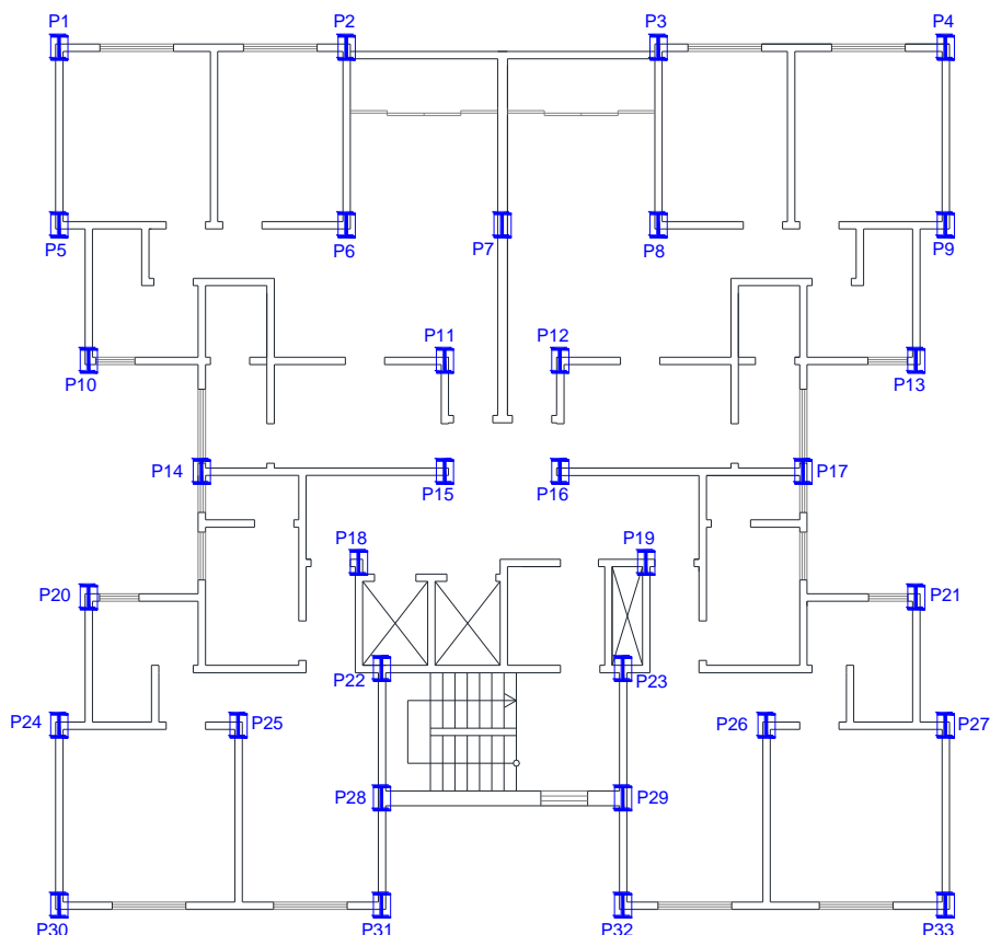
Figura 6: Localização dos pilares de aço em planta – Residencial Navarro.
