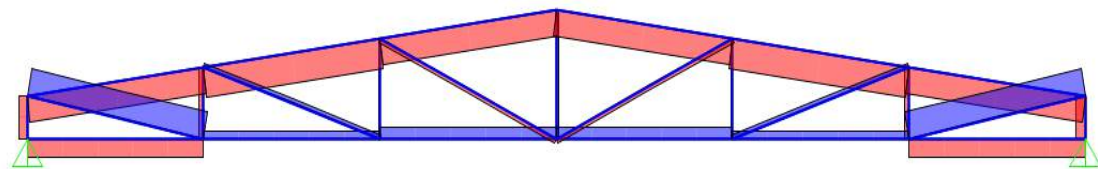
Figura 12: Esforços causados pelo peso próprio da estrutura
