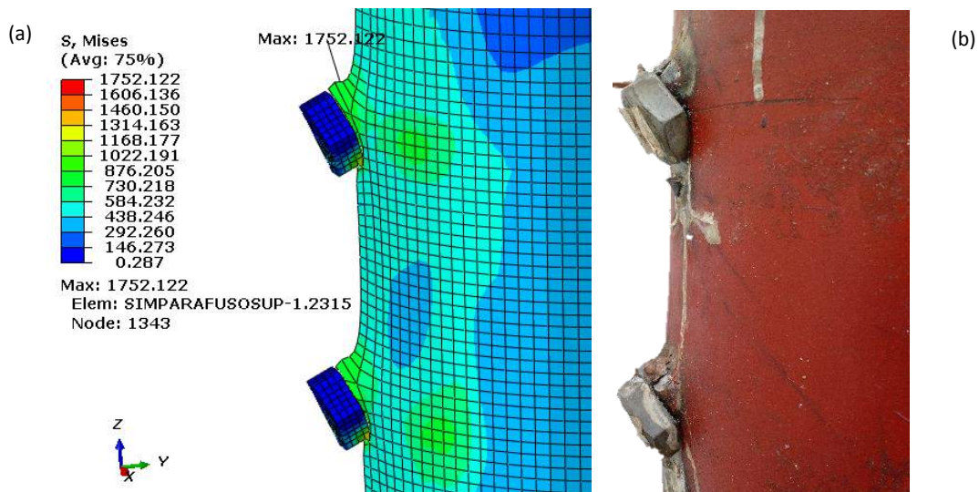
Figura 15 - Variação das tensões de von Mises ; (b) tubo de aço e cabeça do parafuso após a ruptura;
