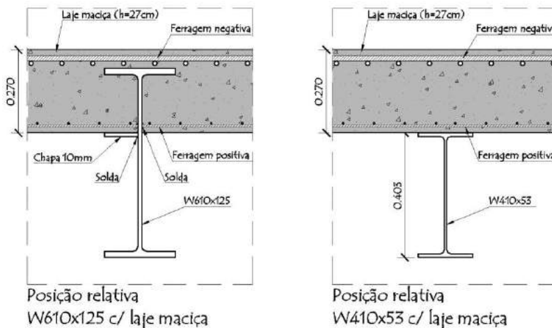
Figura 17 – Posição relativa da laje sem os conectores de cisalhamento (residência AE)
