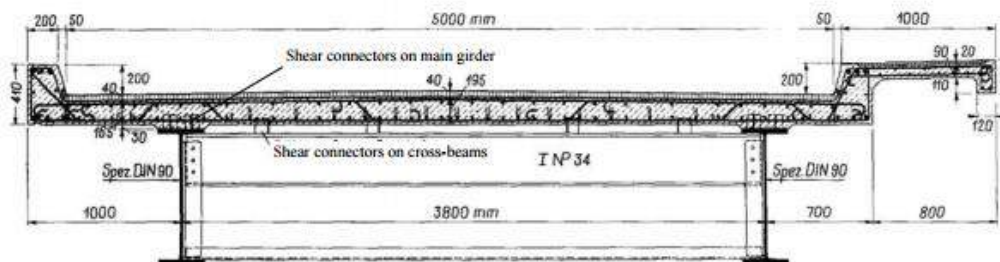
Figura 1 – Seção transversal do viaduto Willerzeller (1936)
