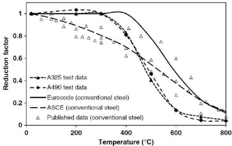
Figura 1 - Fator de redução dos parafusos e aço convencional. (Eixo x: Temperatura (°C), Eixo y: Fator de Redução). Fonte: Kodur (2012)
