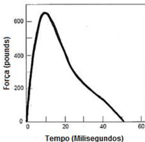
Figura 3 – Função do teste impacto do calcanhar [7].
