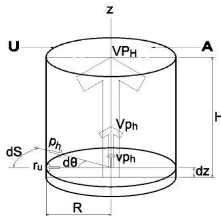
Figura 6 – Conceito de vetores na conversão de p_h em v_{ph}
