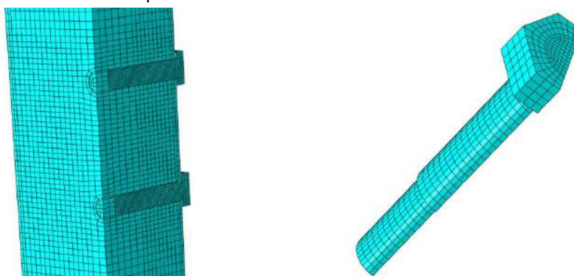
Figura 4 - Malha de elementos finitos: (a) em torno dos conectores; (b) conector
