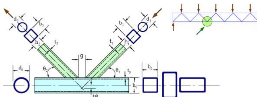
Figura 2: Símbolos usados para ligações do tipo K [11]
