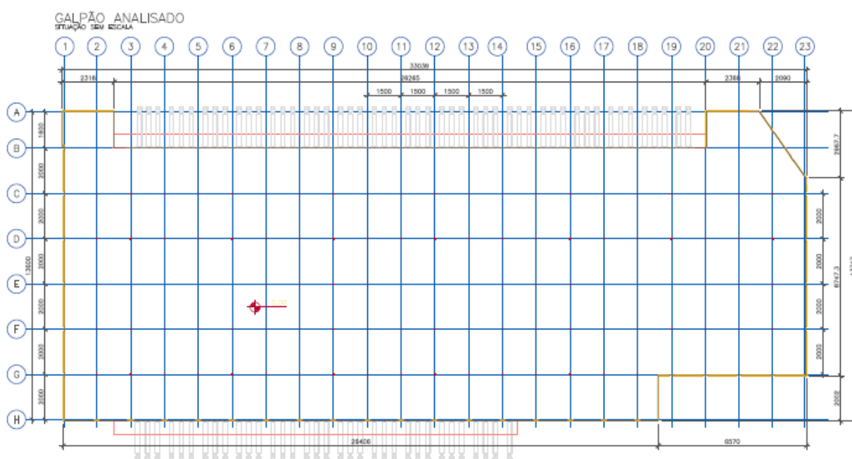
Figura 10 – Imagem da geometria do galpão a ser apresentado no estudo de caso.
