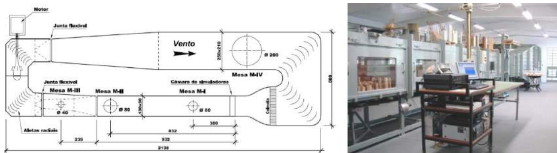
Figura 5 – Túnel de Vento Professor Joaquim Blessmann do LAC/UFRGS.
