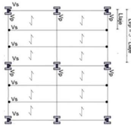
Figura 2 – Sistema de piso 3M. (Fonte: adaptado de Brito e Silva [8]).
