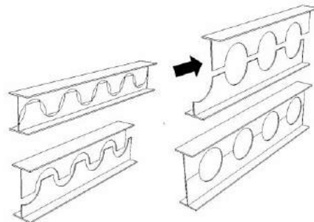
Figura 2 - Processo de obtenção de vigas alveolares com abertura circular (fonte: Silveira [2]).
