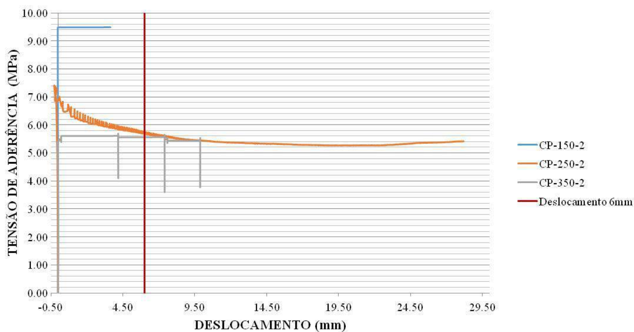
Figura 6 - Tensão de aderência versus deslizamento dos corpos de prova com seção circular.
