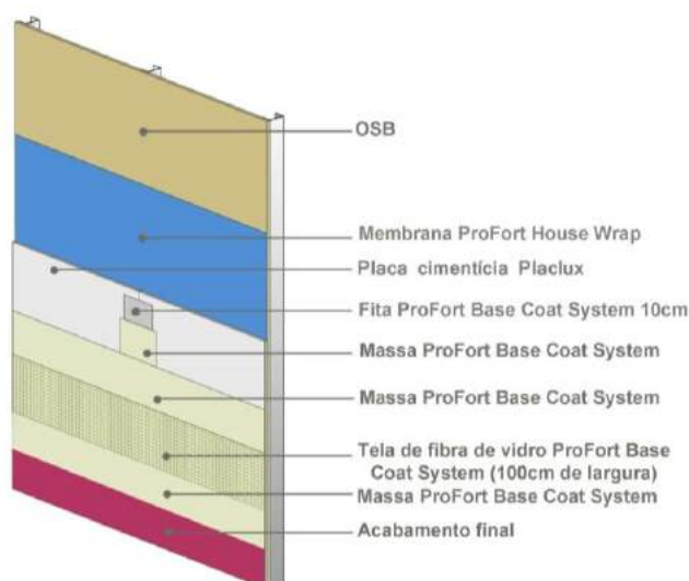
Figura 4: Tratamento de juntas da Placlux
