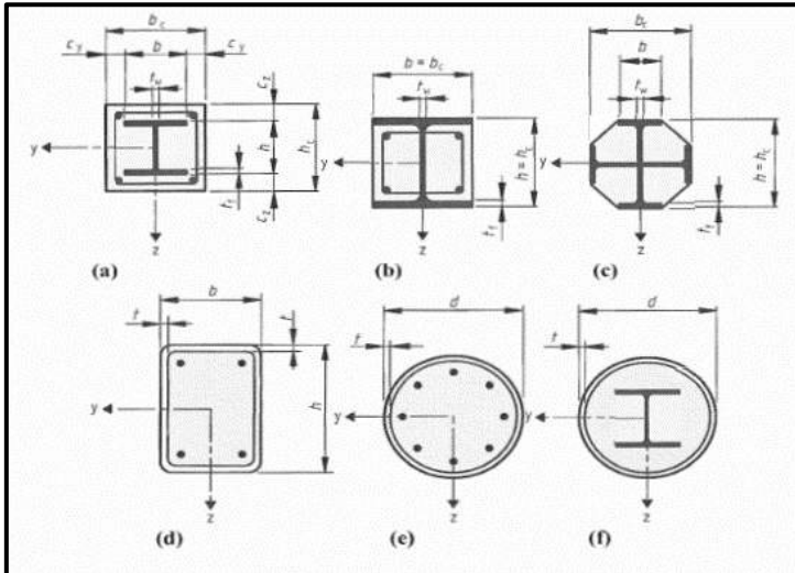
Figura 10 – Pilares Mistos
