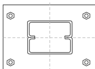
Figura 04 – Base circular para pilar metálico de seção duplo U enrijecido
