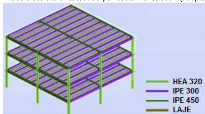
Figura 11 - Modelo estrutural estudado por Costa-Neves et al. (adaptado de [28]).
