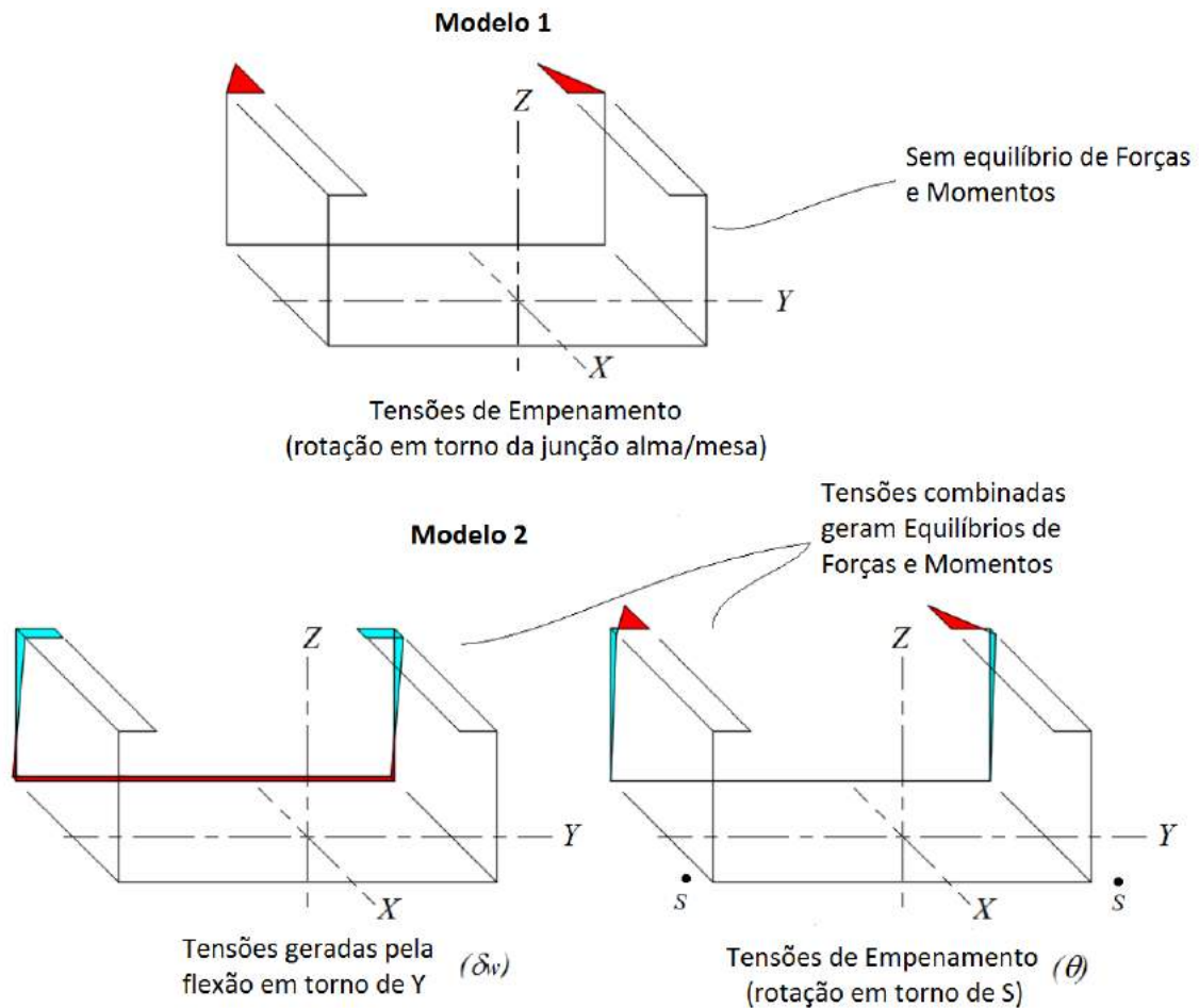
Figura 4: Tensões normais nos Modelos 1 e 2.
