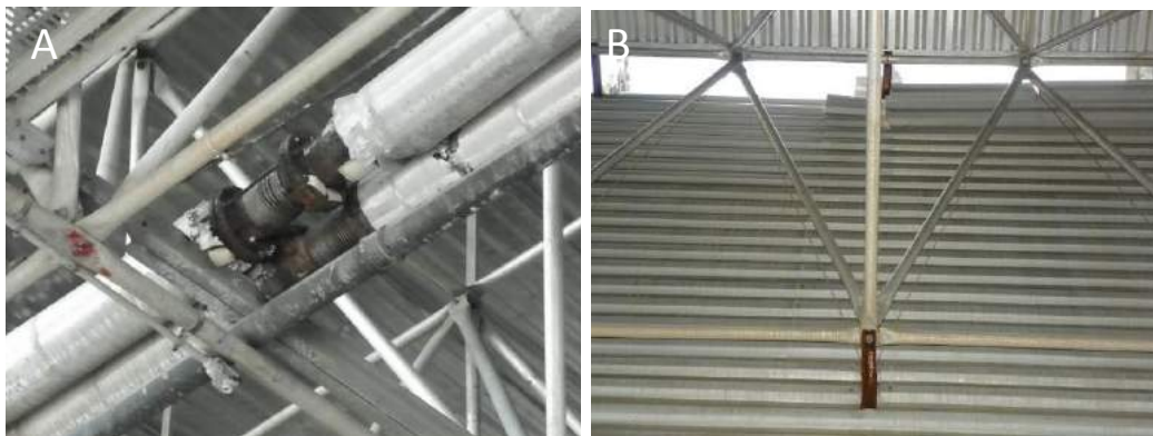
Figura 14 – Contato de metais diferentes (A- Tubos de aço em contato com tubo de alumínio; B- perfil de aço ligado na cobertura de alumínio)
