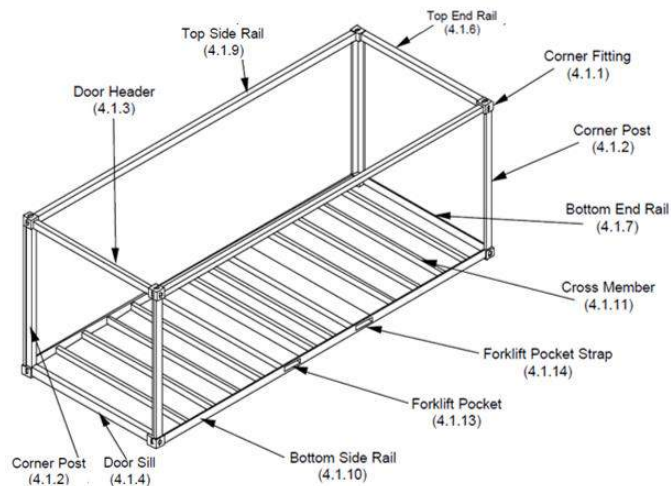
Figura 5: Estrutura primária do container. Fonte: Residential Shipping Container Primer [13].
