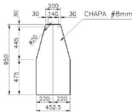
Figura 17 – Dimensões finais da chapa-montante (Fonte: Elaborada pelo autor)
