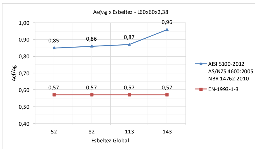
Figura 15 — Resultados analíticos para cantoneira simples – A_{ef}/A_g x E.G. - MLE
