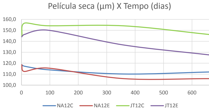
Figura 30: Comparativo gráfico entre corpos de prova com a mesma camada de película seca ( 120\mu\text{m} )
