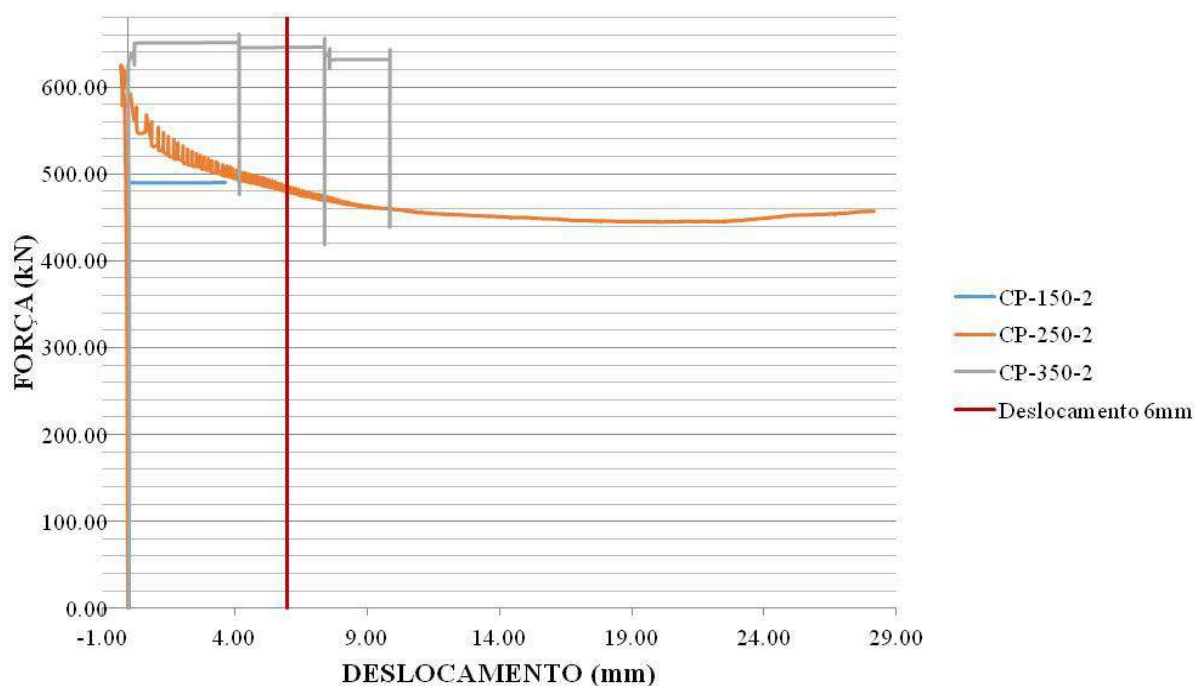
Figura 5 - Força versus Deslizamento perfis de seção circular.
