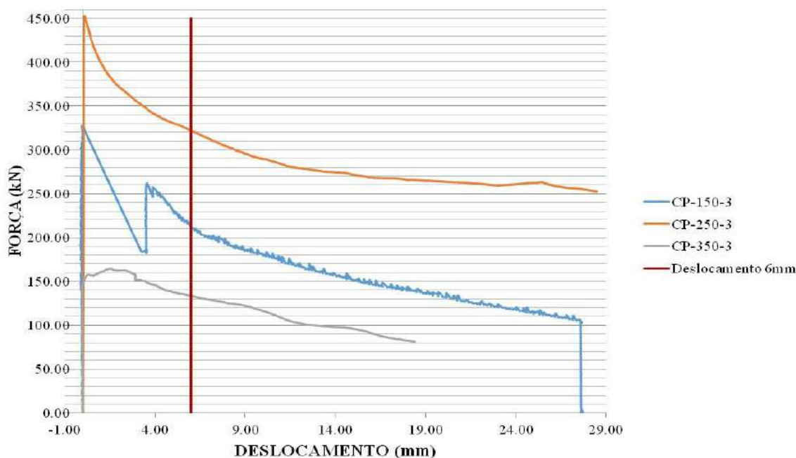
Figura 7 - Força versus Deslizamento perfis de seção retangular.
