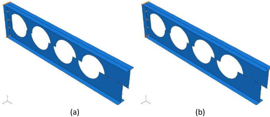
Figura 14 - Indicação das condições de contorno na (a) análise de encurvamento e na (b) análise de carregamento.
