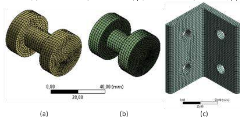
Figura 11 – Malhas: (a) Parafuso de comprimento 2.1/4"; (b) Parafuso de comprimento 2"; (c) Cantoneira.
