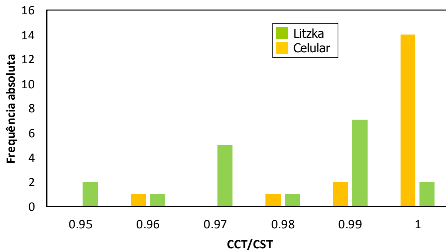
Figura 24 - Relações entre cargas máximas para modelos com tensão (CCT) e sem tensão (CST).
