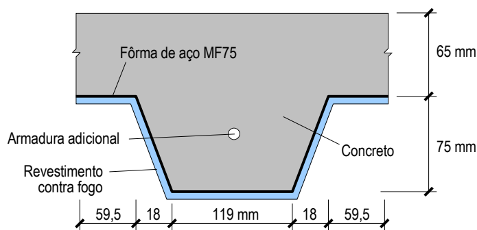
Figura 2 - Dimensões da laje MF-75
