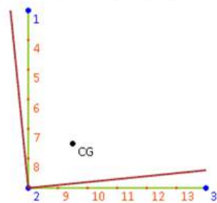
Figura 19 — Resultados para análise numérica via GBTUL para cantoneira L60x60x2.38x970 – Determinação da carga crítica de flambagem elástica e respectivo modo de falha. Torção 96,11% e Flexão 3,88%
