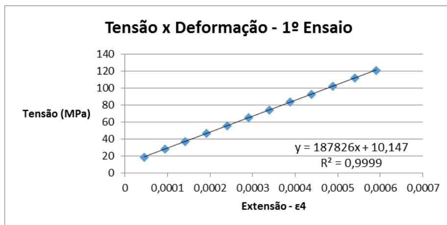
Figura 10 –Valores tensão vs deformação – 1º ensaio.
