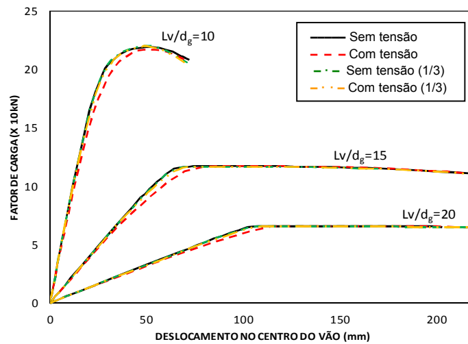
Figura 22 - Curvas de resistência para o perfil W 410x85,0, padrão Litzka.
