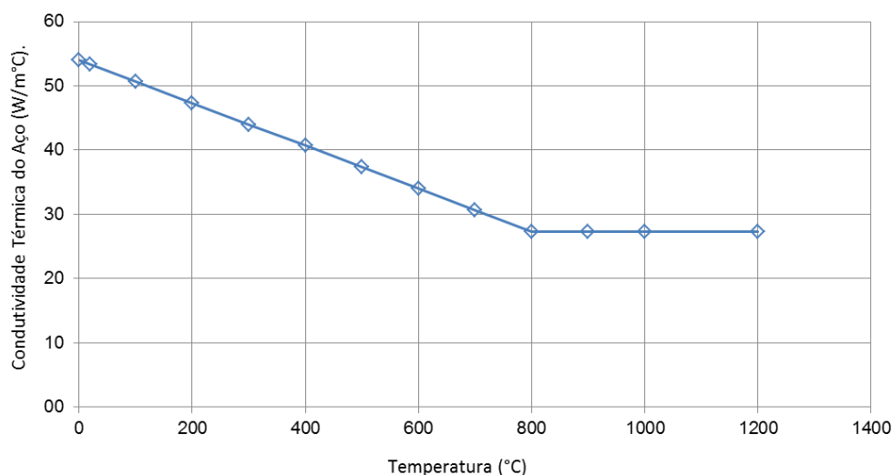
Figura 7: Condutividade Térmica do Aço.
