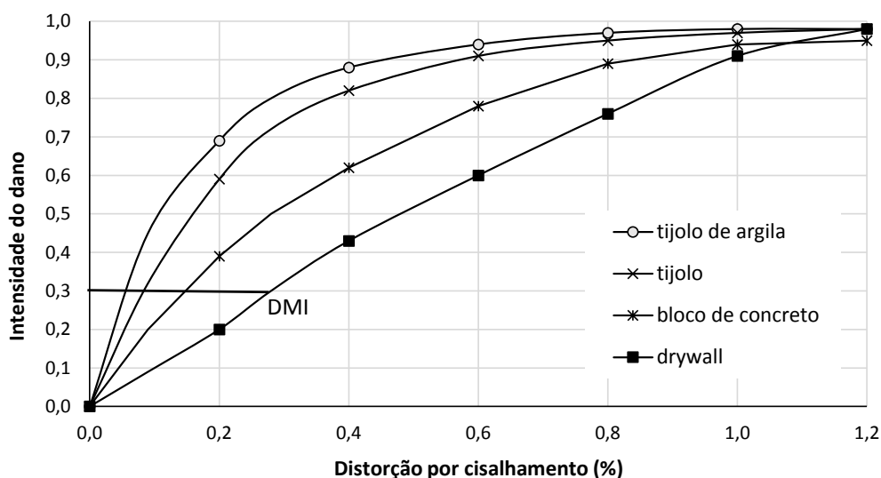
Figura 4. Limiar de dano para diferentes materiais (adaptado de Griffis, 1993).
