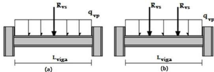
Figura 4 – Vigas principais dos sistemas (a) 2M e (b) 3M. (Fonte: elaborada pelos autores).
