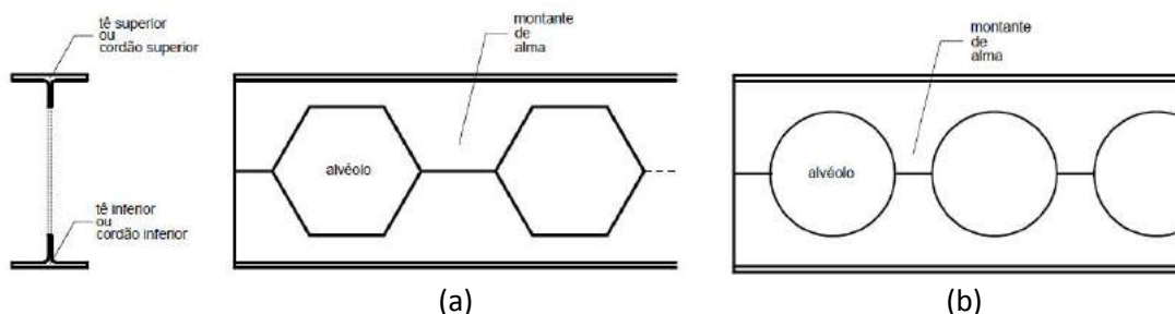
Figura 5 - (a) Viga castelada com aberturas hexagonais e (b) viga celular (fonte: Silveira [2]).
