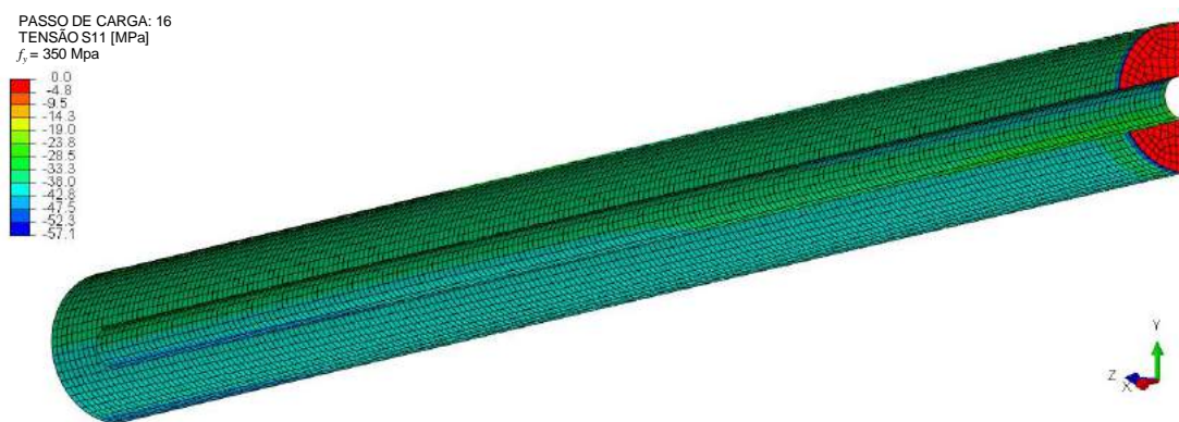
Figura 13 – Modelo 17 sem travamentos – Tensões atuantes – Passo de carga 16 ( \lambda_0 = 1,07 e \lambda = 80 )
