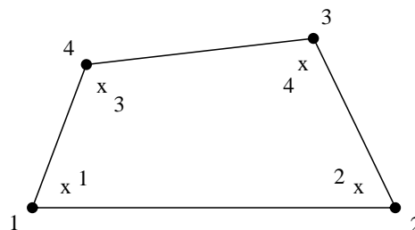
Figura 4: Representação elemento de casca S4
