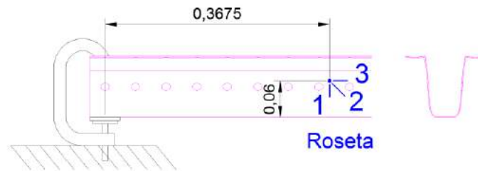
Figura 2 – Roseta de extensômetros (dimensões em metros).
