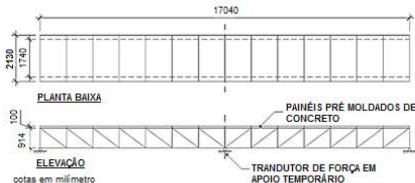
Figura 6 - Plataforma de força utilizada por Rainer, Pernica e Allen [12].
