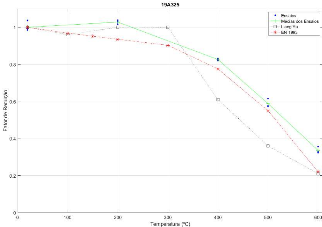
Figura 7 - Gráfico Carregamento de Ruptura x Temperatura comparado com o EN 1993-1-2: 2005 e Liang Yu (2006)
