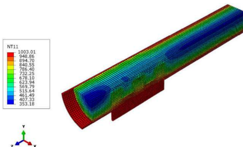
Figura 15: Modelo Numérico da Transferência de Calor no Pilar Misto com o uso do Conector Crestbond
