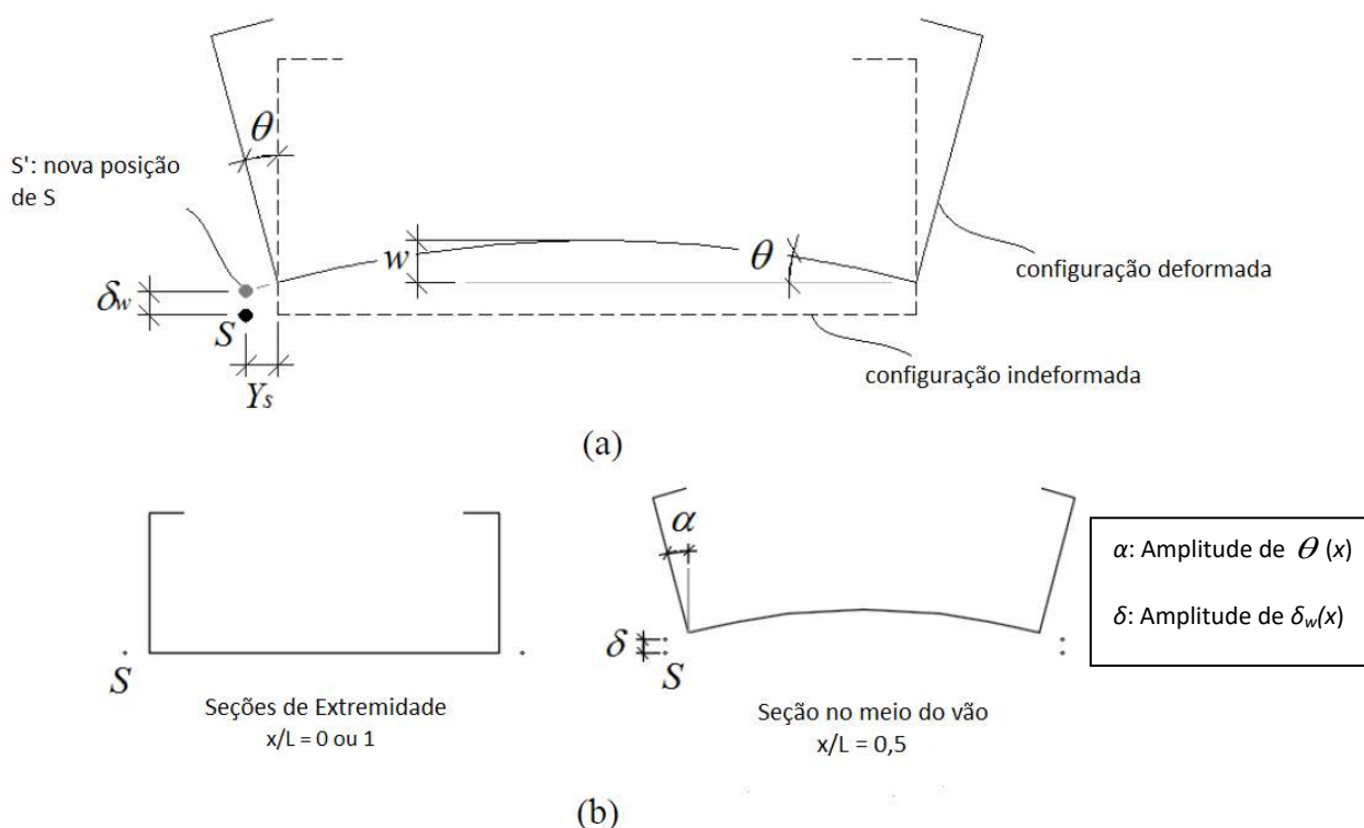
Figura 3: (a) Deformações do modo distorcional (b) configurações deformadas das seções extremas e central.
