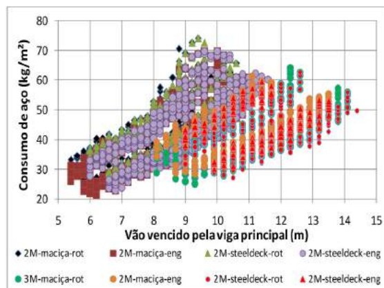
Figura 14 - Consumo de aço dos perfis das vigas em aço AR345. (Fonte: elaborada pelos autores)
