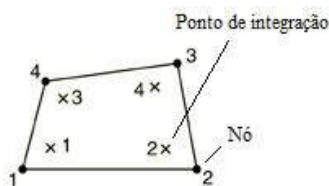
Figura 16 - Elemento quadrilátero S4 (fonte: adaptado de SIMULIA [13]).
