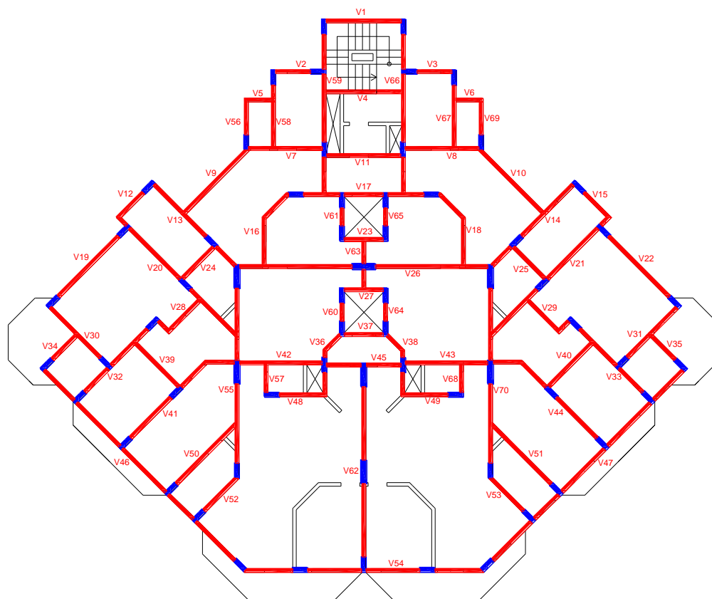
Figura 11: Localização das vigas – Residencial San Marcos.
