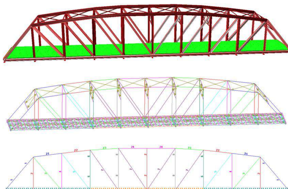
Figura 10 – Modelo computacional de análise da ponte
