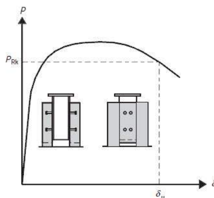
Figura 9 - Determinação da capacidade de deslizamento Du . EN 1994-1-1:2004 [6].
