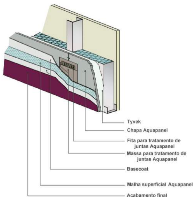
Figura 3: Tratamento de juntas da Knauf Fonte: Criado pelos autores baseado em material gráfico da Knauf
