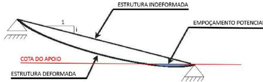
Figura 03 – Potencial ao empoçamento em coberturas com medianas inclinações.
