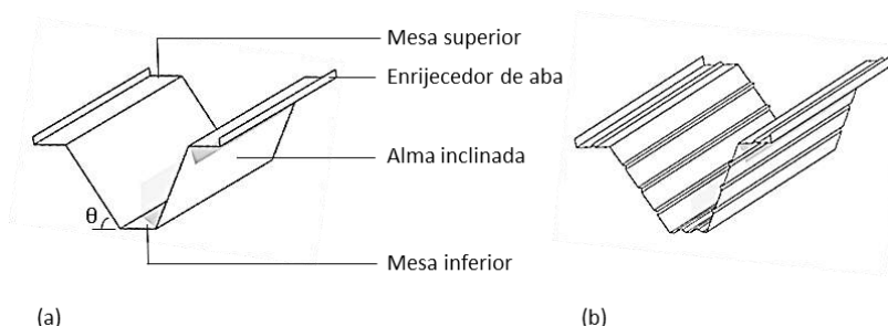
Figura 2: Seções de vigas de aço formadas a frio: (a) sem enrijecedores intermediários e (b) com enrijecedores intermediários.
