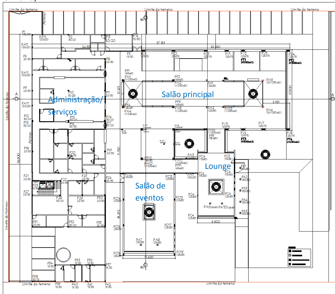
Figura 26 – Planta de pilares na arquitetura do térreo (restaurante NN, pilares de aço em vermelho)
