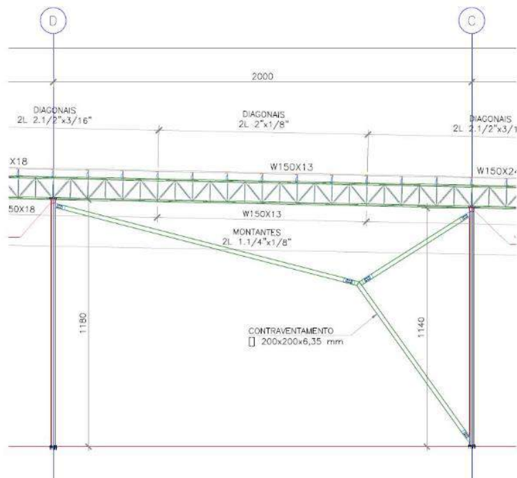
Figura 16 – Sistema da junta de dilatação existente no modelo.
