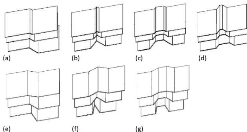
Figura 4: Propriedades acidentais de enrijecedores com duas, três e quatro dobras: variação da largura da parede dos elementos (a-d); ângulo entre elementos de placa (e-g).
