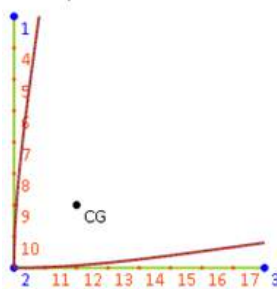
Figura 21 — Resultados para análise numérica via GBTUL para cantoneira L60x60x2.38x1685 – Determinação da carga crítica de flambagem elástica e respectivo modo de falha. Flambagem por flexão em torno do eixo de menor inercia 99,81%.
