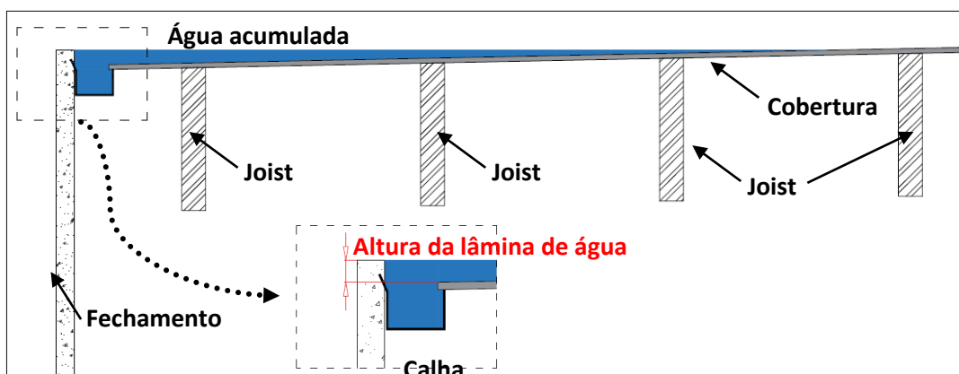
Figura 15 – Configuração de acúmulo de água para cobertura de baixa inclinação.
