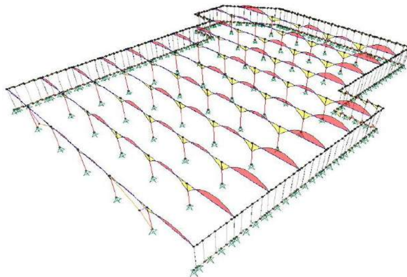
Figura 14 – Imagem do modelo de análise, mostrando a inexistência de momento fletor nos pilares centrais.
