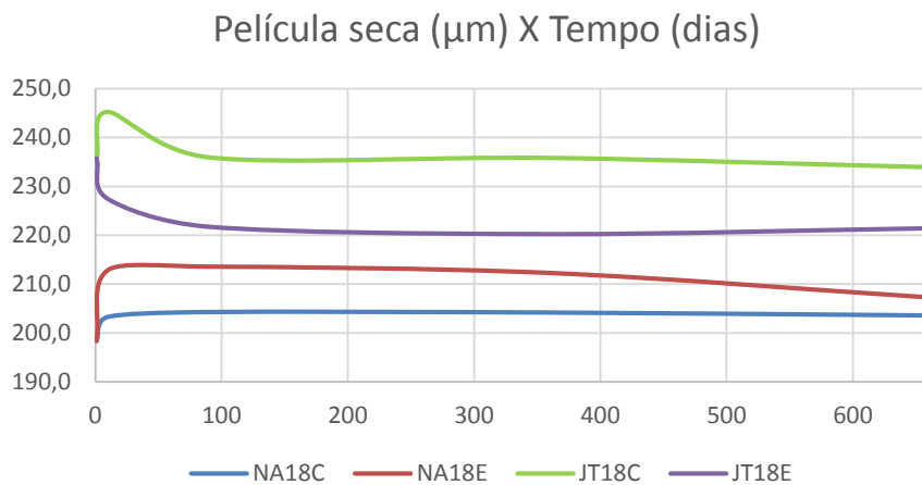
Figura 36: Comparativo gráfico entre corpos de prova com a mesma camada de película seca ( 180\mu\text{m} )
