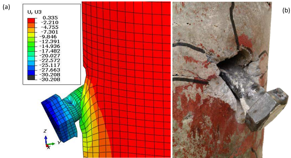
Figura 14- Deslocamentos U3 – eixo z: (a) modelo numérico; (b) modelo experimental;
