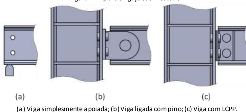
Figura 2 – Apoio e ligações em estudo.
