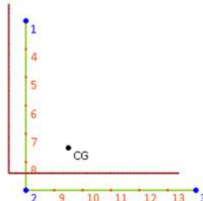
Figura 19 — Resultados para análise numérica via GBTUL para cantoneira L60x60x2.38x970 – Determinação da carga crítica de flambagem elástica e respectivo modo de falha. Torção 96,11% e Flexão 3,88%
