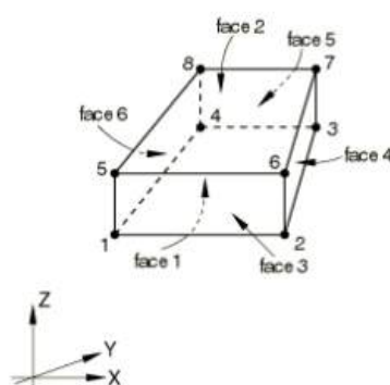
Figura 3: Elemento Sólido DC3D8.
