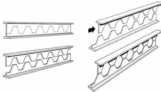
Figura 1 - Processo de obtenção de vigas alveolares com abertura hexagonal (fonte: Grünbauer [1]).
