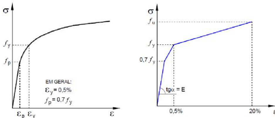
Figura 22 – Modelos constitutivos (Fonte: [6]).
