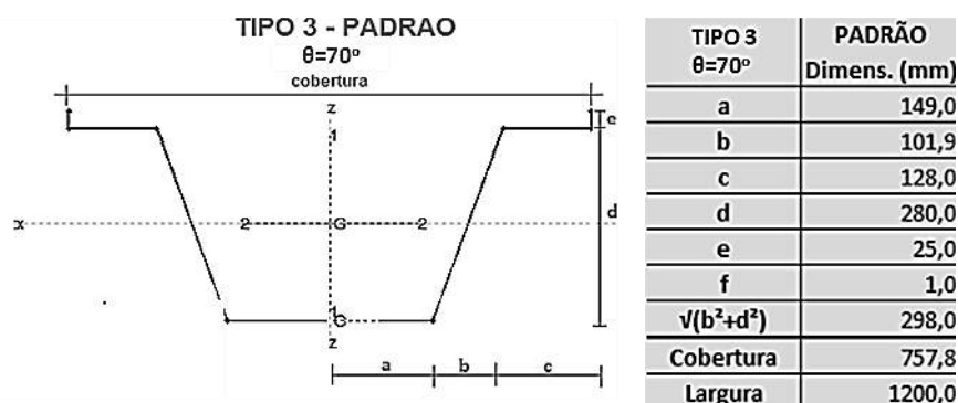
Figura 19: Parâmetros geométricos de viga-calha sem enrijecedores e \theta = 70^\circ .
