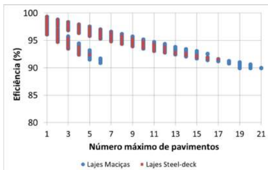
Figura 31 - Relação entre número de pavimentos da torre e a eficiência para aço MR250. (Fonte: elaborada pelos autores)
