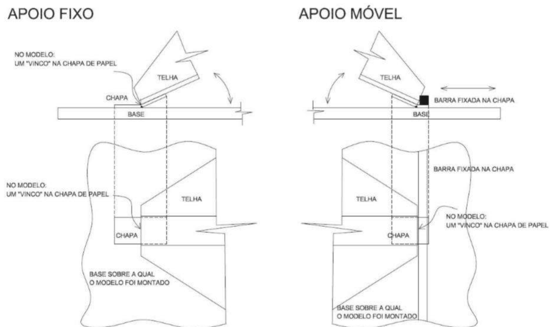
Figura 14 – Alternativa para os apoios (DIAS, 2015).
