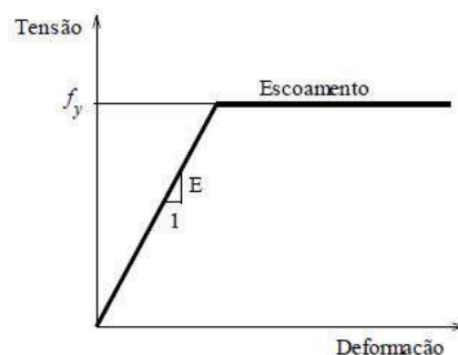
Figura 13 - Relação tensão x deformação para o material elástico perfeitamente plástico.
