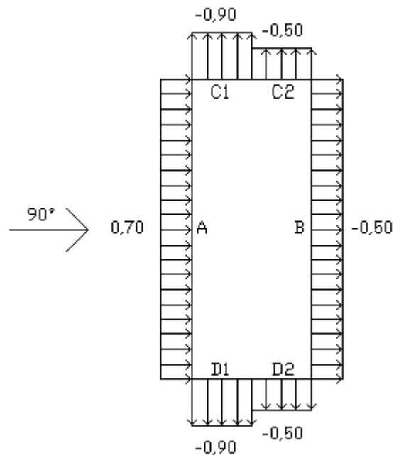
Figura 11 - Coeficiente de pressão externa nas paredes com vento a 90^\circ . Fonte: VisualVentos
