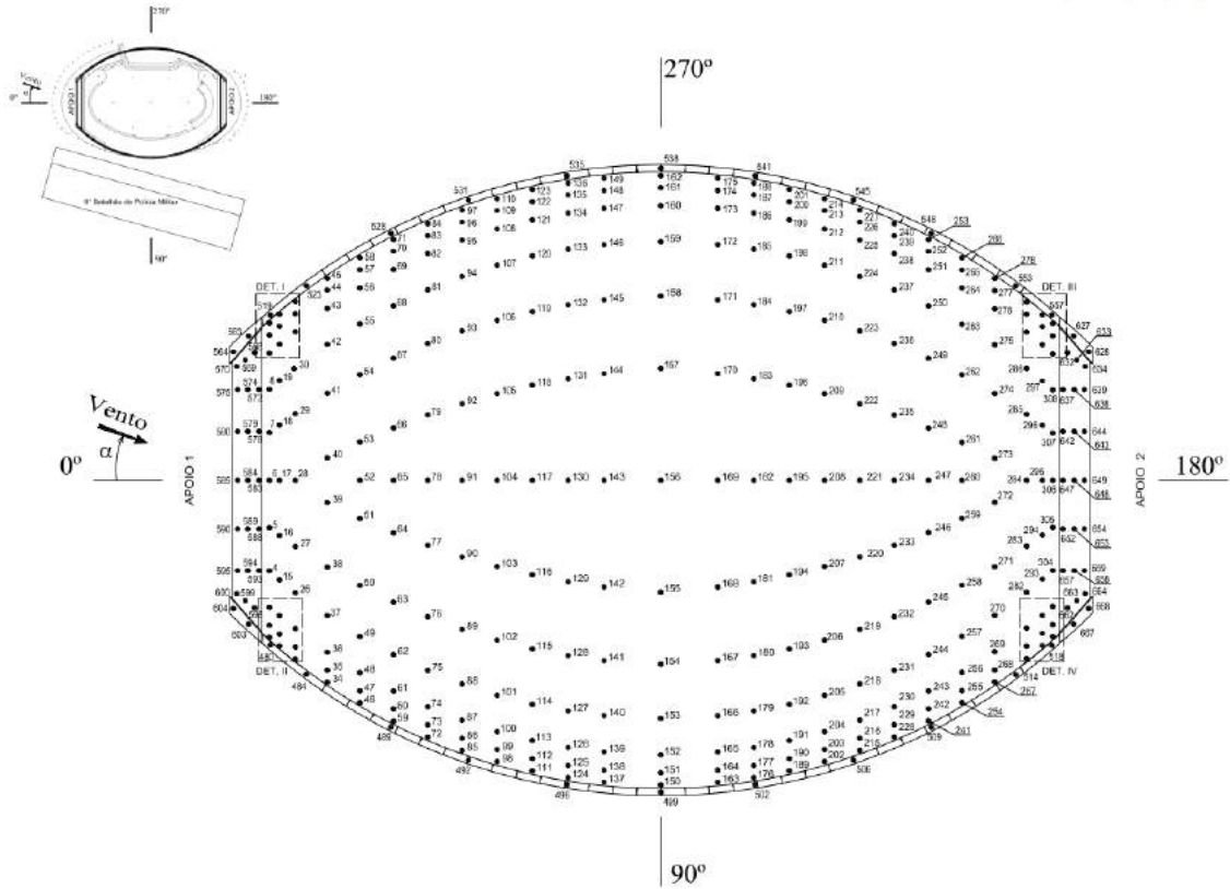
Figura 3 – Distribuição das tomadas de pressão na face superior da cobertura.
