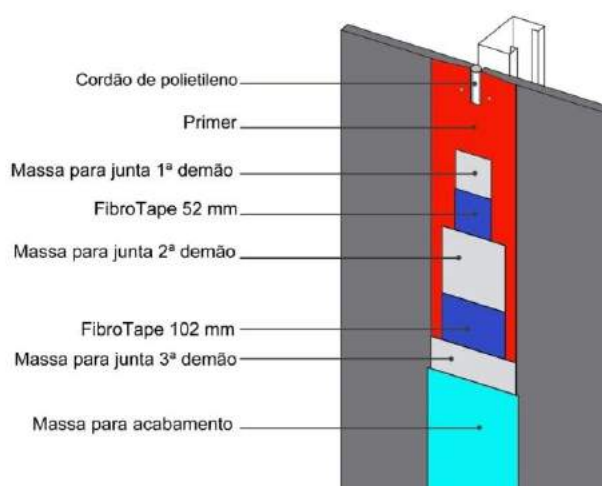
Figura 1 - Tratamento de juntas Brasilit
