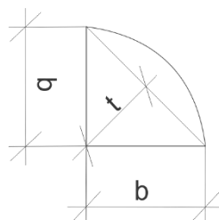
Figura 17 – Dimensões da solda
