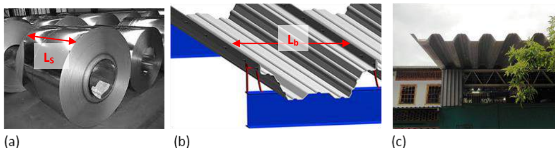
Figura 1: (a) Bobinas de aço, (b) vigas-calha em aço conformadas a frio e (c) sistema estrutural para coberturas de grandes vãos
