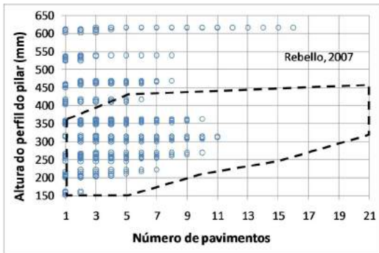
Figura 19 - Relação do número de pavimentos e perfis do pilar em aço MR250 e laje steel-deck. (Fonte: elaborada pelos autores)
