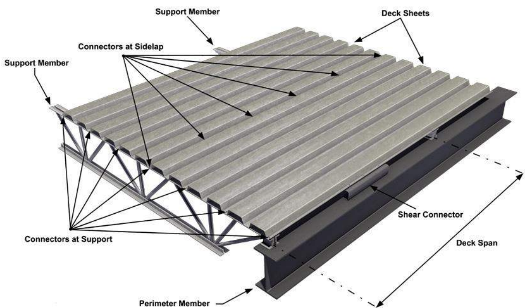
Figura 01 – Módulo do sistema Roof Deck e seus componentes.
