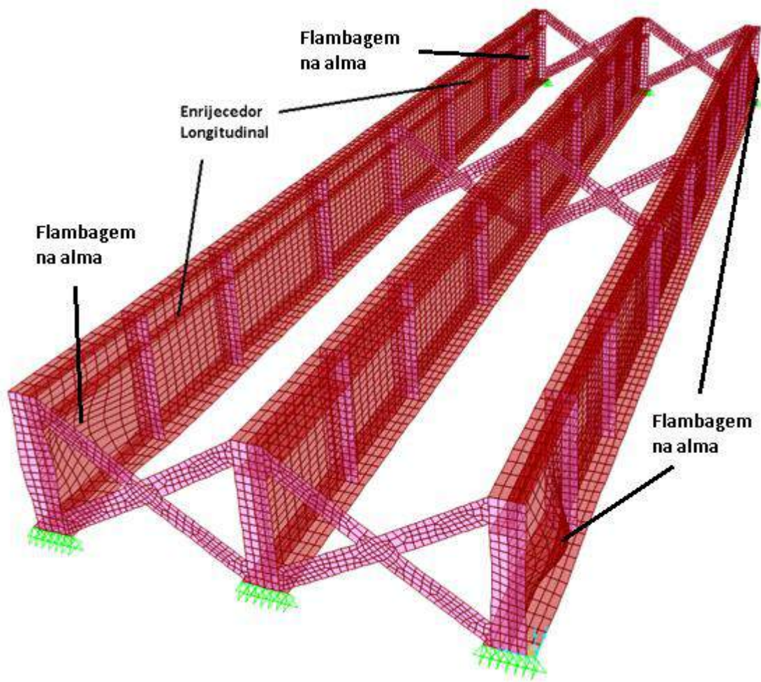
Figura 11: Enrijecedores longitudinais
