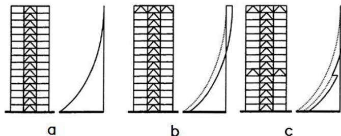
Figura 4 – Diferenças entre diagramas de momento fletor entre edifícios sem e com treliças horizontais Fonte: Bayati; Mahdikhani e Rahaei [20].
