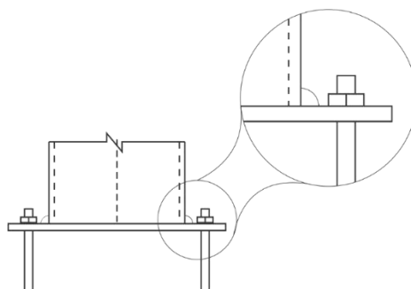
Figura 16 – Detalhe da solda tipo filete
