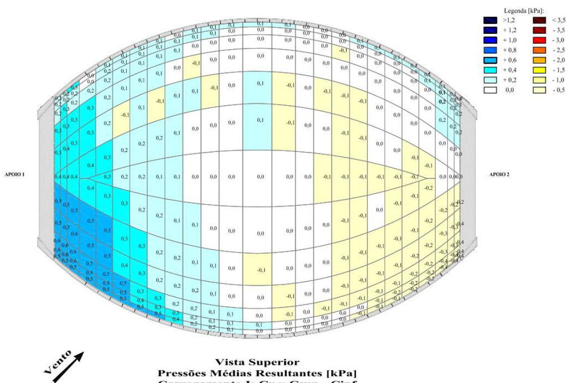
Figura 9 – Carregamento I para ângulo 45°.
