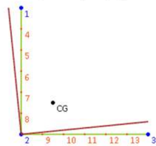
Figura 18 — Resultados para análise numérica via GBTUL para cantoneira L60 \times 60 \times 2,38 \times 615 — Determinação da carga crítica de flambagem elástica e respectivo modo de falha. Torção 98,49% e Flexão 1,47%.
