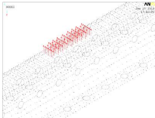
Figura 25 – Modelação da região de carregamento.
