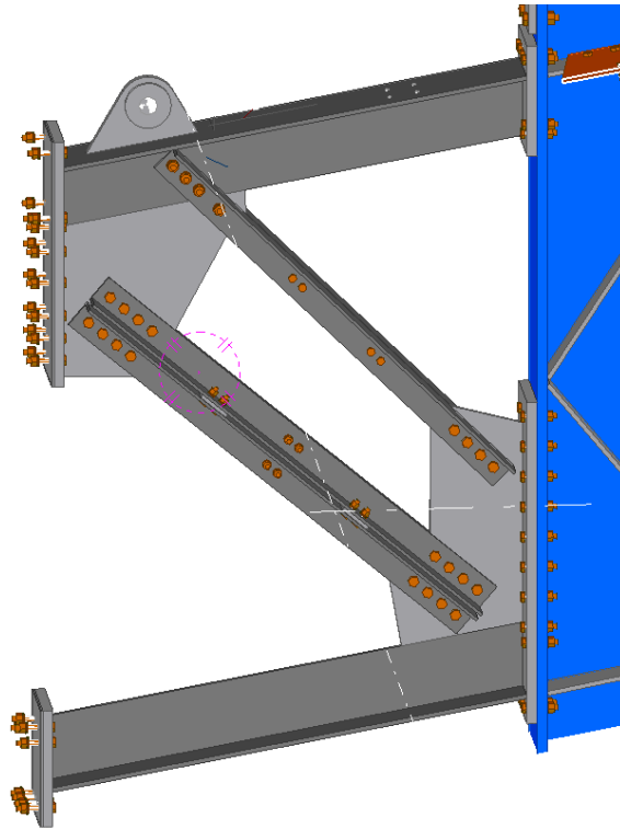
Figura 18. Ménsulas segundo izado.
