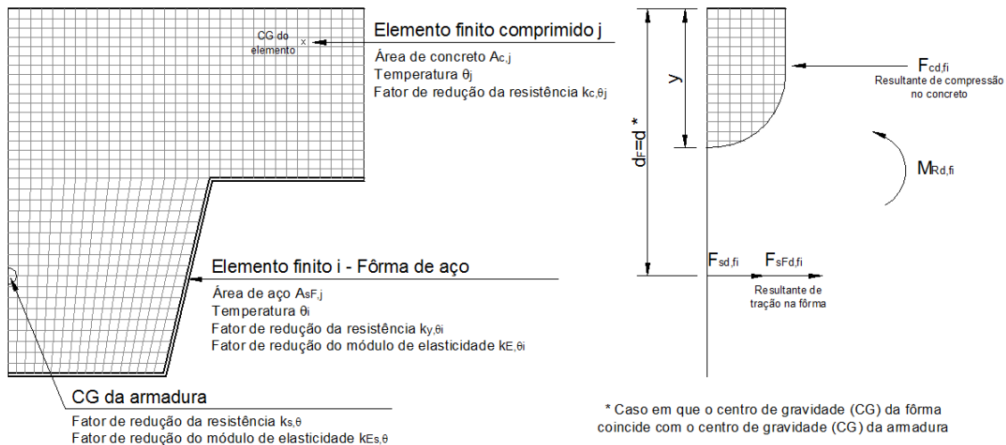
Figura 1 - Seção da laje mista discretizada com malha de elementos finitos
