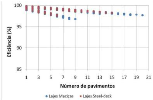
Figura 24 - Eficiência dos pilares de perfis em aço AR345. (Fonte: elaborada pelos autores)
