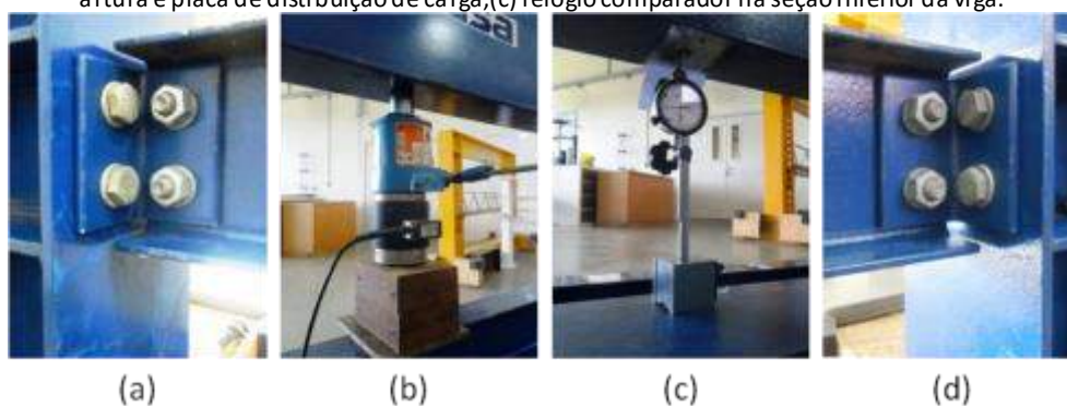
Figura 7 – Ensaio de viga com LCPP. (a, d) LCPPs; (b) macaco hidráulico, célula de carga, placas de compensação de altura e placa de distribuição de carga; (c) relógio comparador na seção inferior da viga.
