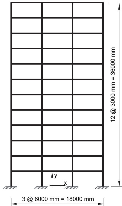
Figura 5 – Esquema estrutural do modelo estudado.
