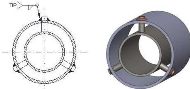
Figura 6 – Travamentos deslizantes
