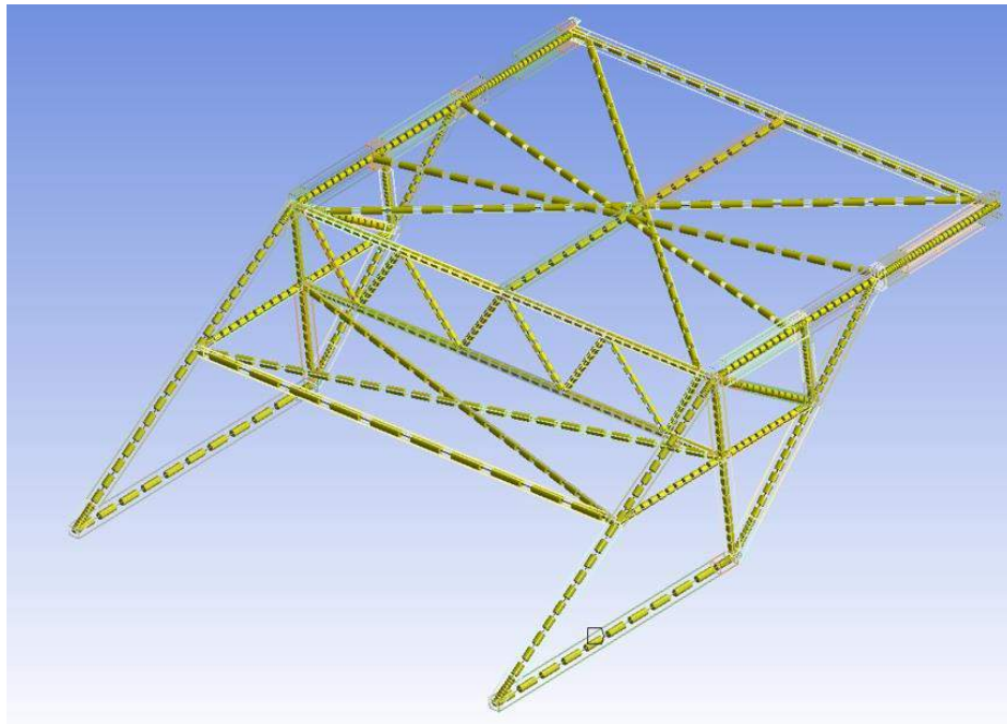
Figura 6 – Malha de elementos finitos da treliça içadora de aduelas.
