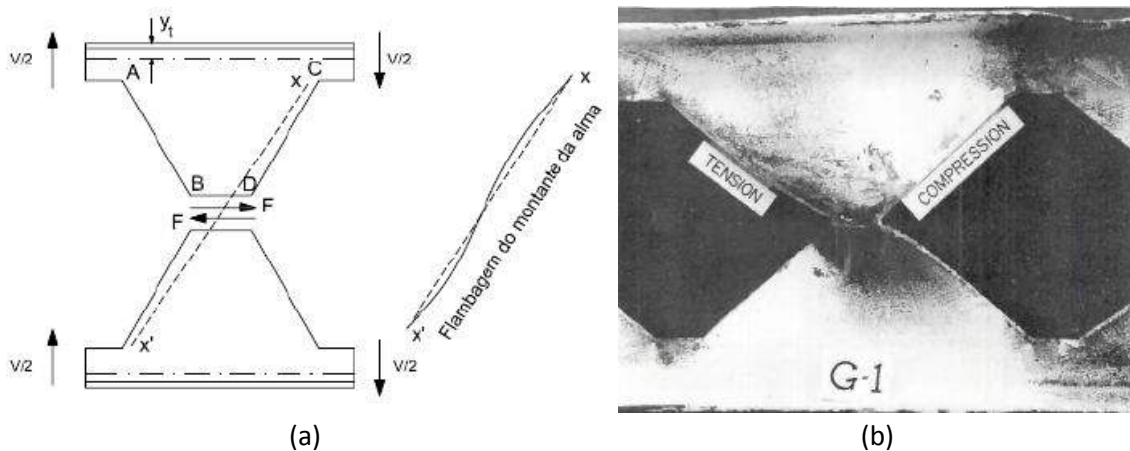
Figura 9 - (a) Mecanismo de flambagem (fonte: Kerdal e Nethercot [10]). (b) Flambagem do montante de alma de uma viga castelada (fonte: Hosain e Speirs [9]).
