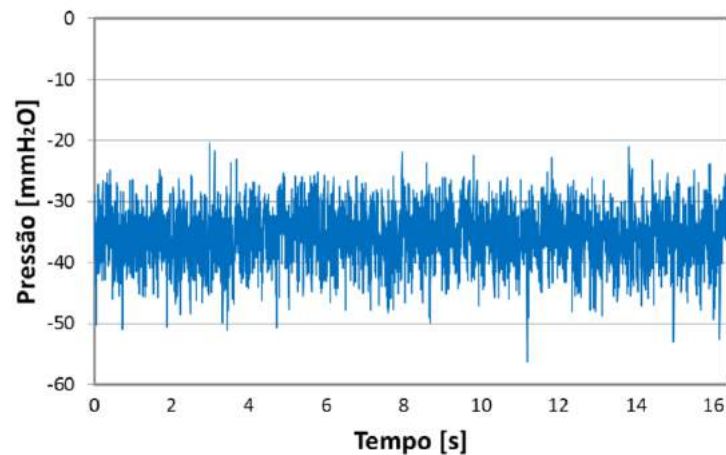
Figura 6 – Registro da variação de pressão ao longo do tempo para a tomada 300 e ângulo de incidência do vento a 330° (vento com expoente p=0,11 ).
