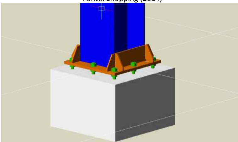
Figura 11 – Ligações: parafusos A325, 19mm Fonte: Shopping (2014)
