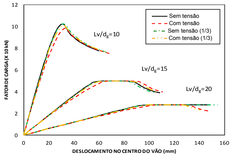
Figura 18 - Curvas de resistência para o perfil W 410x38,8, padrão Litzka.
