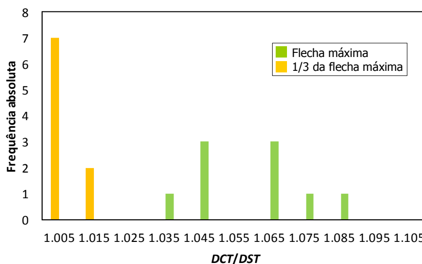
Figura 25 - Relações entre deslocamentos no centro do vão para modelos com tensão (DCT) e sem tensão (DST) para padrão Litzka.
