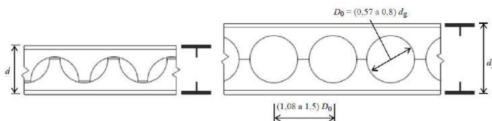
Figura 7 - Geometria de vigas celulares (fonte: Silveira [2]).
