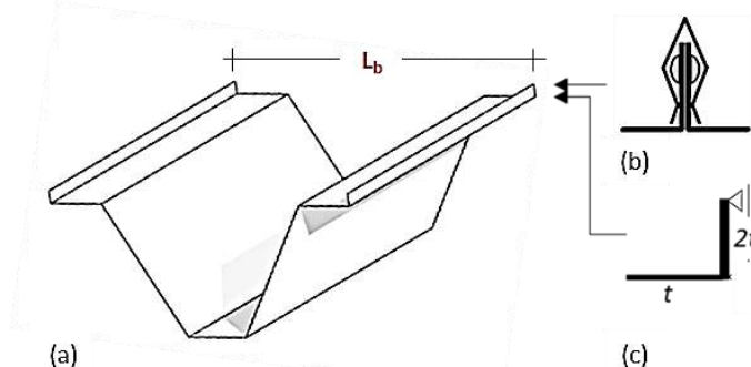
Figura 5: (a) viga calha sem enrijecedores; (b) conectores de aba típicos entre vigas-calha adjacentes e (c) condição de apoio admitida na análise de estabilidade elástica.
