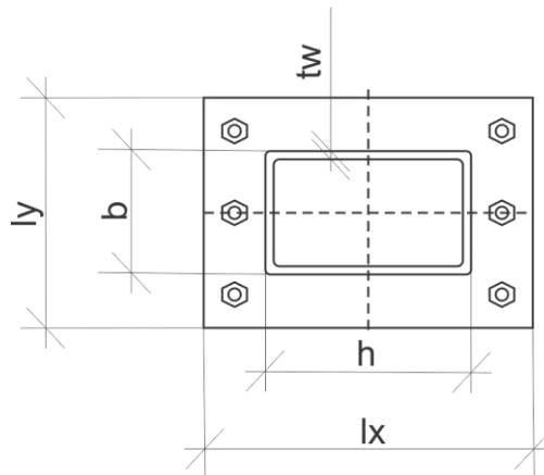
Figura 01 – Base retangular para pilar metálico de seção retangular
