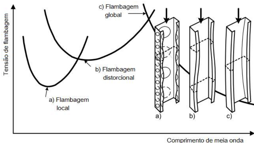
Figura 3 — Exemplos de modos de flambagem: a) local; b) distorcional; c) global
