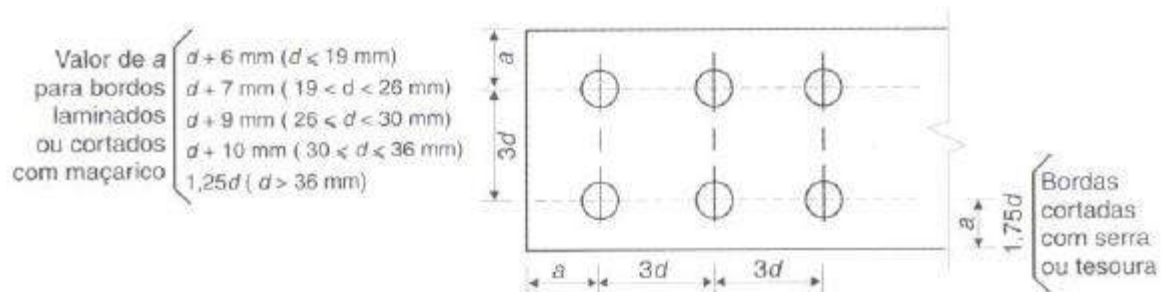
Figura 16 – Espaçamentos construtivos mínimos recomendados para conectores (Fonte: Pfeil, 2008)
