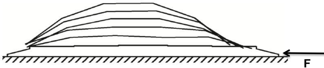
Figura 3 – Ilustração da cinemática do movimento gerado pela aplicação de uma força horizontal (F) na base da cobertura, gerando sua curvatura até a forma final desejada.
