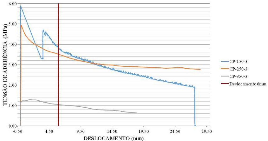
Figura 8 - Tensão de aderência versus deslocamento dos corpos de prova com seção o retangular.
