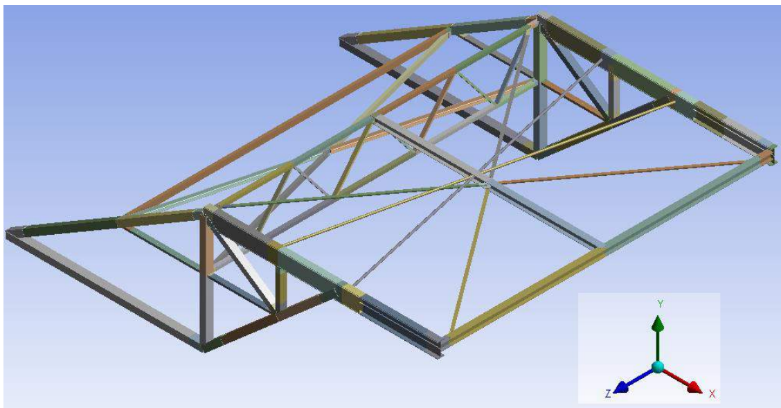
Figura 5 – Modelo geométrico da treliça içadora de aduelas.
