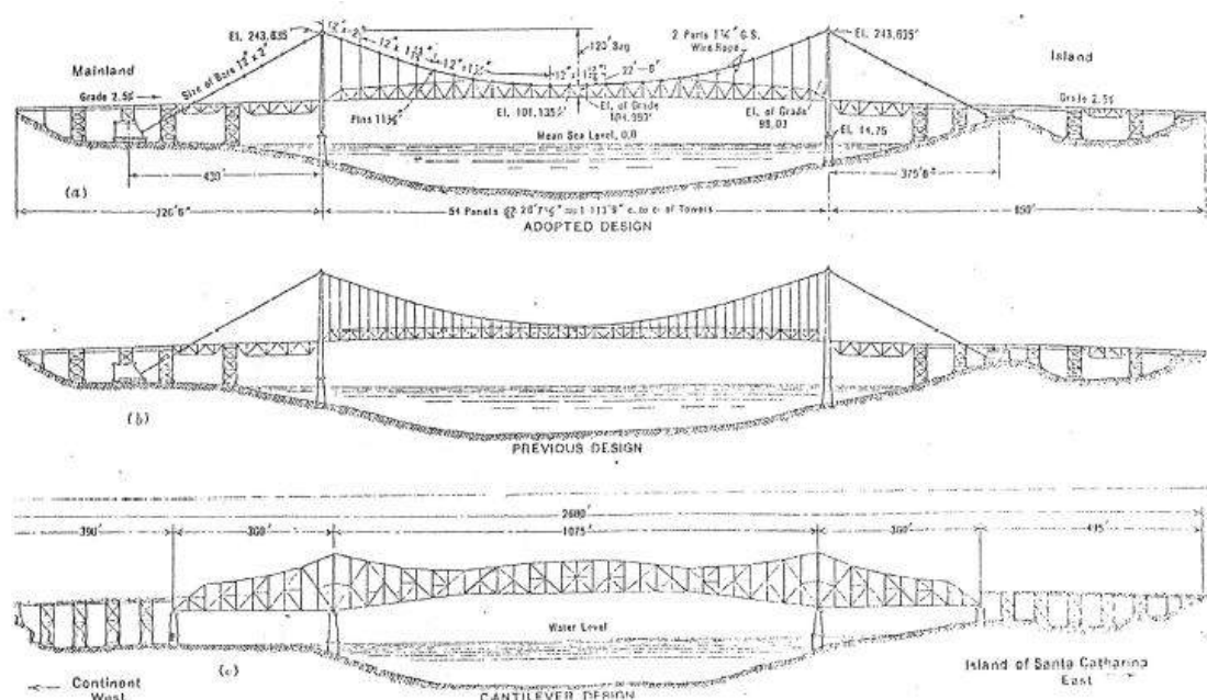
Figura 2: Soluções estruturais avaliadas pelos projetistas originais (Steinman, 1926).
