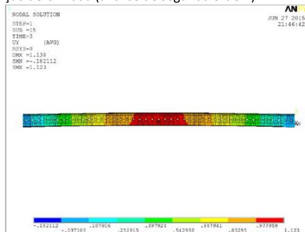
Figura 28 – Deslocamentos verticais – análise não linear de 2ª ordem (medidas em cm).
