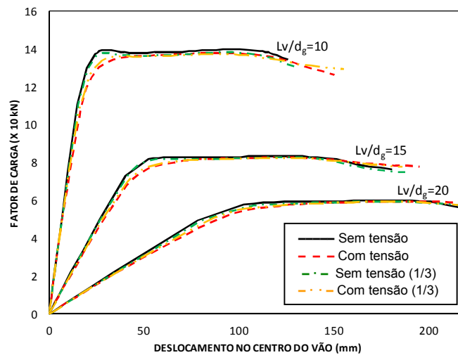
Figura 23 - Curvas de resistência para o perfil W 410x85,0, padrão celular.
