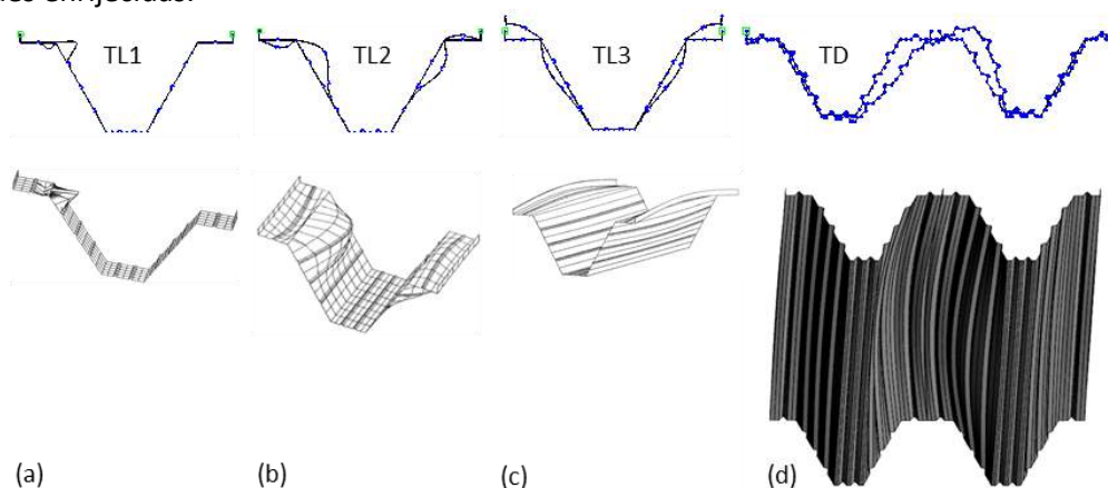
Figura 6: Modos de flambagem elástica para vigas calhas com mesa superior comprimida: (a-c) modos locais e (d) modo distorcional.
