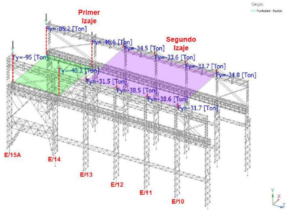
Figura 24. Esfuerzos aplicados en estructura de la nave de aceria debido al primer y segundo izaje de la campana de extracción.
