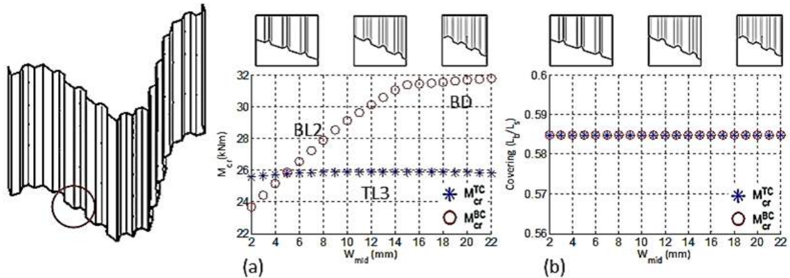
Figura 15: Tendências resultantes da variação da largura da parede intermediária de enrijecedores trapezoidais na alma ( 45^\circ , w_{incl3} = 17 mm): (a) momentos críticos associados à compressão da mesa superior e inferior e (b) taxa de cobrimento.
