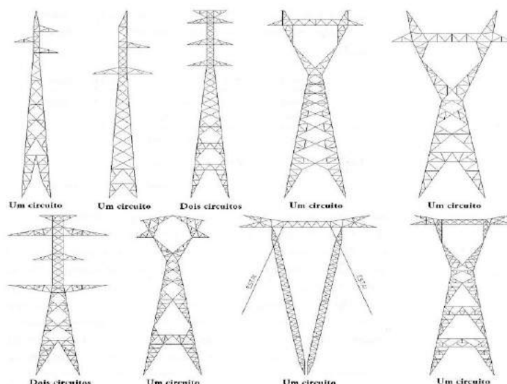
Figura 1 – Configurações de torres para 1 e 2 circuitos (GONTIJO [2], 1994)
