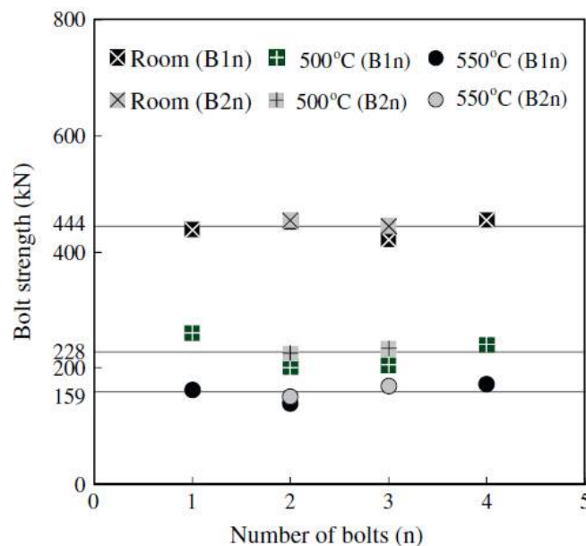
Figura 2 - Resistência média dos parafusos em temperatura ambiente, 500 °C e 550 °C e diferentes disposições da ligação. (Eixo x: Número de parafusos (n), Eixo y: Resistência dos parafusos (kN)). Fonte: Yang et al. (2011).
