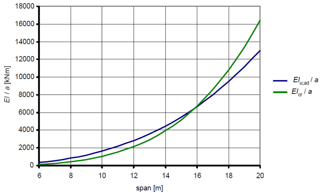
Figura 09 – Gráfico mostrando a relação entre a rigidez crítica ( EI_{cr} ) e a mínima normatizada ( EI_{u,ad} ) em função do vão do elemento.
