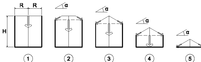
Figura 7 – Transbordamento pelas bordas do costado do silo
