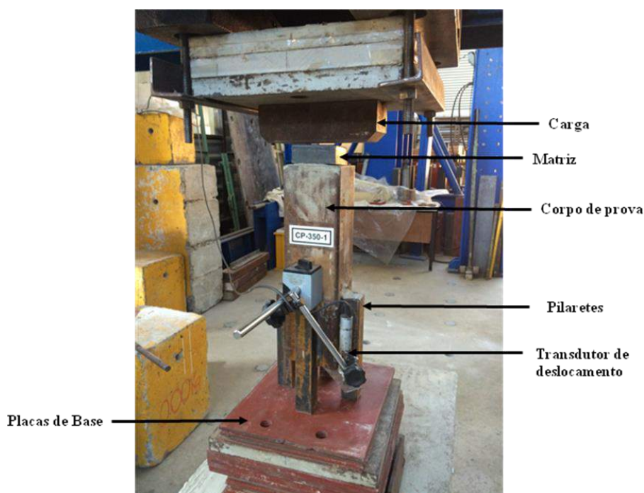
Figura 2 - Esquema ensaio utilizado.
