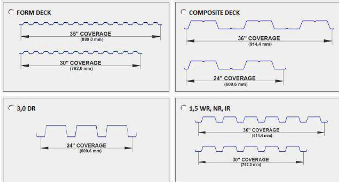
Figura 02 – Tipologias de decks atestadas pelo manual de dimensionamento de diafragmas do SDI.
