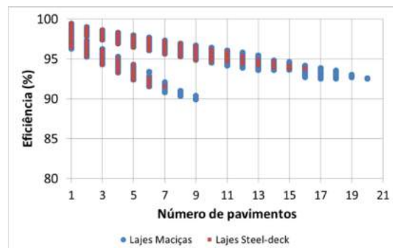
Figura 32 - Relação entre vão da laje e número de da torre e a eficiência para aço AR345. (Fonte: elaborada pelos autores)
