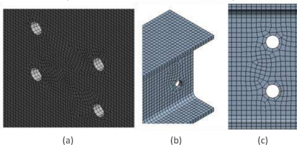
Detalhes: (a) dos furos na coluna; (b, c) da viga.
