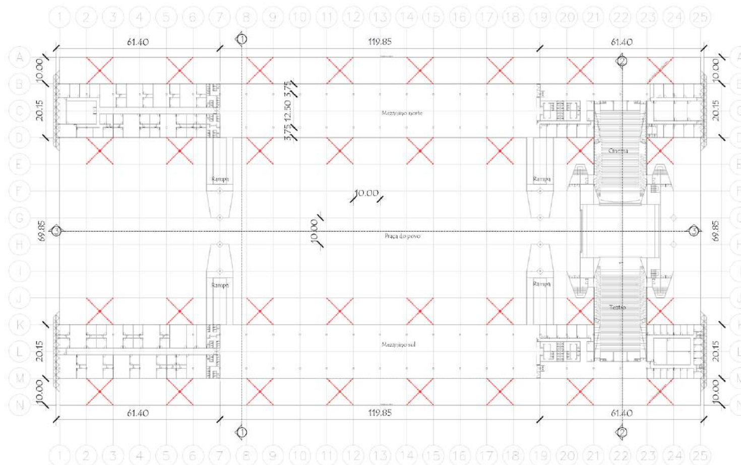
Figura 3 - Planta baixa geral do mezanino do Espaço Cultural (em vermelho estão representados os pilares-árvores de aço)
