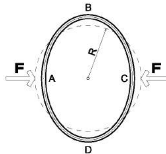
Figura 11 – Esforços internos de flexão provocados num anel
