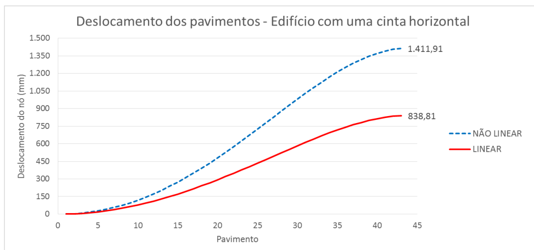
Gráfico 2 - Deslocamentos no edifício com treliças verticais e uma treliça horizontal Fonte: As autoras (2016).
