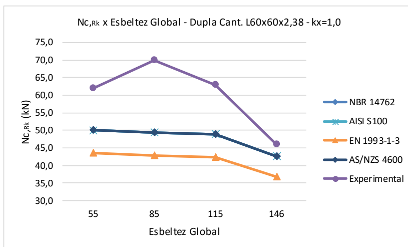
Figura 13 — Resultados analíticos para dupla cantoneira – rótula na direção x - MLE
