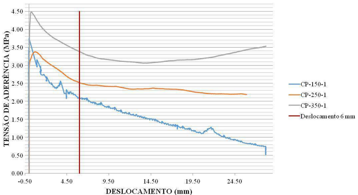
Figura 4 - Tensão de aderência versus deslocamento dos corpos de prova com seção quadrada.
