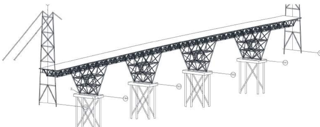
Figura 7: Estrutura inferior auxiliar de sustentação do vão central.
