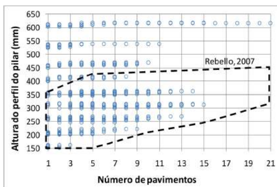
Figura 17 - Relação do número de pavimentos e perfis do pilar em aço MR250 e laje maciça. (Fonte: elaborada pelos autores)
