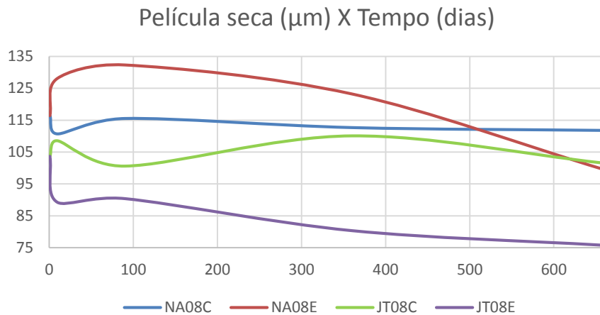
Figura 23: Comparativo gráfico entre corpos de prova com a mesma camada de película seca ( 80\mu\text{m} )
