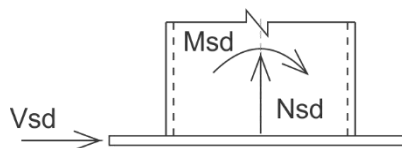
Figura 07 – Solicitações provenientes da estrutura com esforço normal de tração
