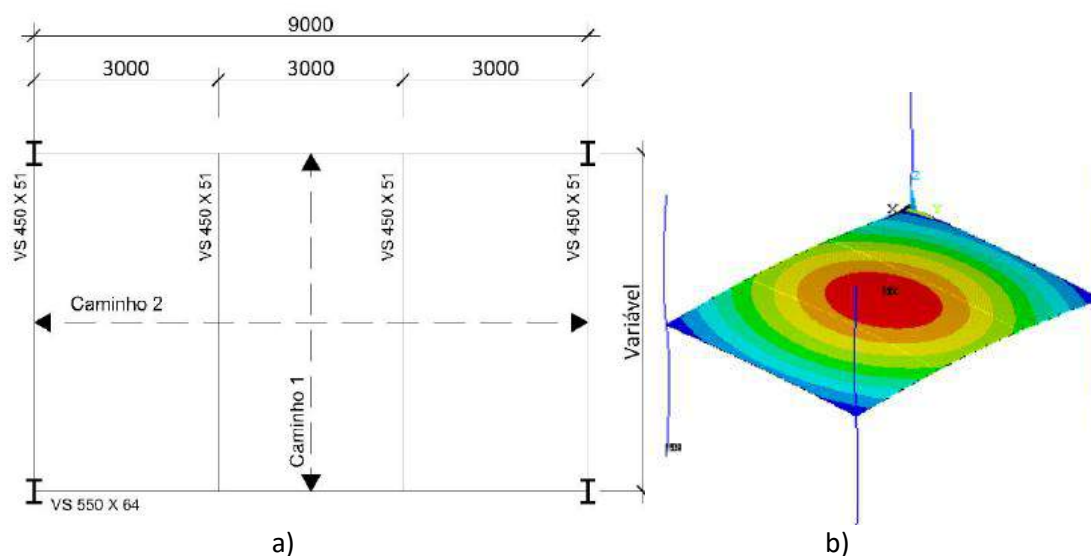
Figura 10 – a) Layout do sistema estrutural estudado por Mello (cotas em milímetros) [8]. b) Modo de vibração associada a primeira frequência natural, f_n = 7,42 Hz [8].
