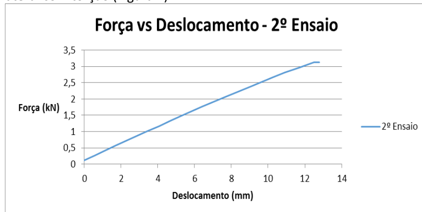
Figura 6 - Força vs Deslocamento obtido pelo transdutor a meio vão – 2º Ensaio.
