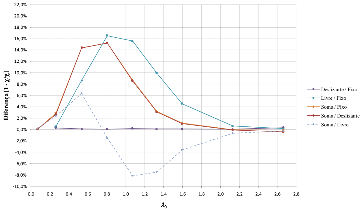
Figura 11 – Diferenças entre forças críticas de compressão
