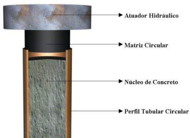
Figura 1 - Esquema do ensaio de deslizamento do pilar misto circular Campolina [4].
