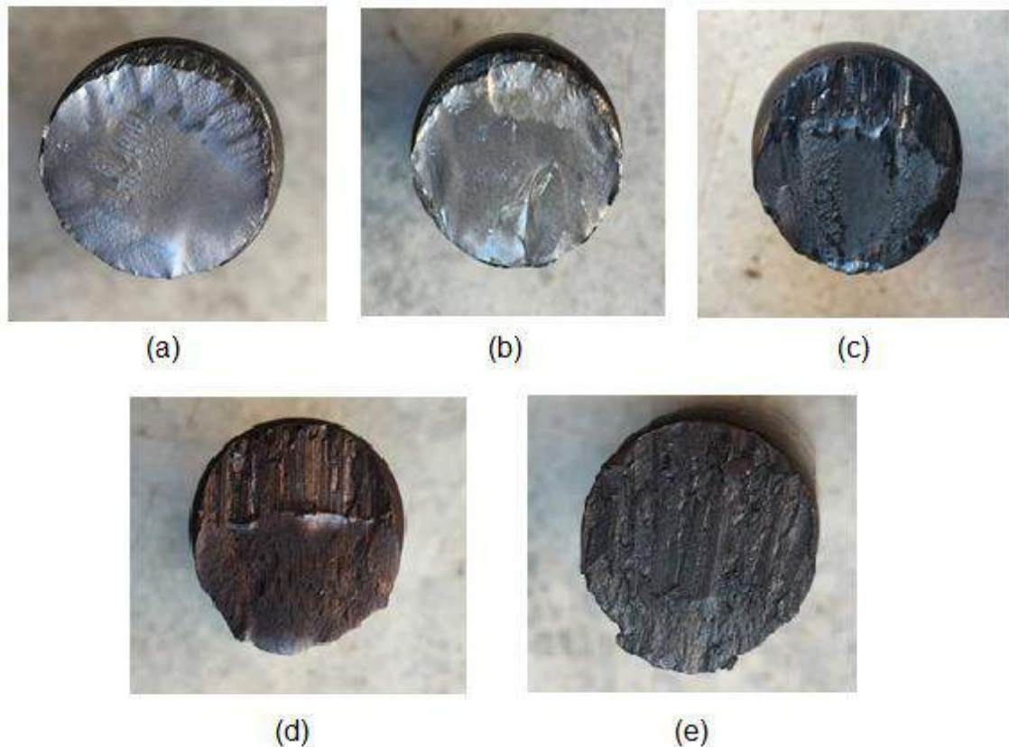
Figura 8 – Fotos dos planos de corte dos parafusos para cada temperatura: (a) Temperatura Ambiente; (b) T = 200 °C; (c) T = 400 °C; (d) T = 500 °C; (e) T = 600 °C
