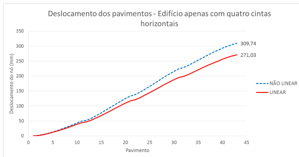
Gráfico 5 - Deslocamentos no edifício com treliças verticais e quatro treliças horizontais Fonte: As autoras (2016).
