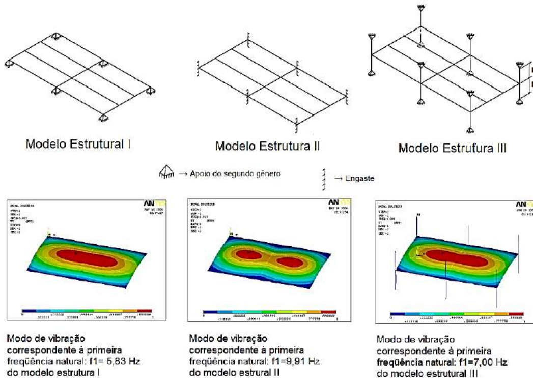
Figura 9 – Modelos estruturais e respectivos modelos de vibração correspondente à frequência natural estudados por Loose (adaptado de [22]).
