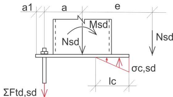
Figura 13 - Situação caso 03 solicitada a esforço de compressão
