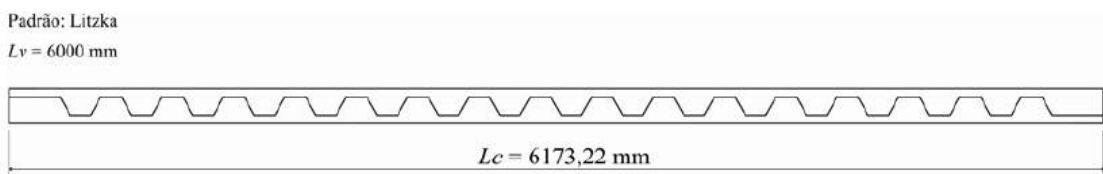
Figura 9 – Comprimento do vão necessário para corte em um vão de 6000 mm (Oliveira [4]).
