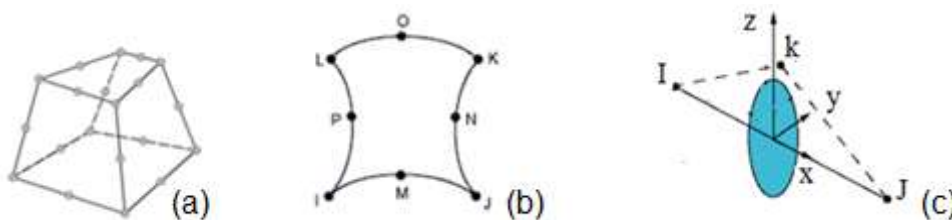
Figura 3 – Elementos utilizados (Fonte: Adaptado de ANSYS, 2015)
