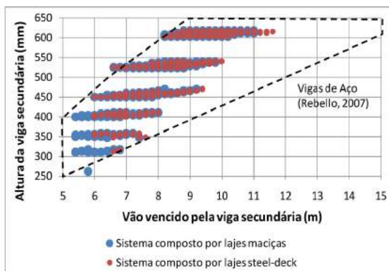
Figura 10 - Relação entre vão e altura da viga secundária em aço AR345. (Fonte: elaborada pelos autores)
