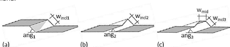
Figura 3: Enrijecedores intermediários: (a) de duas dobras, (b) de três dobras e (c) de quatro dobras.
