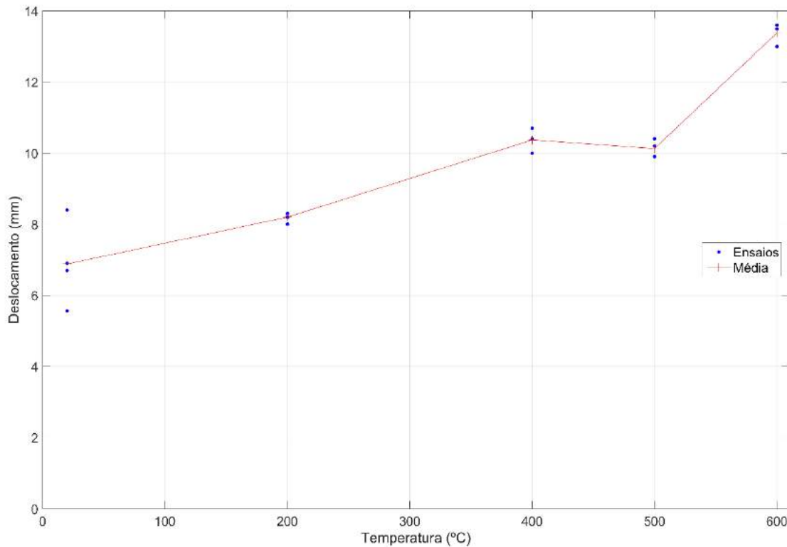
Figura 9 - Gráfico Deslocamento (carregamento máximo) x Temperatura
