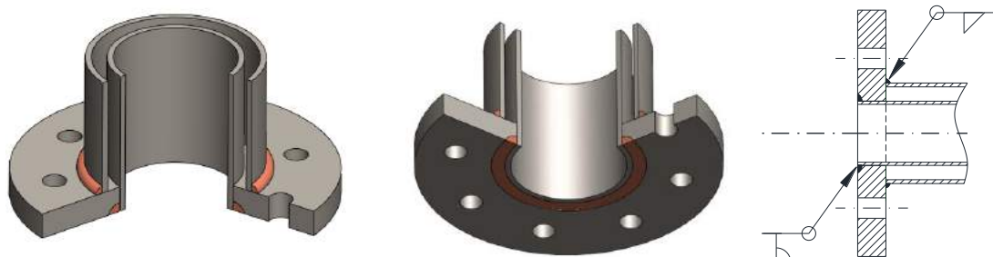
Figura 4 – Ligação do flange
