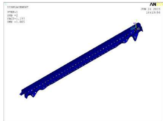
Figura 15 – 2º modo de flambagem (distorcional, \alpha_d=1,197 )
