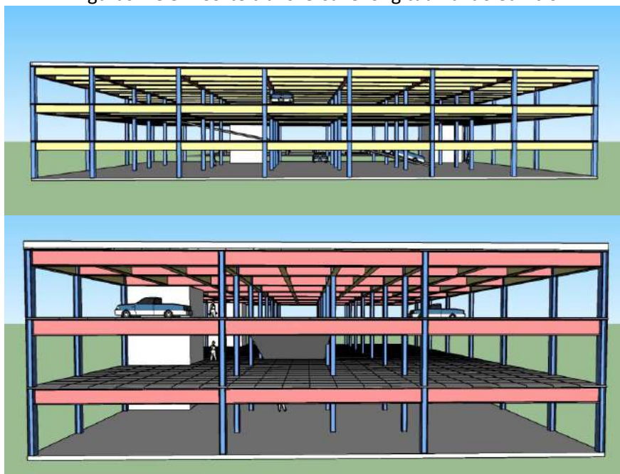
Figuras 7 e 8 – Corte transversal e longitudinal do edifício
