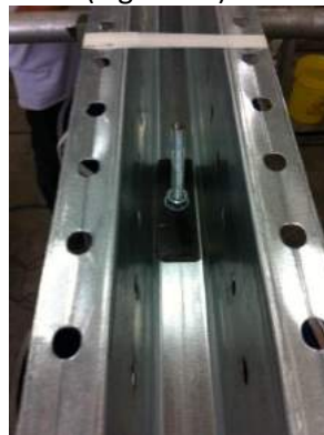
Figura 26 – Chapa de distribuição de carga (Laboratório de Estruturas da UNICAMP).
