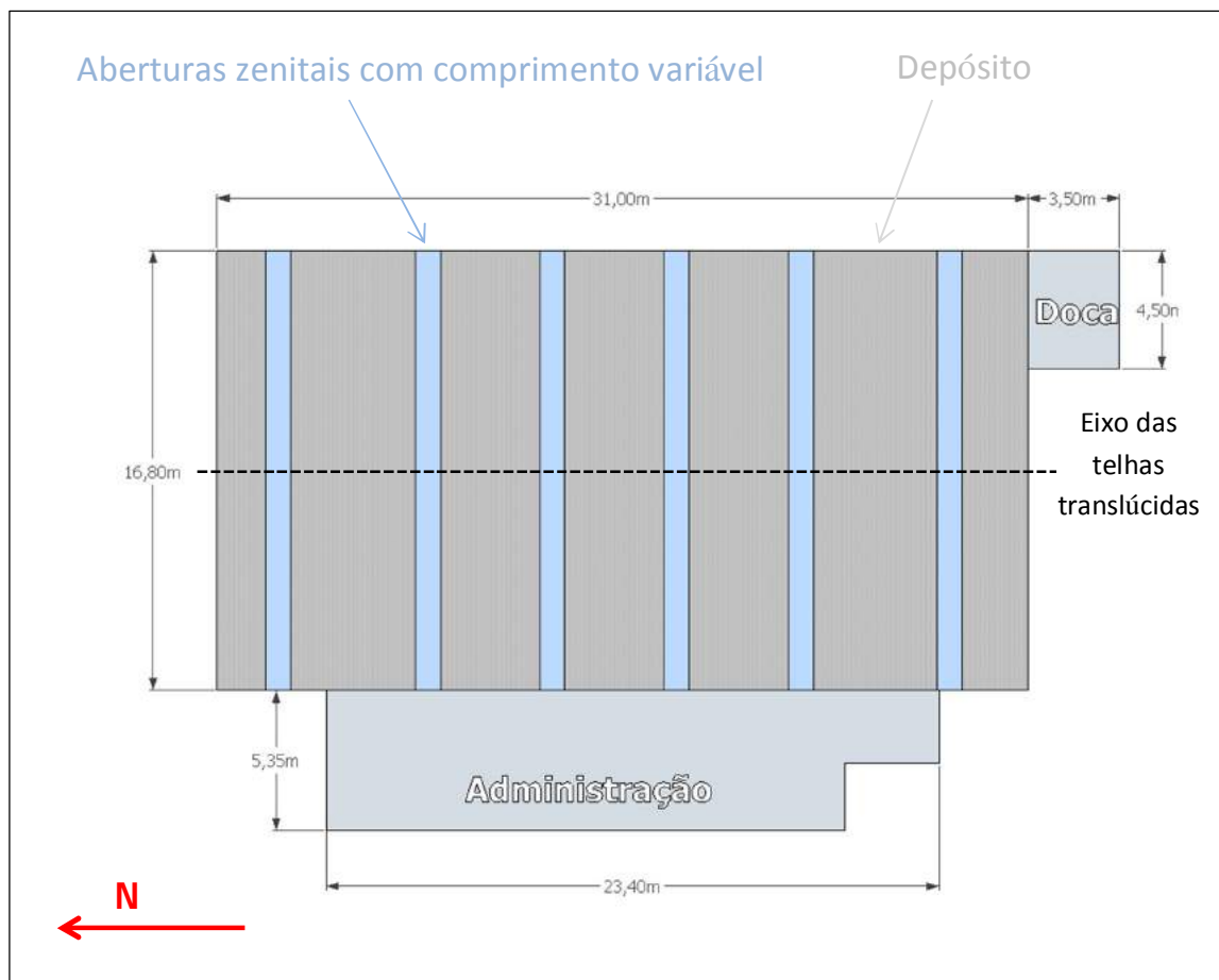
Figura 1: Vista superior da cobertura do galpão com a indicação das aberturas translúcidas com área variável, sem escala.
