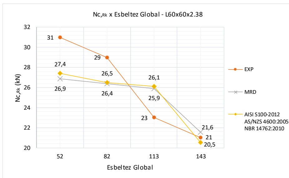
Figura 22 — Resultados analíticos para cantoneira simples – N_{c,Rk} x E.G. - MRD x MLE x EXP
