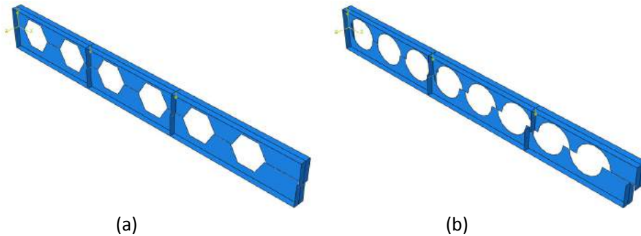
Figura 12 - Indicação das posições de aplicação das cargas para vigas com padrão (a) Litzka e (b) celular.
