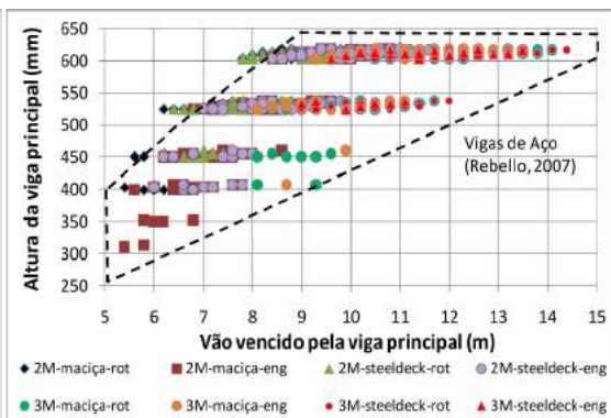
Figura 12 - Relação entre vão e altura da viga principal em aço AR345. (Fonte: elaborada pelos autores)
