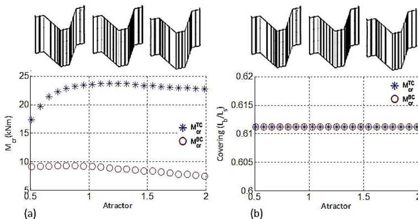
Figura 12: Tendências resultantes de diferentes distribuições de enrijecedores na alma, com base no parâmetro “atrator”: (a) momentos críticos associados à compressão da mesa superior e inferior e (b) taxa de cobertura
