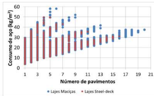
Figura 34 - Relação entre vão da laje e número de pavimentos da torre e o consumo para aço AR345. (Fonte: elaborada pelos autores)
