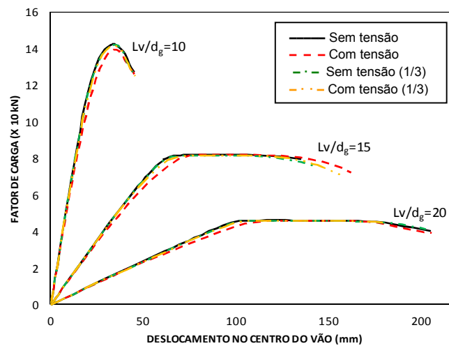
Figura 20 - Curvas de resistência para o perfil W 410x60,0, padrão Litzka.
