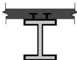
Figura 5 – Ligação mesa-laje por meio de conectores. (Fonte: adaptado de Pfeil [11]).
