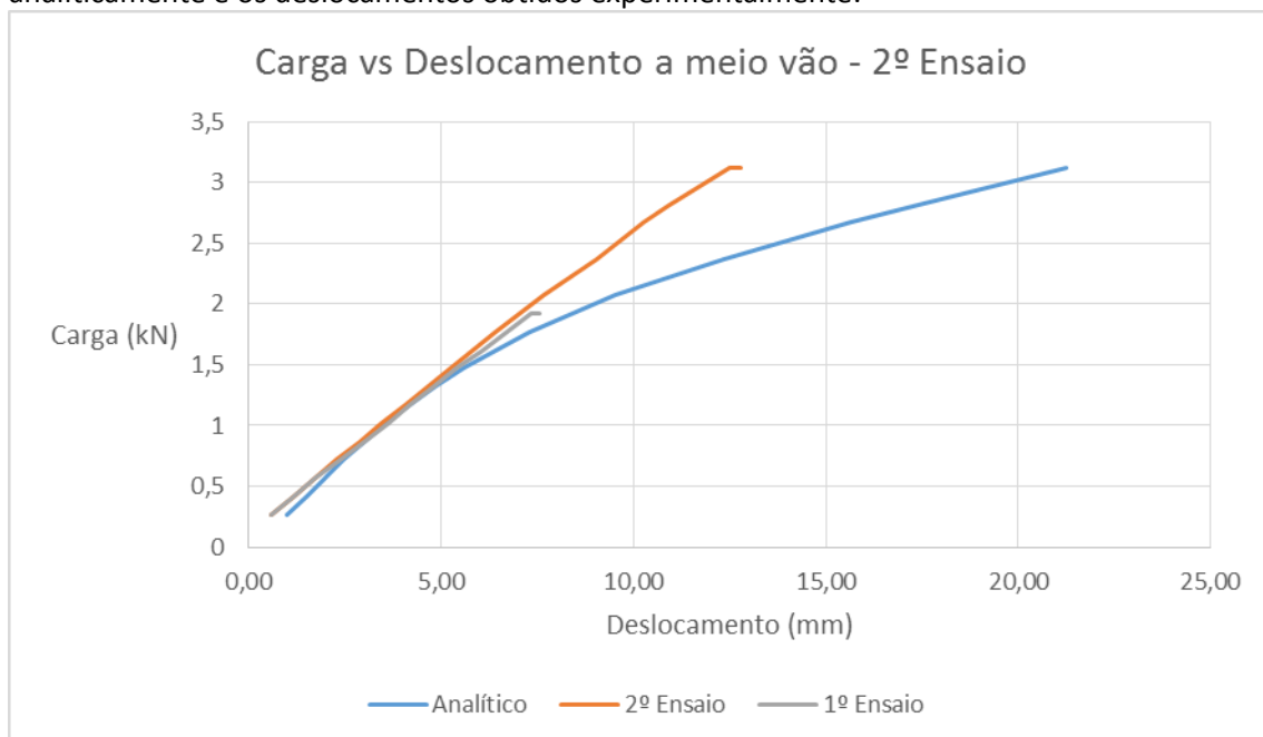
Figura 11 – Comparação dos deslocamentos obtidos analiticamente com os obtidos experimentalmente.
