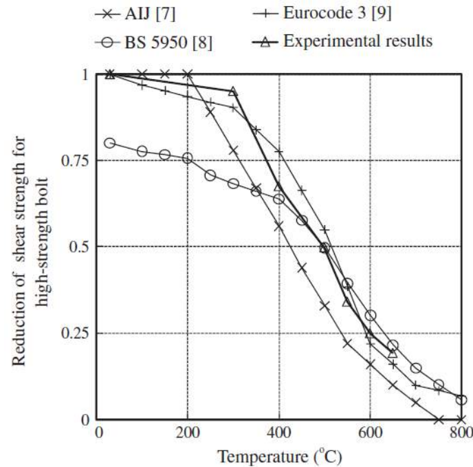
Figura 3 - Redução da resistência ao cisalhamento de parafusos de alta resistência com a temperatura. (Eixo x: Temperatura (°C), Eixo y: Redução da resistência ao cisalhamento de parafusos de alta resistência). Fonte: Yang et al. (2011).
