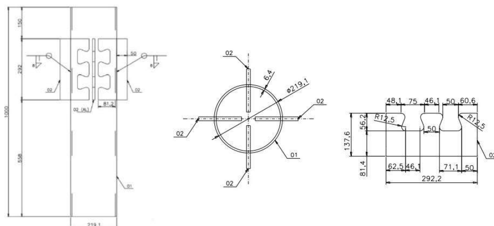
Figura 13: Geometria do Pilar misto com o uso do Conector Crestbond
