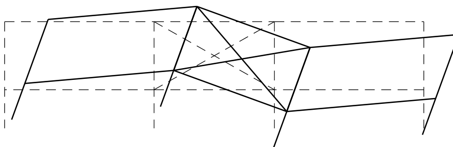
Figura 3. Distorção por cisalhamento dos painéis de um pavimento contraventado.
