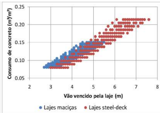
Figura 8 - Taxa de concreto em relação ao vão. (Fonte: elaborada pelos autores)
