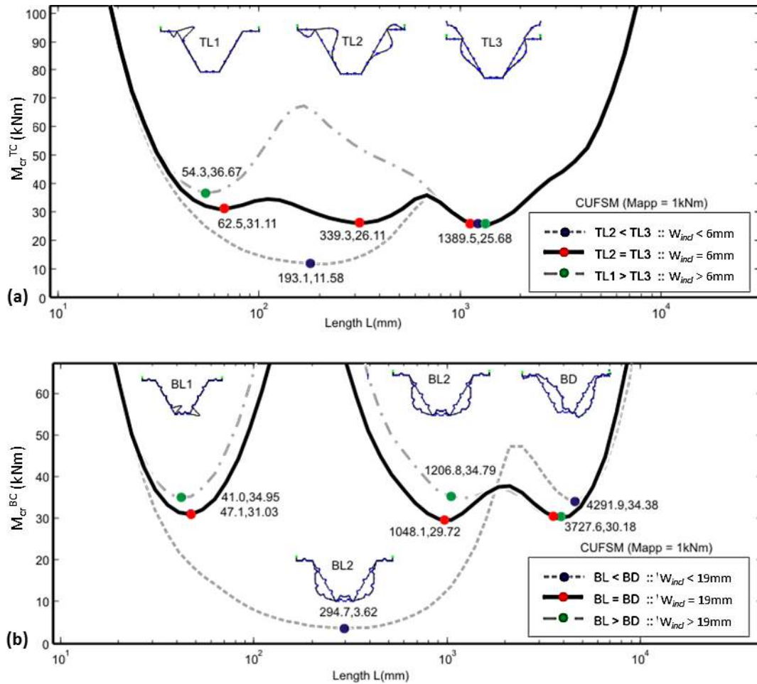
Figura 14: Curvas de “assinatura” obtidas por análise de estabilidade através do Método das Faixas Finitas: (a) momento fletor crítico associado à compressão da mesa superior em função da dimensão w_{incl3} , (a) momento fletor crítico associado à compressão da mesa inferior em função da dimensão w_{incl3} .
