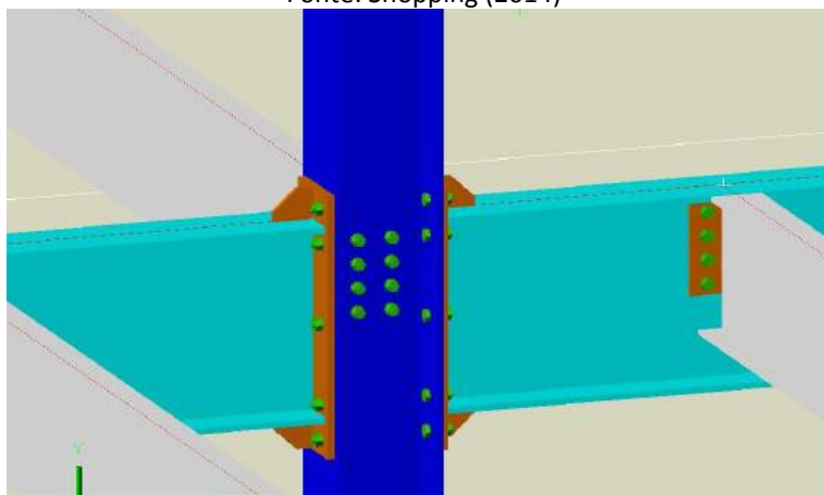
Figura 10 – Ligações: parafusos A325, 19mm Fonte: Shopping (2014)
