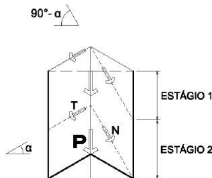
Figura 9 – Estágios de pressão nas paredes, definidos pela componente N
