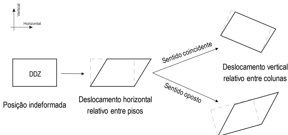
Figura 2. Distorção por cisalhamento de um painel (DDZ).
