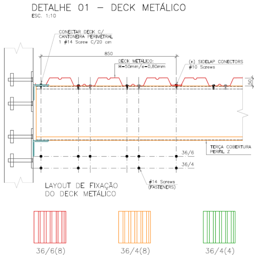
Figura 18 – Detalhe do deck, bem como as configurações de conectores referentes a cada região, representadas pelas cores vermelho, laranja e verde.
