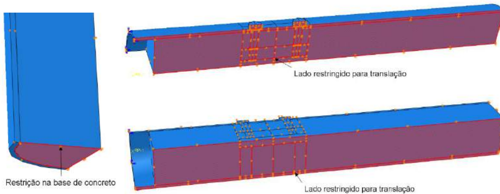
Figura 6 - Restrições aplicadas na modelagem numérica
