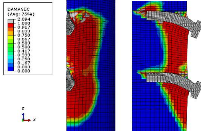
Figura 12 - Dano à compressão no núcleo de concreto
