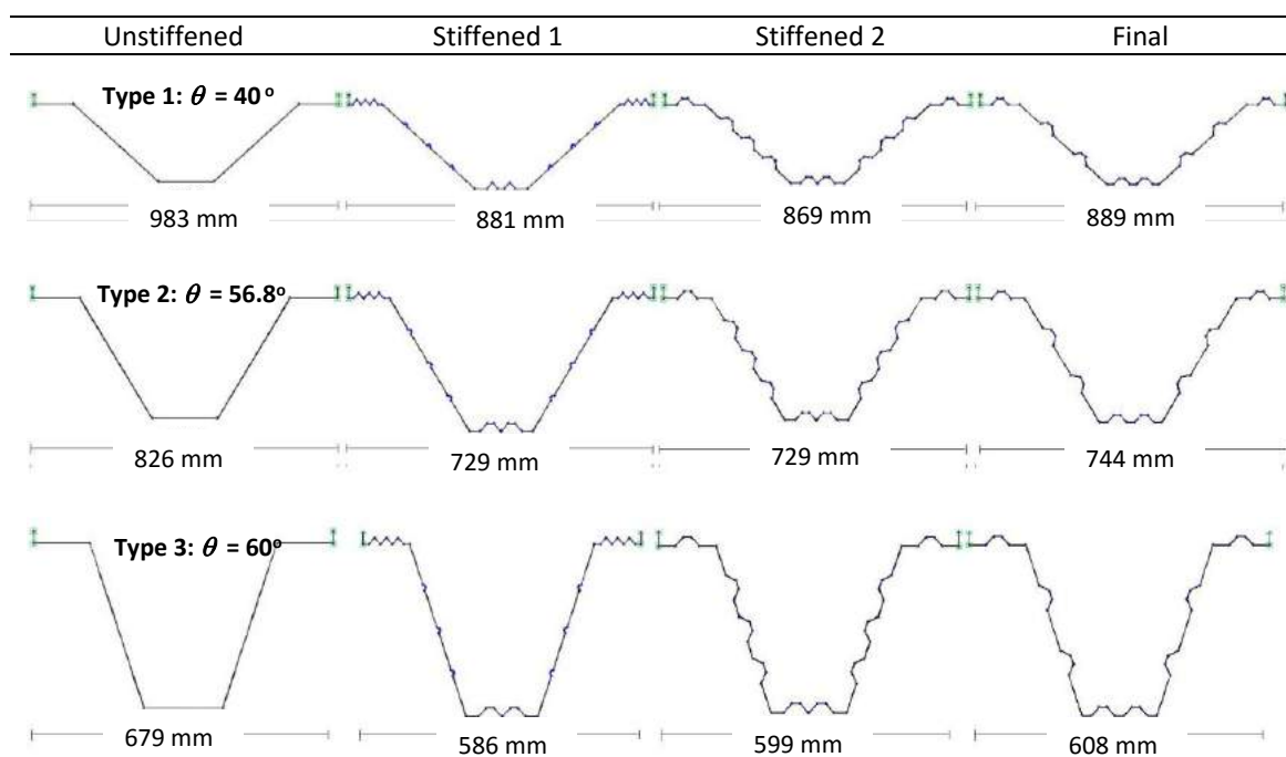
Figura 20: Resultados da evolução de vigas-calha com espessura t=1,0\text{mm} .
