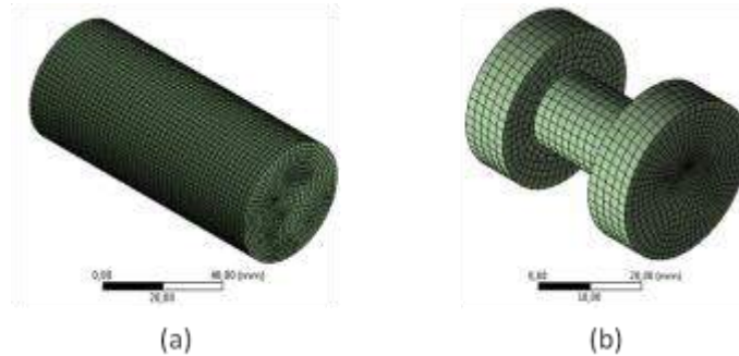
Malha no pino e conjunto do parafuso. (a) Pino; (b) conjuntos de parafusos.
