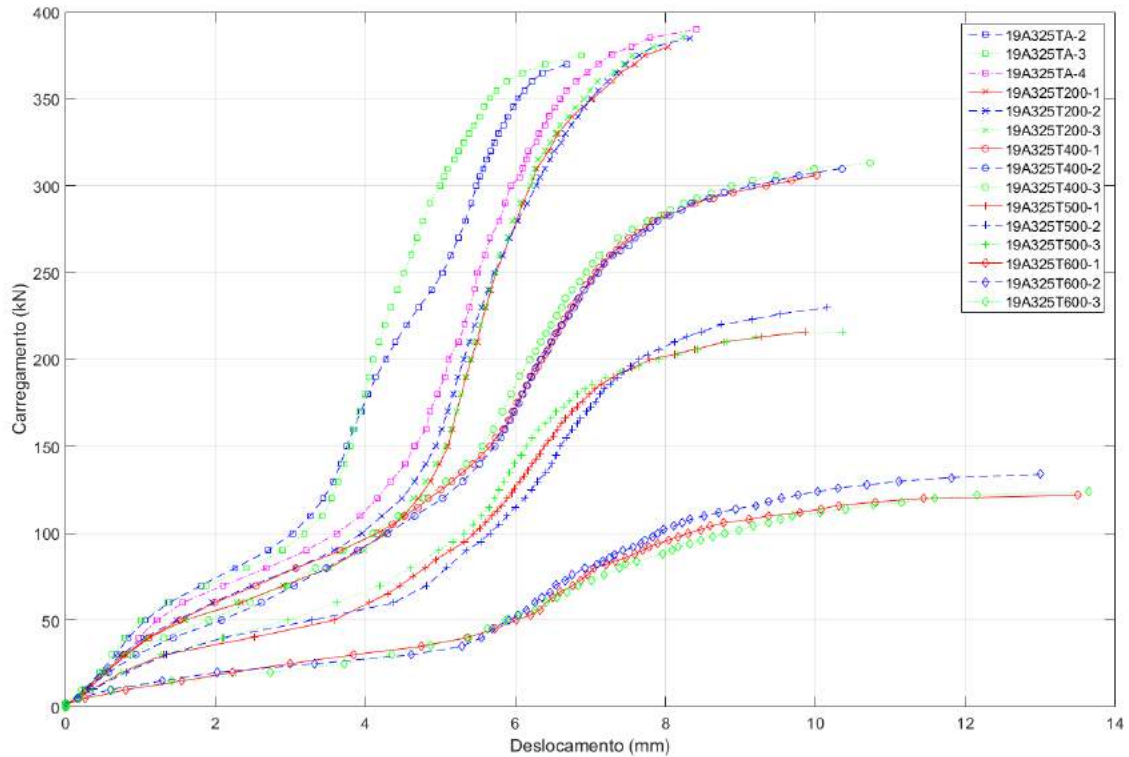
Figura 6 - Gráfico Carregamento x Deslocamento
