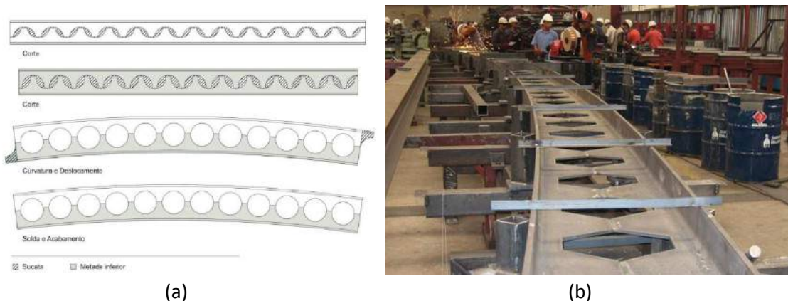
Figura 4 - (a) Esquema de fabricação de uma viga celular com eixo curvo (fonte: Oliveira [4]). (b) Fabricação de uma viga castelada curva (fonte: Steelssalg [5]).
