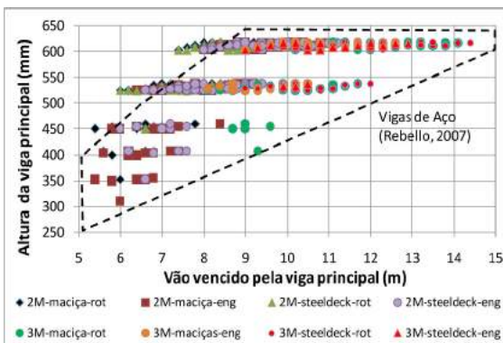
Figura 11 - Relação entre vão e altura da viga principal em aço MR250. (Fonte: elaborada pelos autores)
