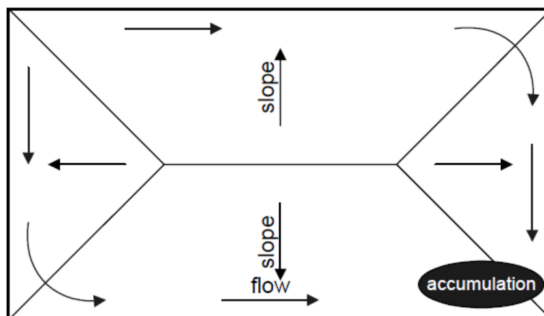
Figura 05 – Potencial ao empoçamento em coberturas com grandes áreas.
