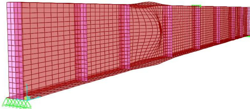
Figura 3: Seções cruciformes
