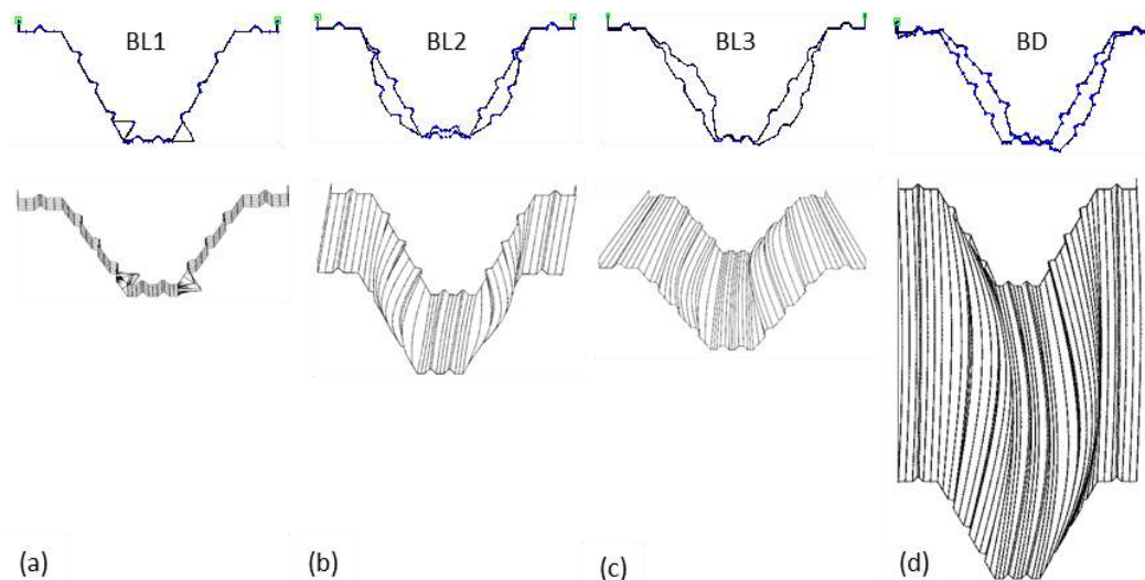
Figura 7: Modos de flambagem elástica para vigas calhas com mesa inferior comprimida: (a-c) modos locais e (d) modo distorcional.
