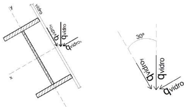
Figura 10 – Carregamento distribuído ao longo da viga (Fonte: Elaborada pelo autor)
