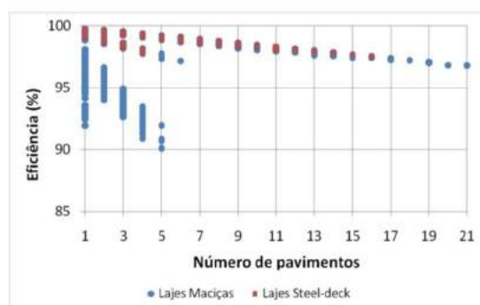
Figura 23 - Eficiência dos pilares de perfis em aço MR250. (Fonte: elaborada pelos autores)
