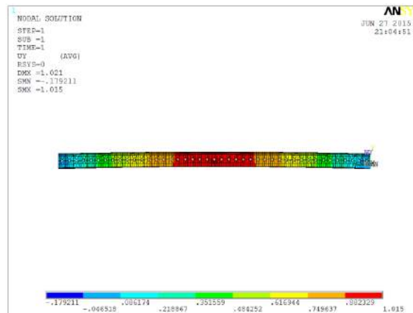
Figura 27 - Deslocamentos verticais – análise linear de 1ª ordem (medidas em cm).
