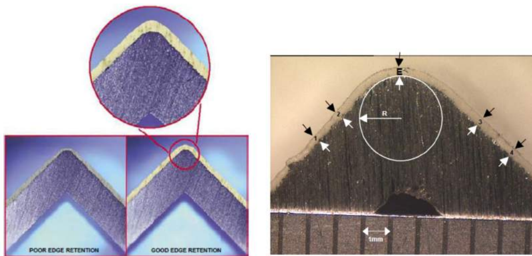
Figura 05: Esquemática do ensaio de retenção de borda
