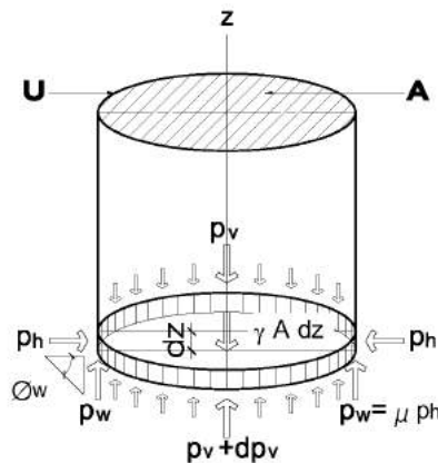
Figura 1 – Modelo matemático de Janssen
