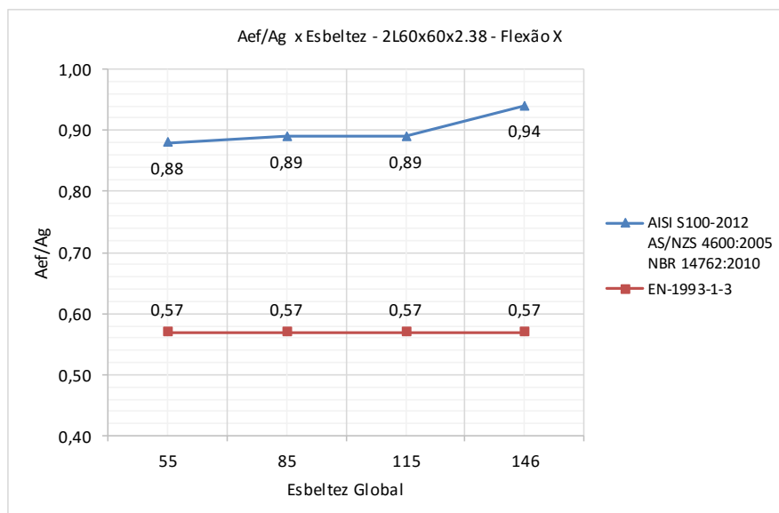
Figura 16 — Resultados analíticos para dupla cantoneira com flexão liberada para eixo X – A_{ef}/A_g x E.G. - MLE
