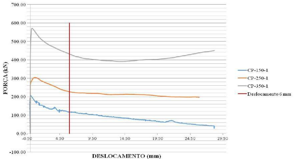
Figura 3 - Força versus deslocamento dos corpos de prova com seção quadrada.
