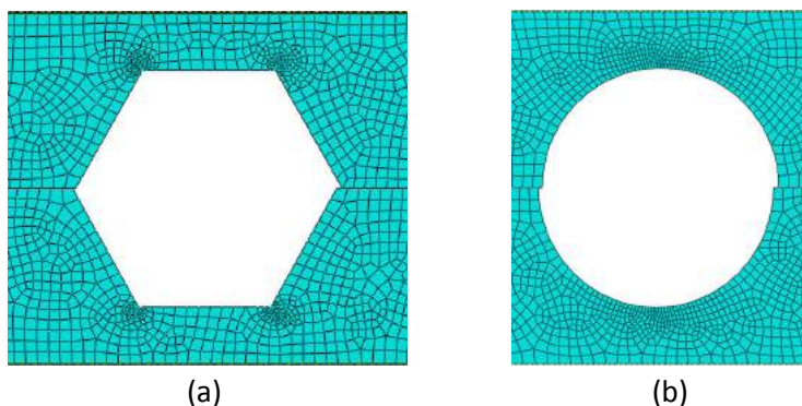
Figura 17 - Refinamento da malha ao redor do alvéolo em vigas (a) casteladas e (b) celulares.
