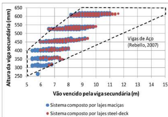
Figura 9 - Relação entre vão e altura da viga secundária em aço MR250. (Fonte: elaborada pelos autores)
