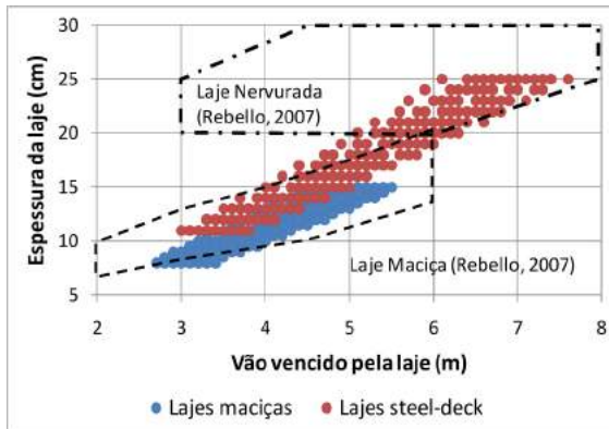
Figura 7 - Relação entre vão e espessura da laje. (Fonte: elaborada pelos autores)
