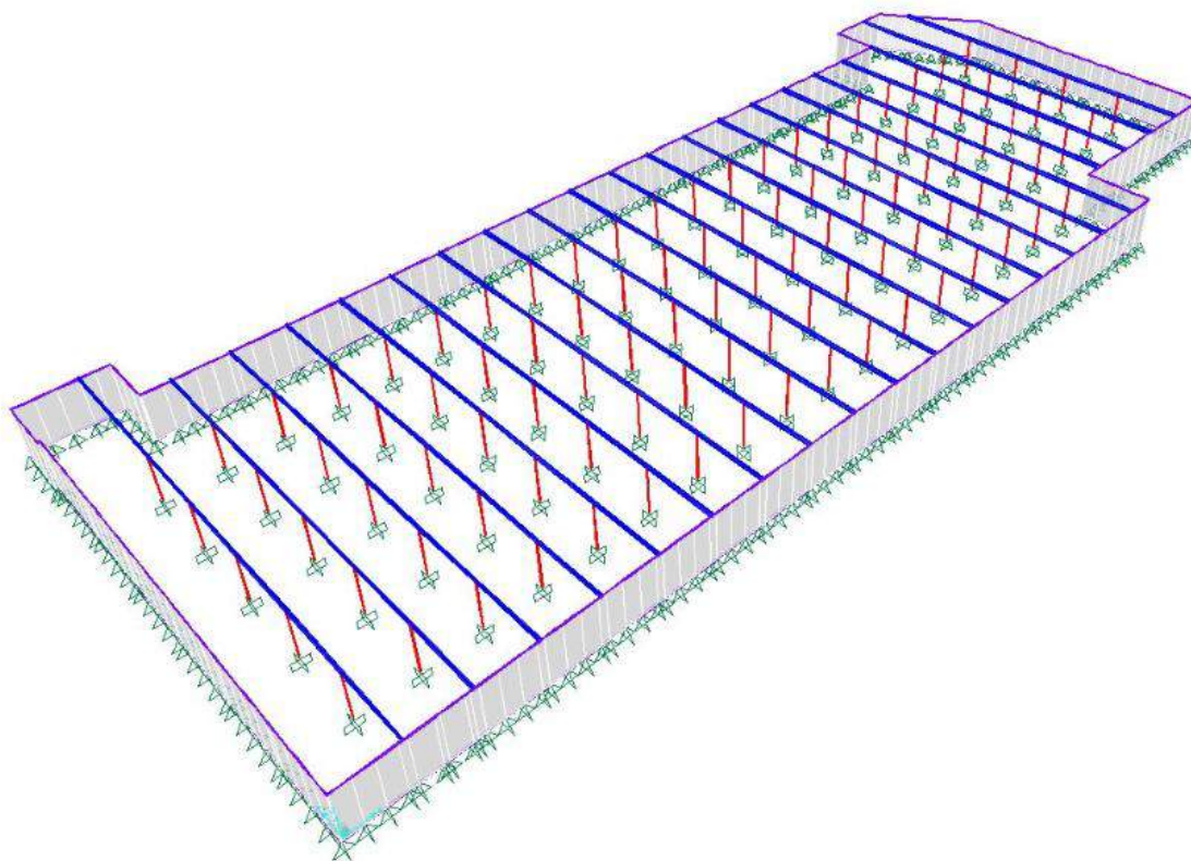
Figura 11 – Vista tridimensional mostrando o sistema estrutural avaliado no estudo de caso, comum ao sistema convencional e “roof deck”.
