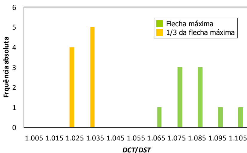
Figura 26 - Relações entre deslocamentos no centro do vão para modelos com tensão (DCT) e sem tensão (DST) para padrão celular.
