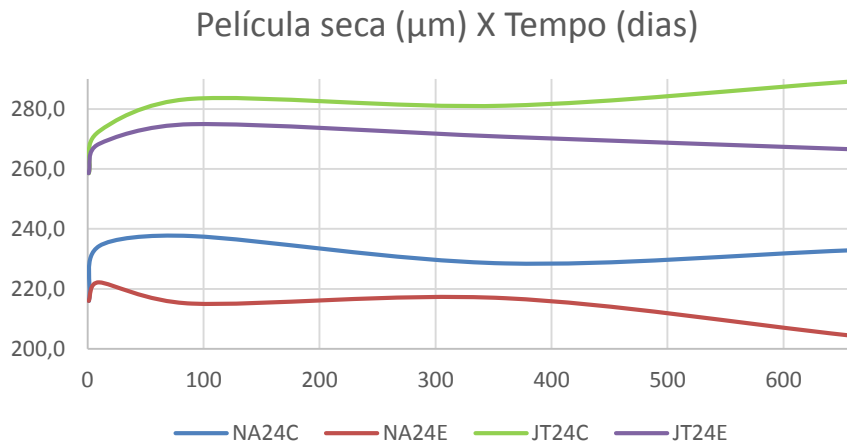
Figura 42: Comparativo gráfico entre corpos de prova com a mesma camada de película seca (240 \mu\text{m} )
