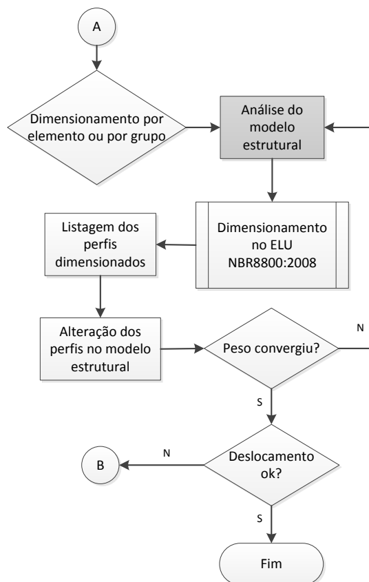
Figura 6 – Fluxograma da otimização do peso no ELU.
