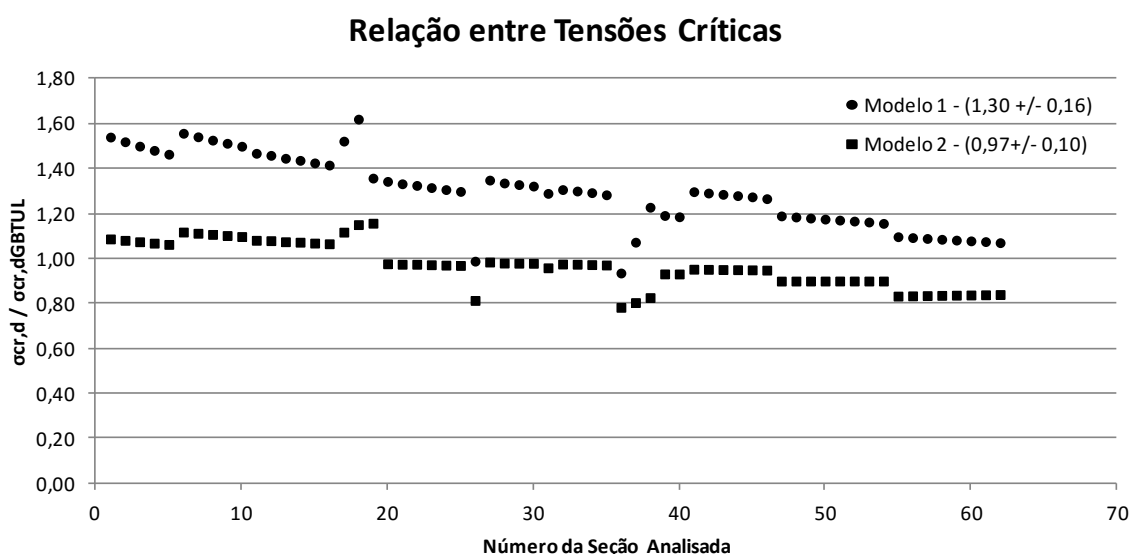
Figura 6: Relação \sigma_{cr,d}/\sigma_{cr,dGBTUL} de cada Modelo de análise para as seções indicadas na tabela 2.
