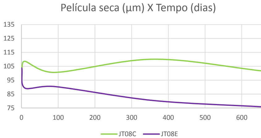
Figura 21: Comparativo gráfico entre corpos JT08 (C) não exposto e (E) exposto
