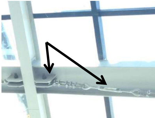
Figura 25 - Detalhe das chapas de extremidade, conector e esticador (Fonte: Arquivo Pessoal)
