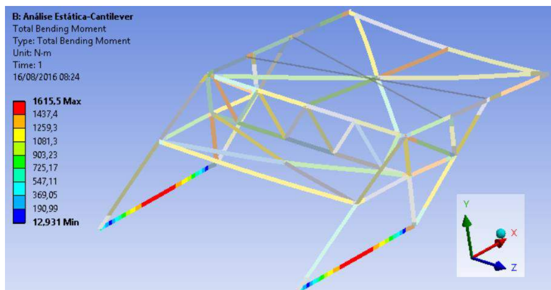
Figura 12 – Momentos fletores atuantes na barra da treliça içadora de aduelas.
