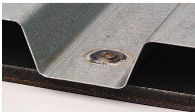
Figura 03 – Conexão “support” efetuada através de solda, denominada solda em poça.
