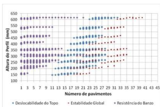
Figura 27 - Relação entre número de pavimentos da torre e perfis em aço MR250 com laje maciça.
