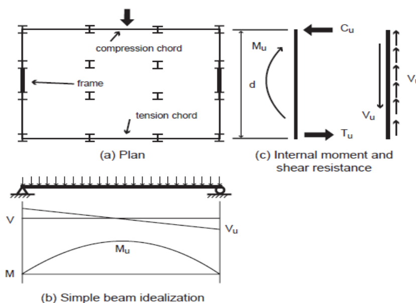
Figura 08 - Análise de diafragma por analogia de viga.
