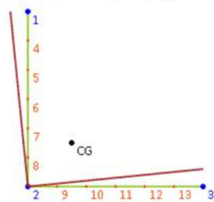
Figura 20 — Resultados para análise numérica via GBTUL para cantoneira L60x60x2.38x1330 — Determinação da carga crítica de flambagem elástica e respectivo modo de falha. Torção 92,21% e Flexão 7,78%.
