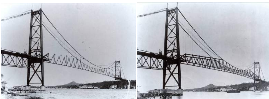
Figura 4: Fechamento dos planos da treliça.
