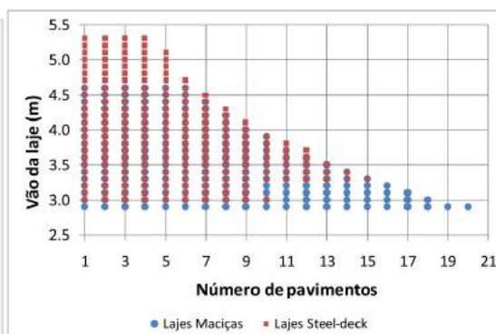
Figura 26 - Relação entre vão da laje e número de pavimentos de pilares em perfis em aço AR345. (Fonte: elaborada pelos autores)
