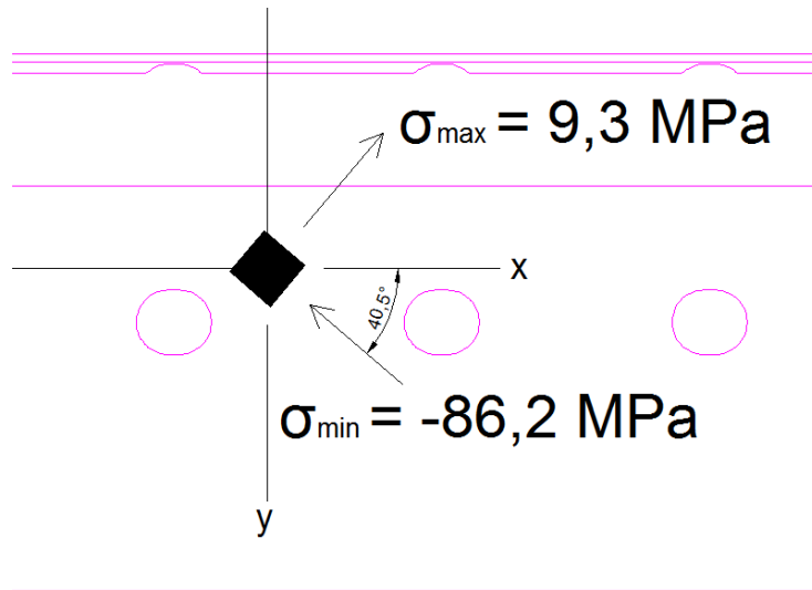
Figura 9 – Direções principais de tensão para o ponto de encontro dos extensômetros colocados em roseta.
