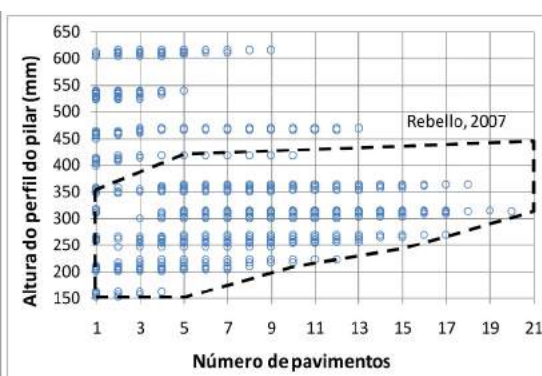
Figura 18 - Relação do número de pavimentos e perfis do pilar em aço AR345 e laje maciça. (Fonte: elaborada pelos autores)
