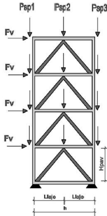
Figura 6 – Torre de contraventamento. (Fonte: adaptado de Pfeil [11]).
