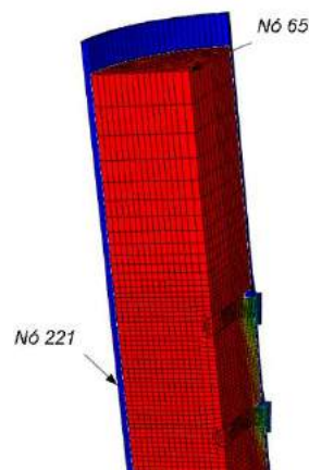
Figura 7 - Localização dos nós referentes aos deslizamento relativo
