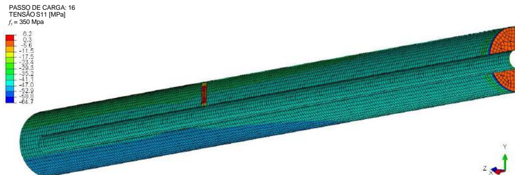
Figura 16 – Modelo com travamentos fixos – Tensões atuantes – Passo de carga 16 ( \lambda_0 = 1,07 e \lambda = 80 )
