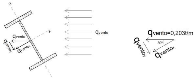
Figura 9 – Decomposição de forças devido ao vento (Fonte: Elaborada pelo autor)
