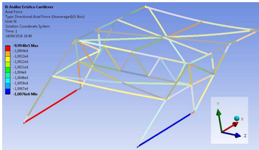
Figura 11 – Força de compressão atuante na barra crítica da treliça içadora de aduelas.
