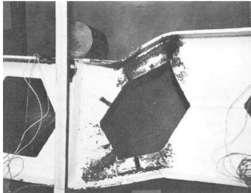
Figura 8 - Formação do mecanismo de Vierendeel (fonte: Hosain e Speirs [9]).
