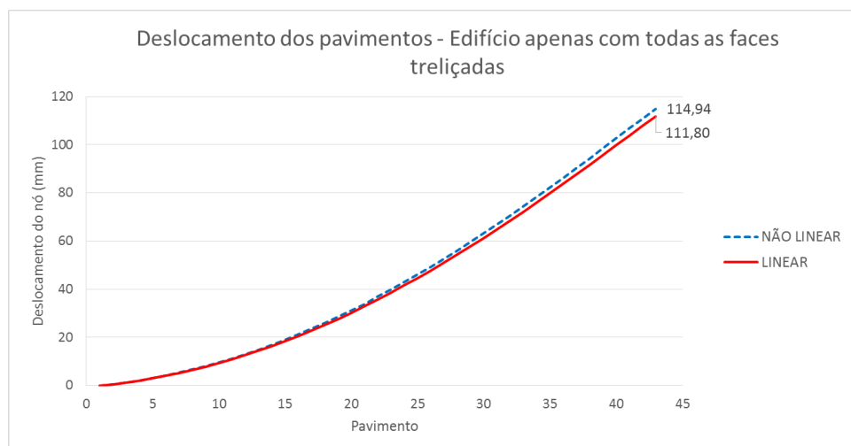
Gráfico 6 – Deslocamentos no edifício com todas as faces treliçadas Fonte: As autoras (2016).
