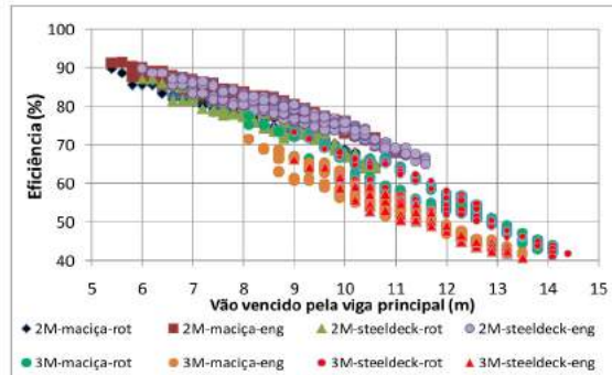
Figura 16 - Eficiência dos perfis das vigas em aço AR345. (Fonte: elaborada pelos autores)
