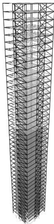
Figura 3 – Vista tridimensional do modelo numérico contraventado com treliças Fonte: As autoras (2016).
