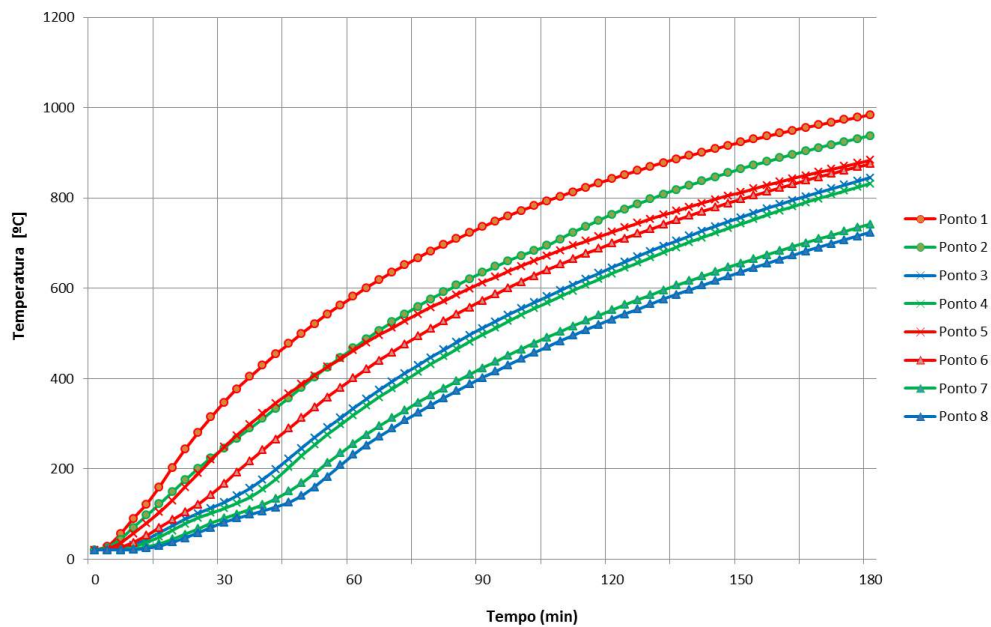
Figura 17: Variação da Temperatura ao longo do Tempo com e sem a Presença do Conector Crestbond
