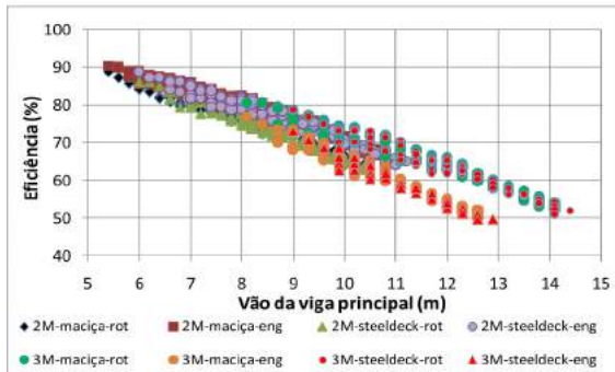
Figura 15 - Eficiência dos perfis das vigas em aço MR250. (Fonte: elaborada pelos autores)
