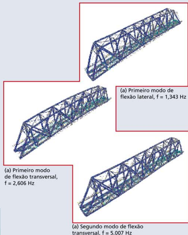
Figura 7 – Parâmetros modais obtidos com modelo numérico
